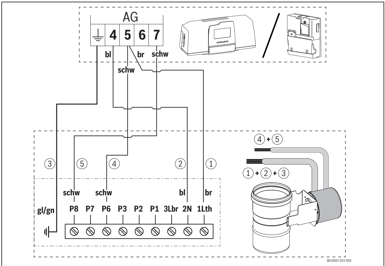
Fig. 34 Schéma de raccordement du clapet des fumées
