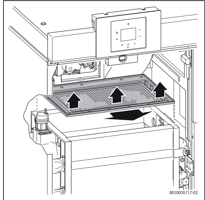
Fig. 43 Démontage du brûleur
