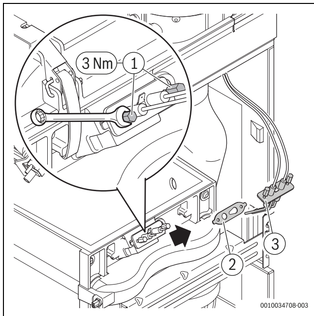
Fig. 48 Insertion de l'allumeur
