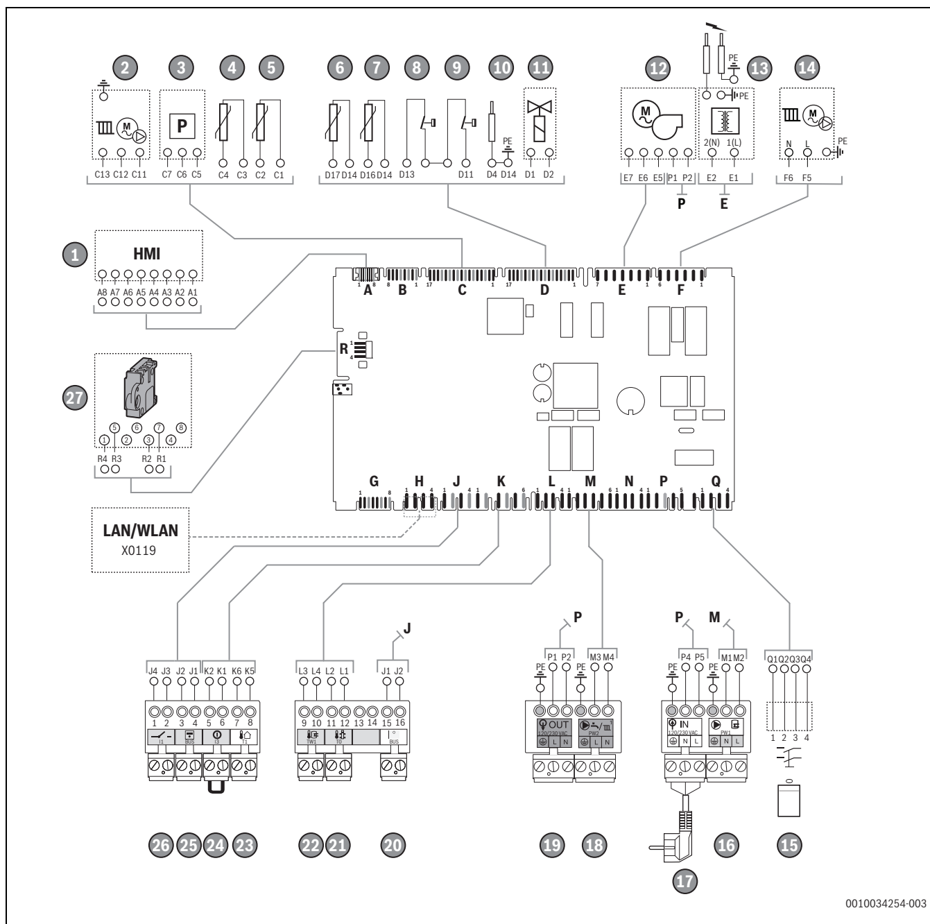
Fig. 51 Schéma de câblage
