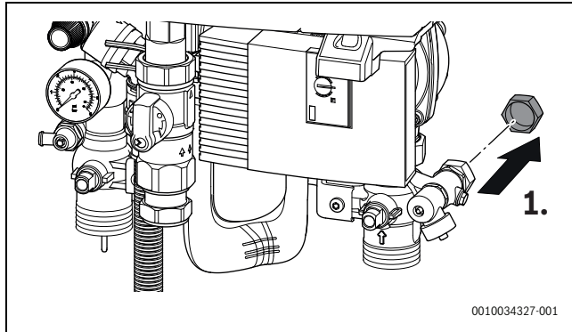
Fig. 20 Raccorder un vase d'expansion
