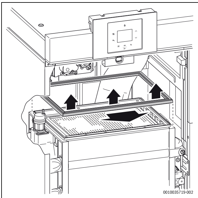
Fig. 42 Démontage du joint du brûleur
