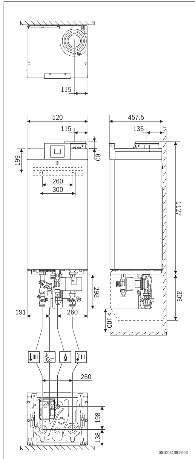
Fig. 3 Dimensions au mur [mm]
