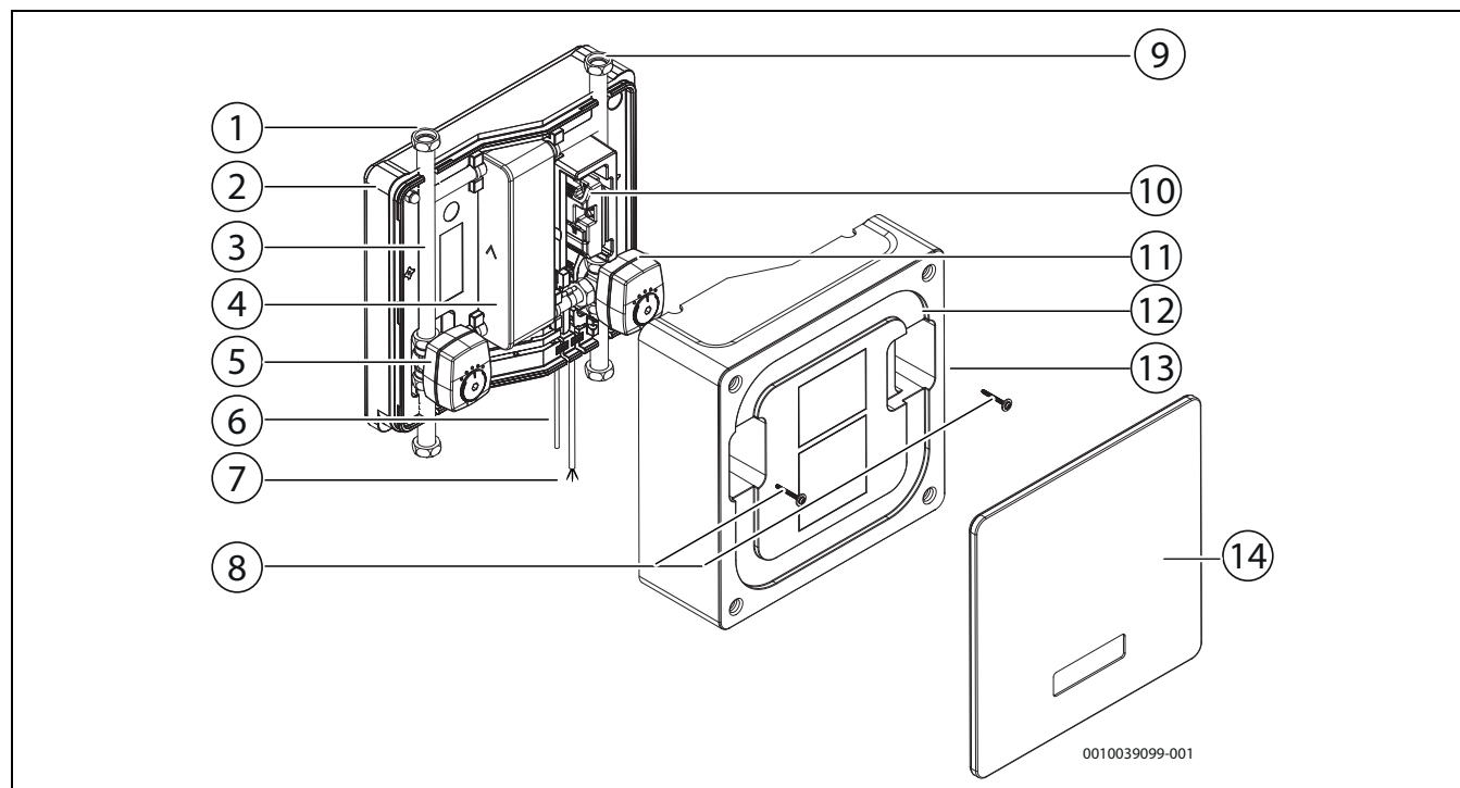
Fig. 2 Panoramica del prodotto
