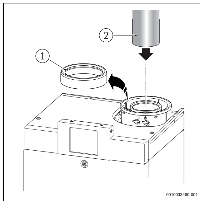
Bild 4 Einzelrohranschluss (raumluftabhängig)
