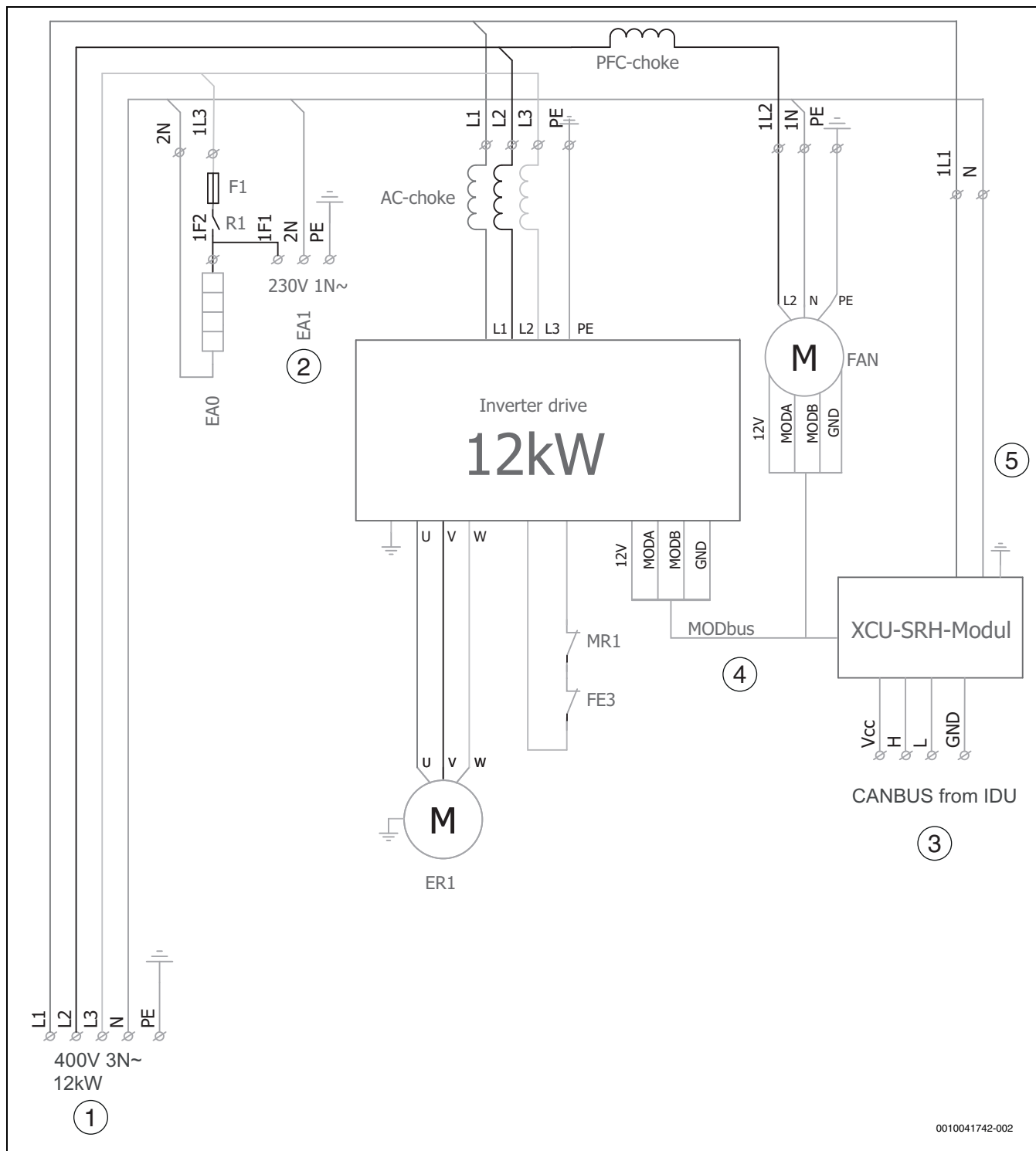
Bild 47 Schaltplan
