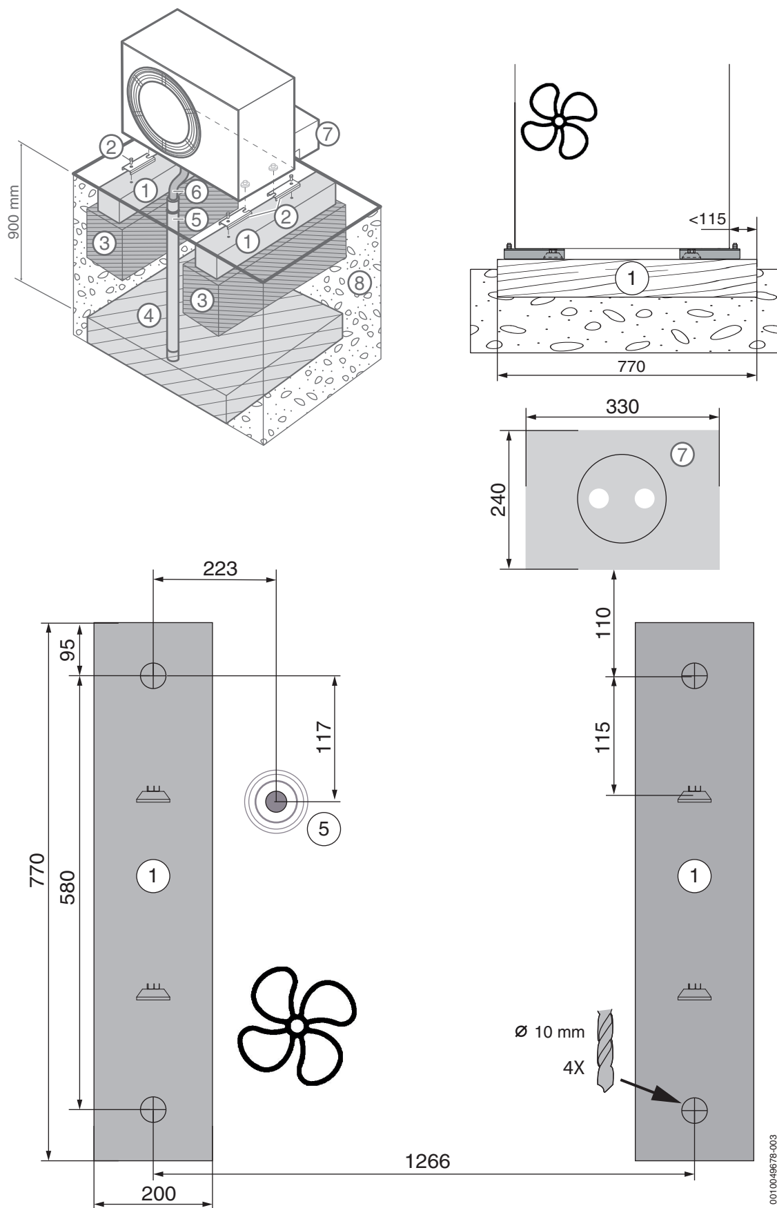
Bild 24 Fundamentplan, Alternative 1
