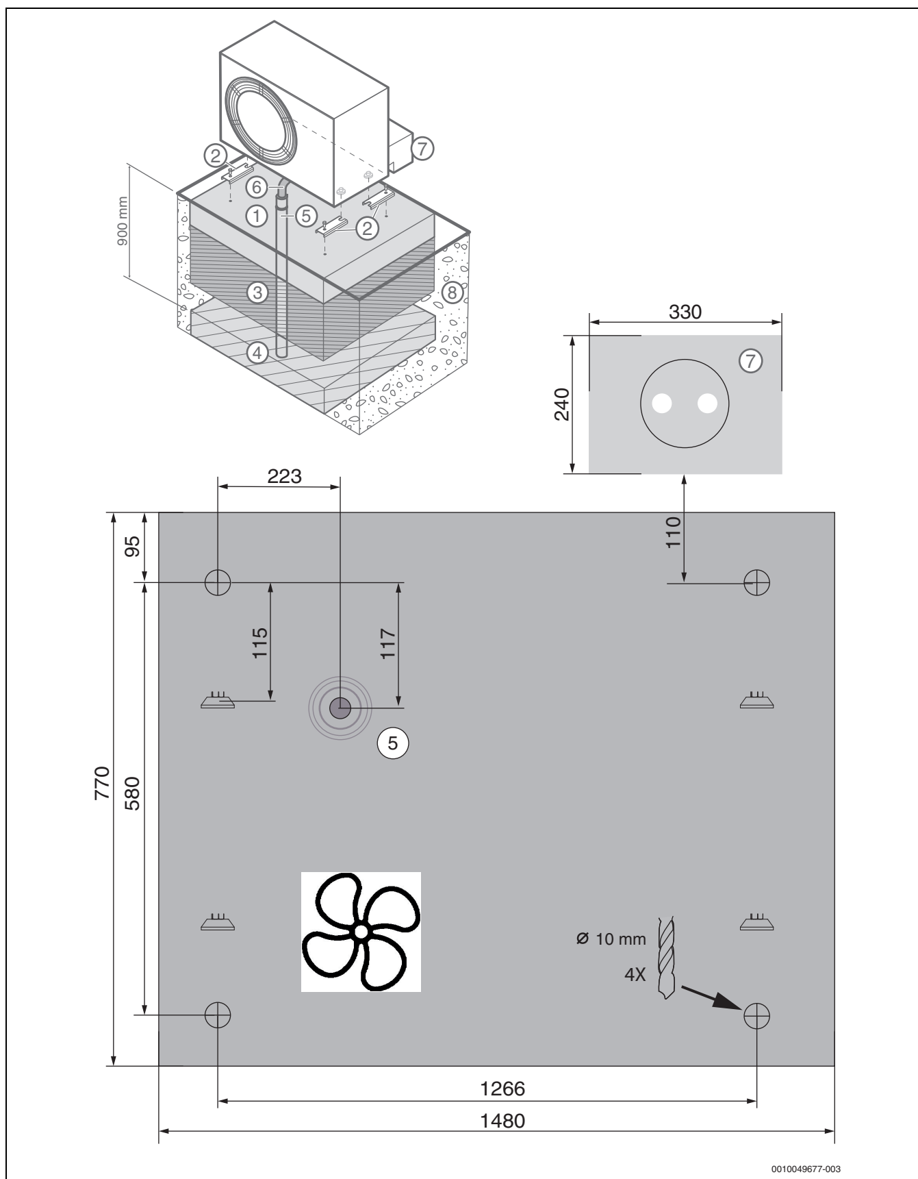
Bild 25 Fundamentplan, Alternative 2
