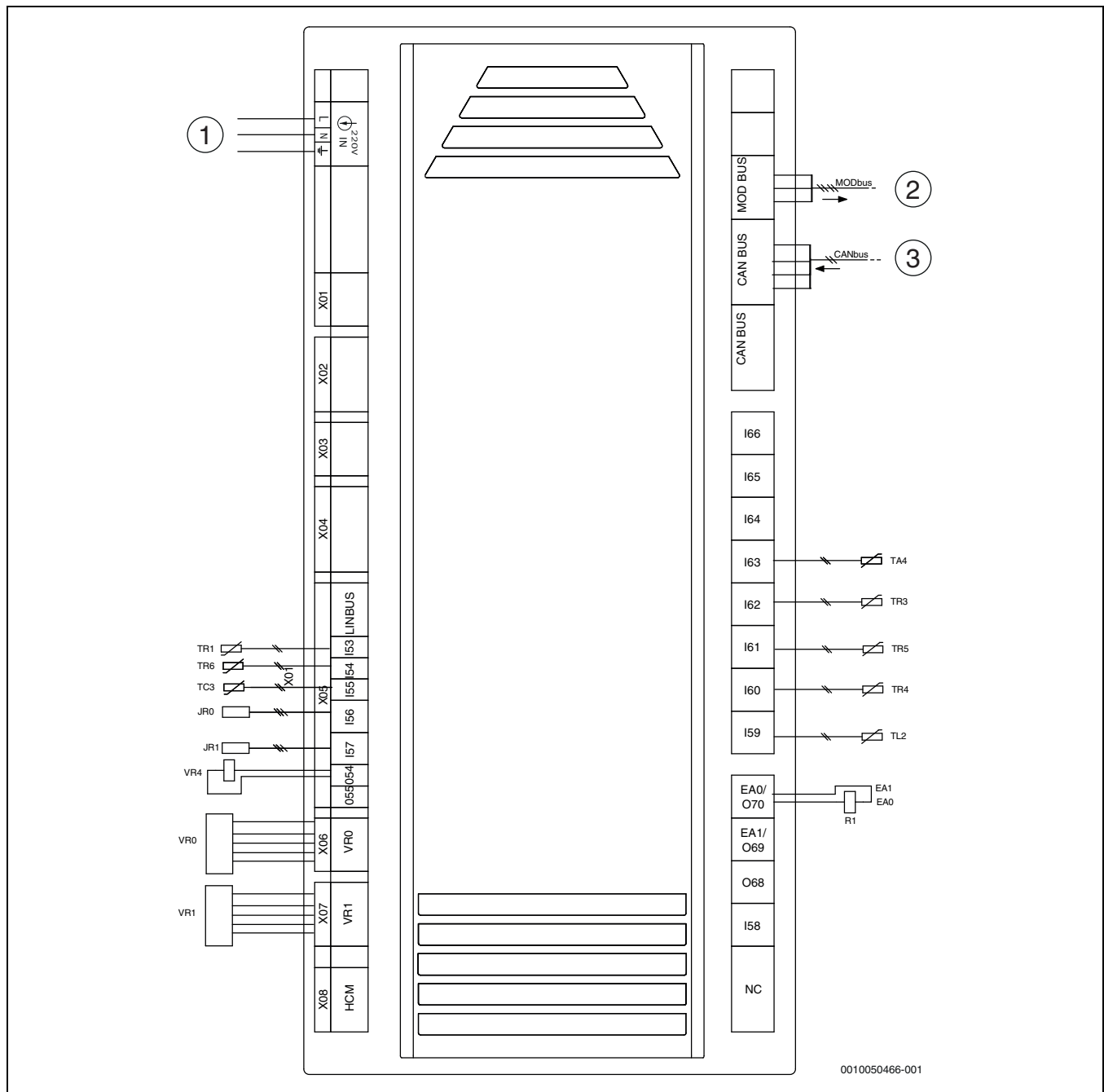
Fig. 50 Schéma de connexion XCU-SRH (XCU-HP)
