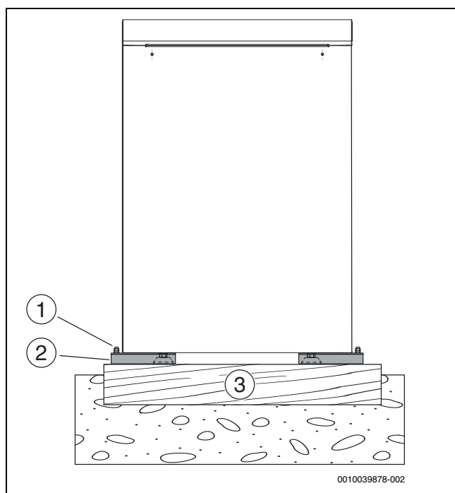
Fig. 20 Fixation de la pompe à chaleur
