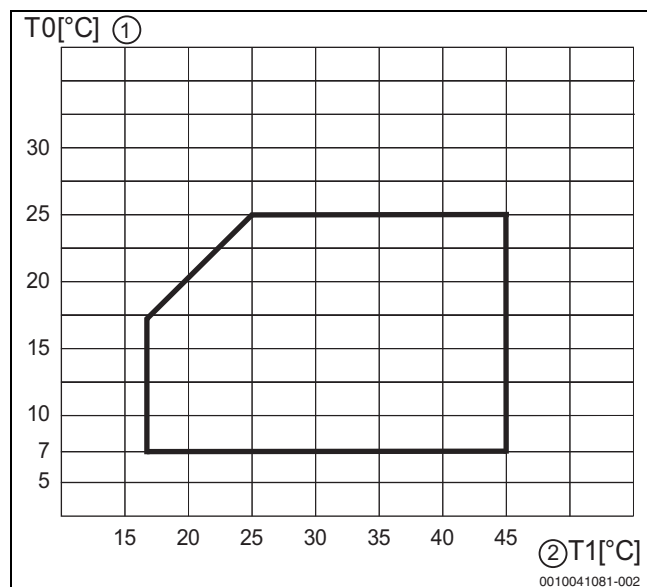
Fig. 47 Pompe à chaleur en mode Refroidissement
