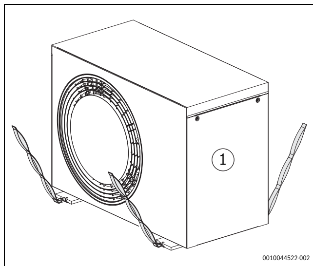
Fig. 11 Utilisation des sangles fournies pour transporter la pompe à chaleur sans son emballage
