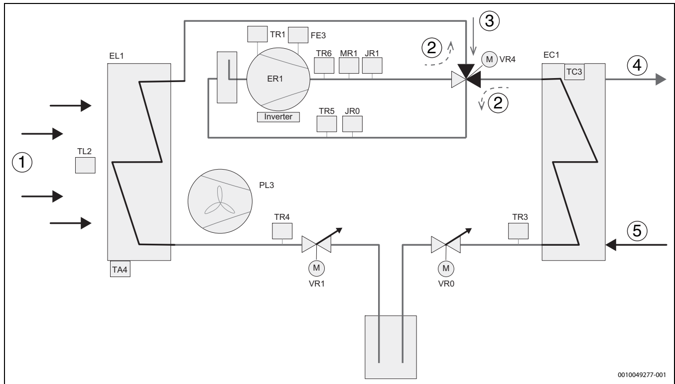
Fig. 48 Circuit de fluide frigorigène
