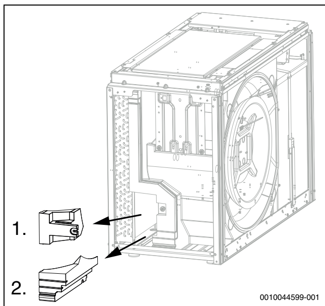
Fig. 41 Pièces en polypropylène expansé
