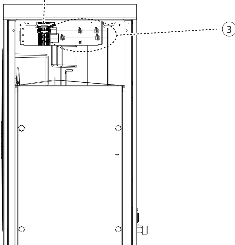
Fig. 37 Bornes de raccordement au niveau de la zone de raccordement de l'installation
