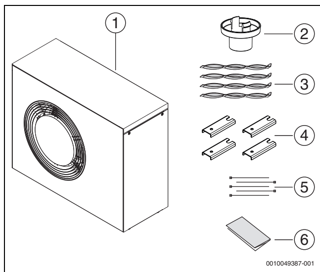
Fig. 1 Pièces fournies
