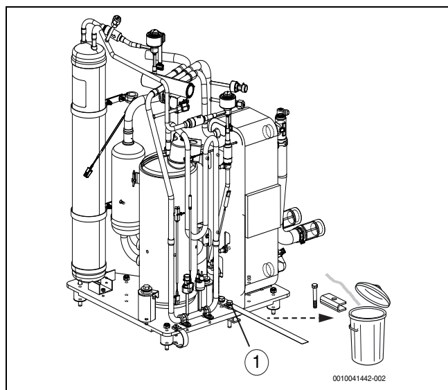
Fig. 33 Sécurisation pour le transport
