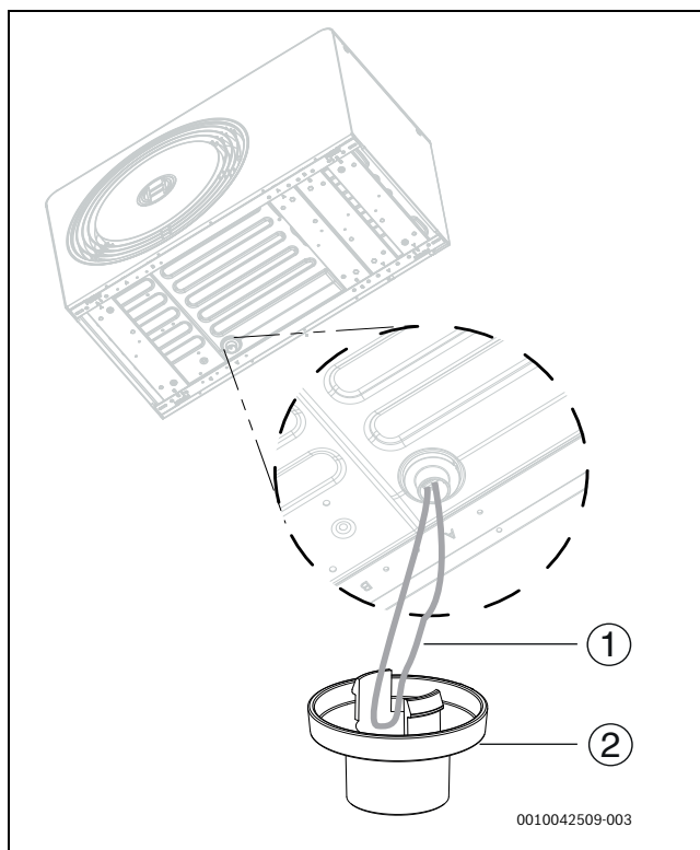
Fig. 27 Installation du raccordement du système d'évacuation
