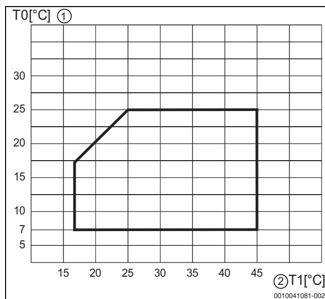
Fig. 45 Pompe à chaleur en mode Refroidissement
