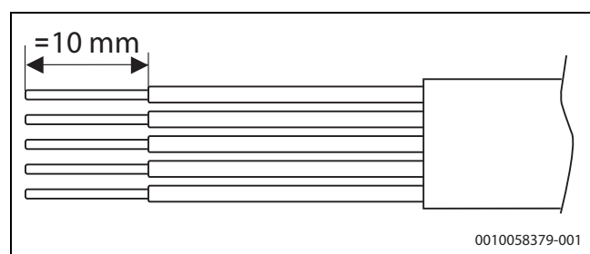
Fig. 38 Dénudage des fils pour le raccordement secteur
