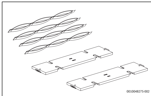
Fig. 12 Parti in legno, staffe metalliche e nastri
