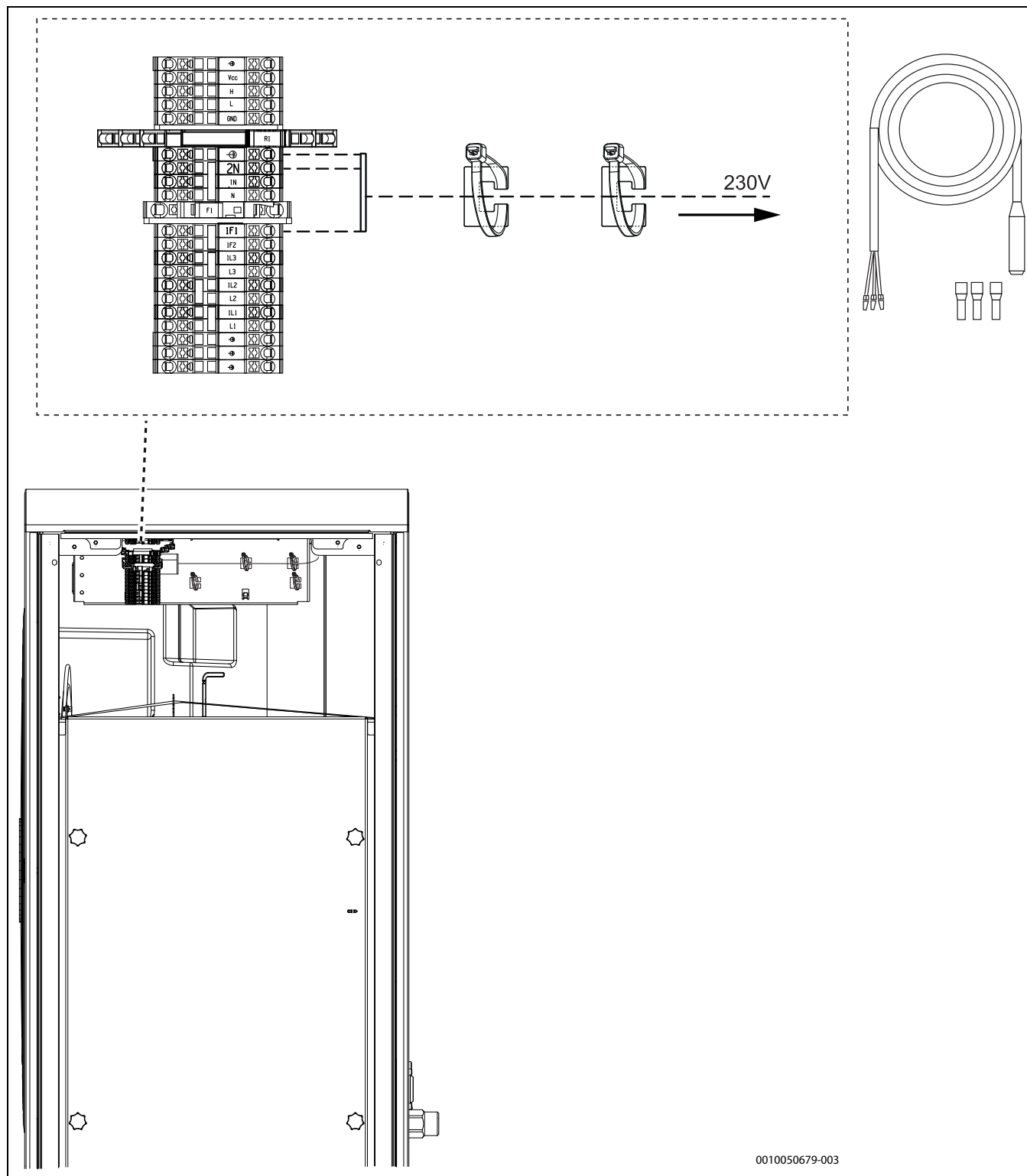
Fig. 39 Collegamento del cavo per riscaldamento (accessorio)
