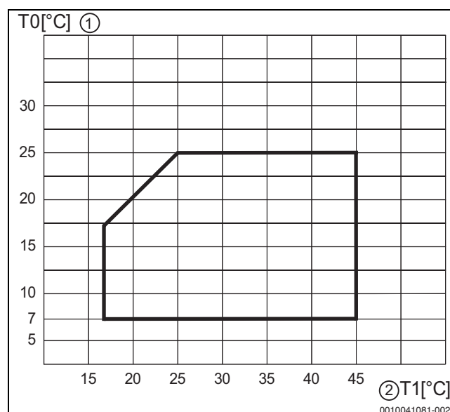
Fig. 45 Pompa di calore in modo raffreddamento
