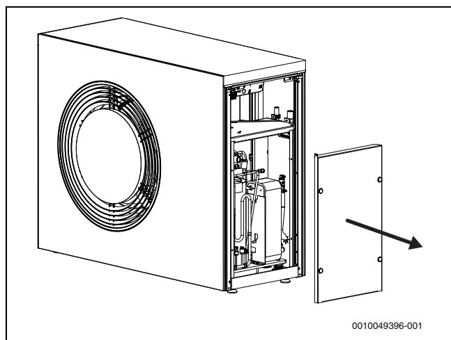
Fig. 32 Coperchio del contenitore del refrigerante
