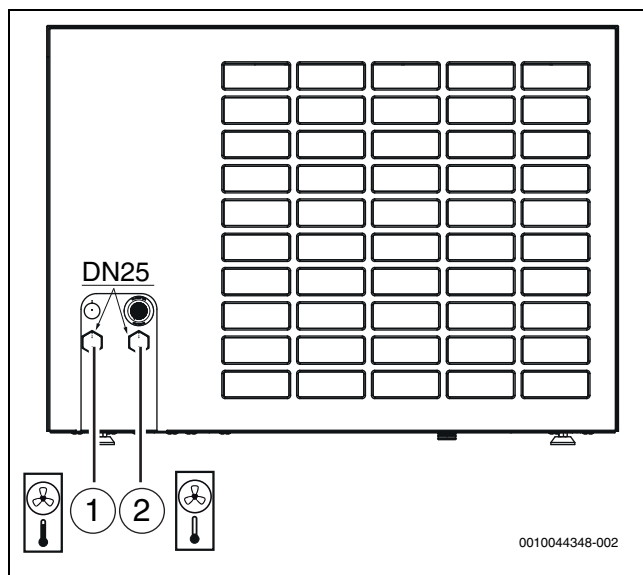
Fig. 30 Collegamenti del tubo del flusso termovettore; la descrizione si applica a tutte le dimensioni
