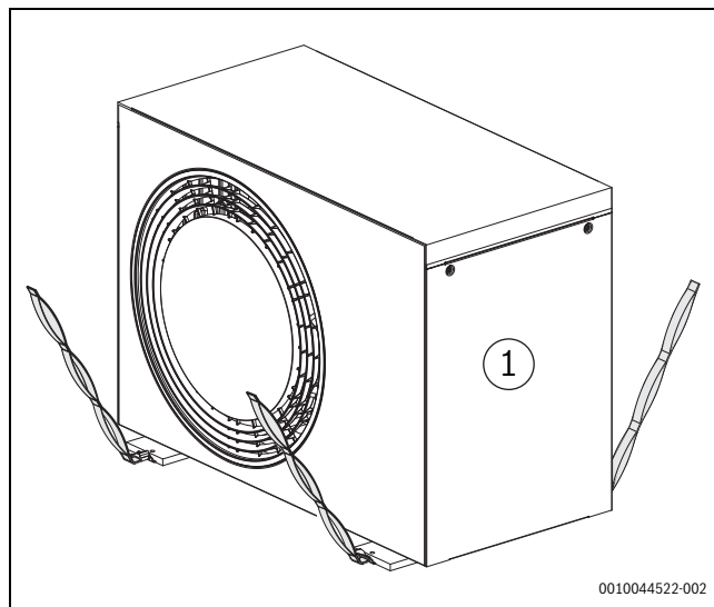
Fig. 11 Utilizzare le fascette per trasportare la pompa di calore senza il suo imballaggio
