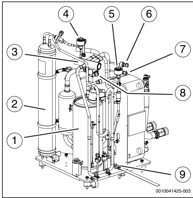
Fig. 2 Panoramica del prodotto - vista anteriore
