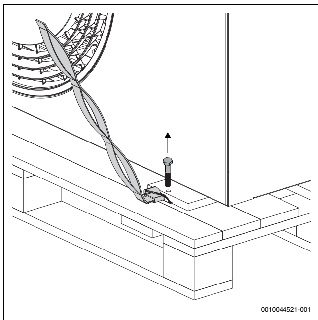
Fig. 10 Applicare le fascette e rimuovere le viti
