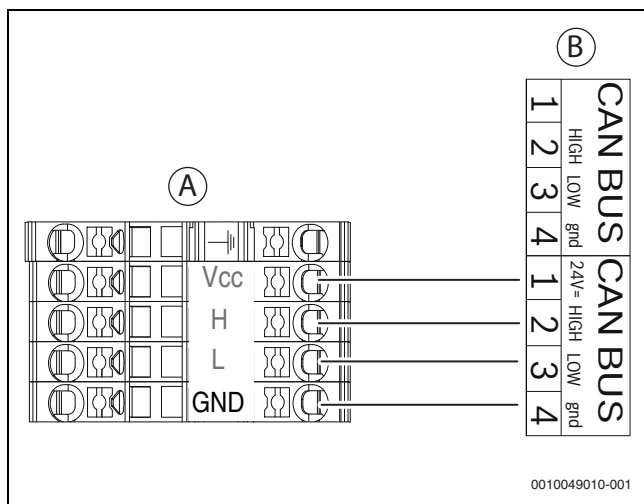
Fig. 34 Pompa di calore CAN-BUS - unità interna
