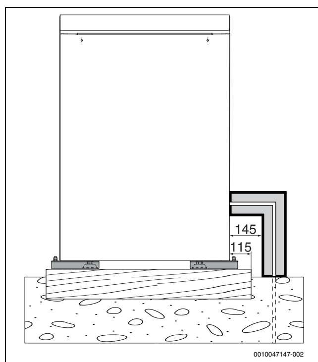
Fig. 23 Vista laterale con set di installazione
