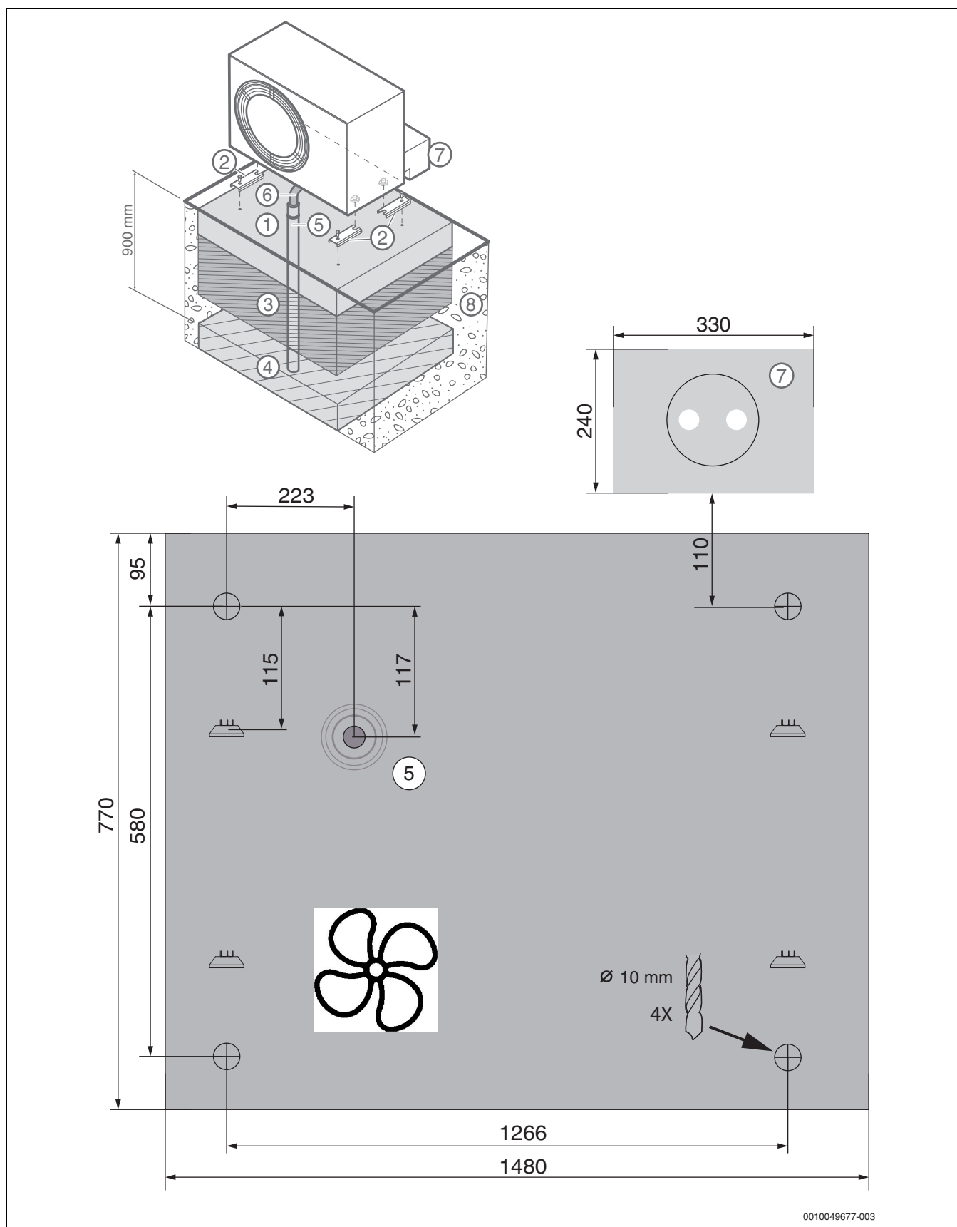
Fig. 25 Schema di fondazione, alternativa 2
