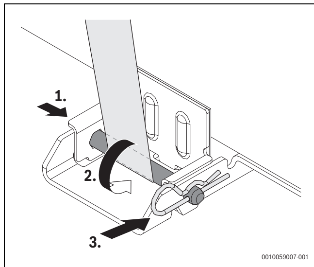
Fig. 13 Inserimento della staffa di bloccaggio, del perno e della cinghia
