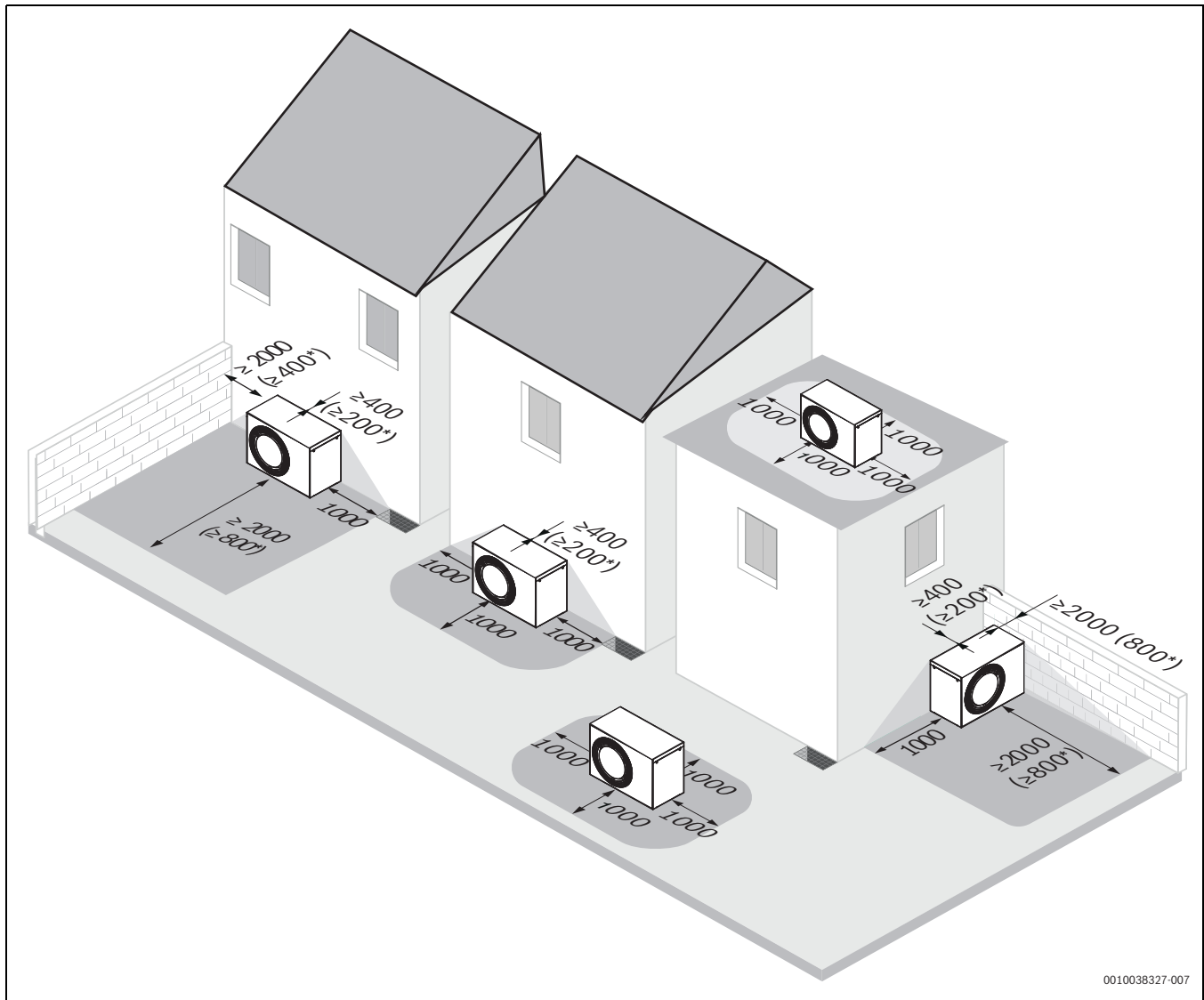
Fig. 18 Spazio raccomandato tra la pompa di calore e i corpi fissi circostanti (mm)
