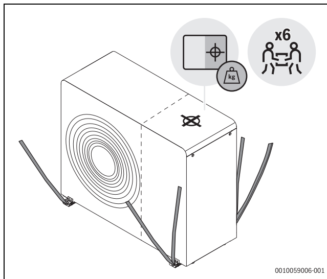
Fig. 14 Utilizzare le fascette per trasportare la pompa di calore senza il suo imballaggio
