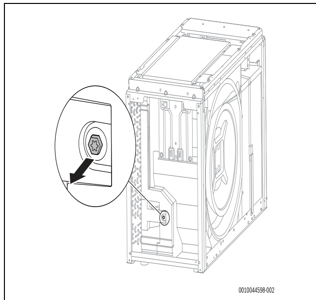
Fig. 40 Svitare
