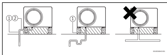
Fig. 29 Scarico della condensa nella rete fognaria/scarico della pioggia
