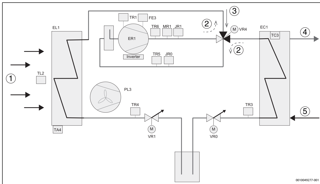
Fig. 46 Circuito refrigerante
