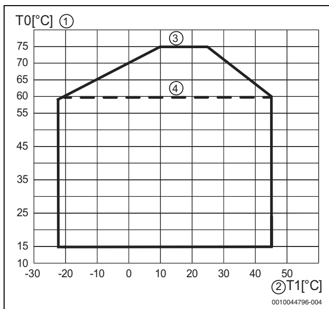
Fig. 44 Pompa di calore in modo riscaldamento senza generatore di calore supplementare
