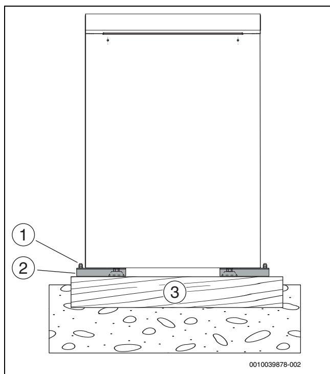
Fig. 20 Fissaggio della pompa di calore
