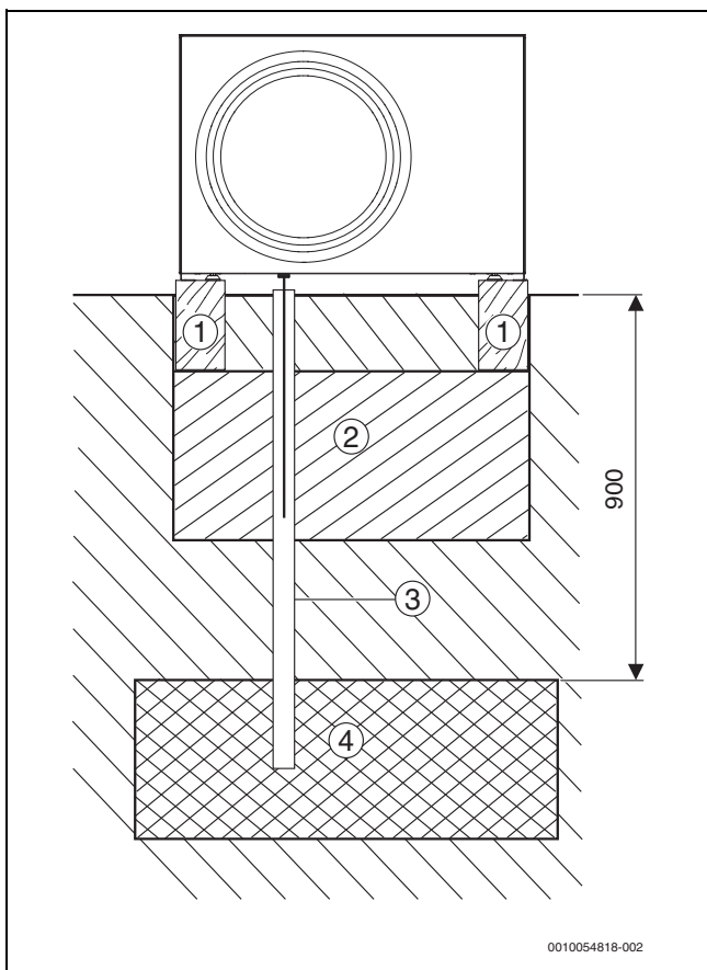
Fig. 28 Scarico della condensa nel letto di ghiaia (dimensioni in mm)
