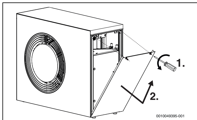
Fig. 31 Pannello protettivo laterale
