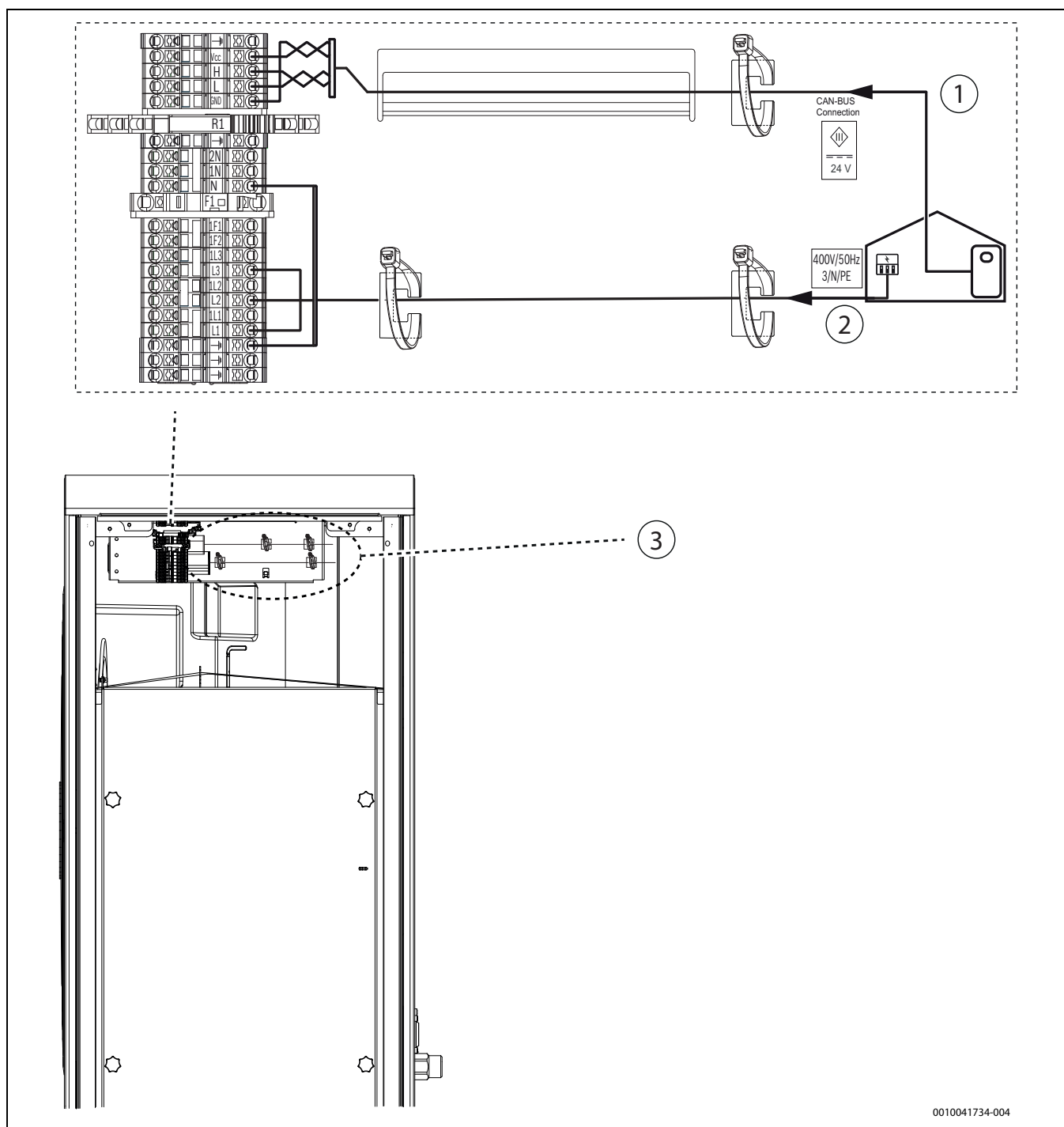
Fig. 37 Terminali nell'area di collegamento dell'installazione
