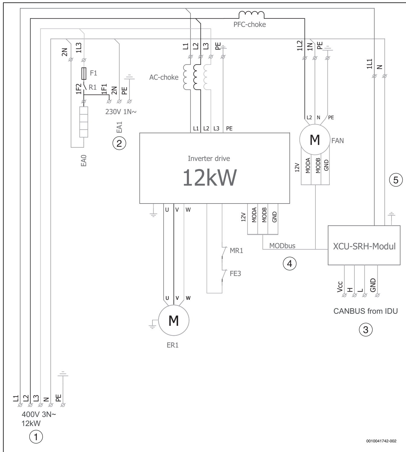
Fig. 47 Schema elettrico inverter
