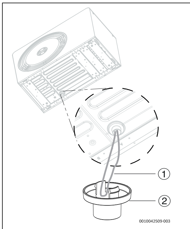
Fig. 27 Installazione del raccordo di drenaggio
