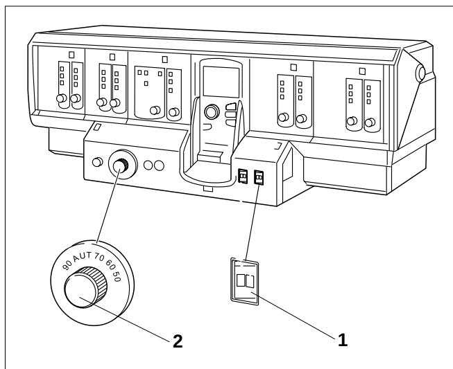
Fig. 1 Apparecchio di regolazione, ad esempio Logamatic 4311
