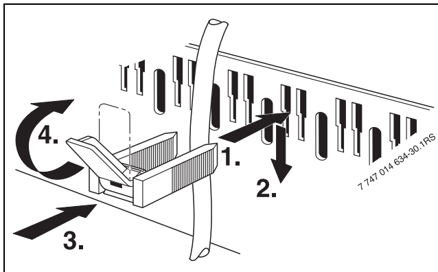
Fig. 4 Passaggio cavi e fermo antitrazione
