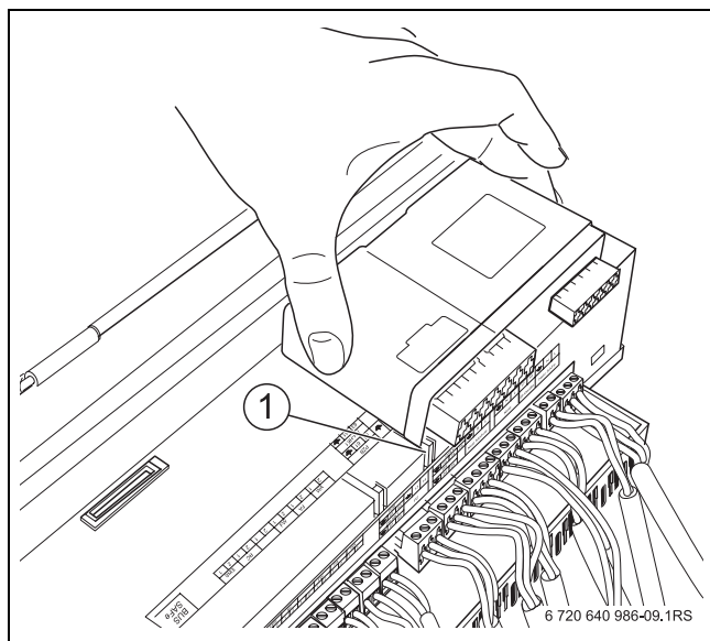
Fig. 5 Inserimento del modulo funzione
