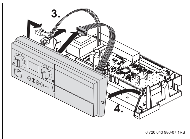
Fig. 9 Smontaggio del dispositivo di controllo base
