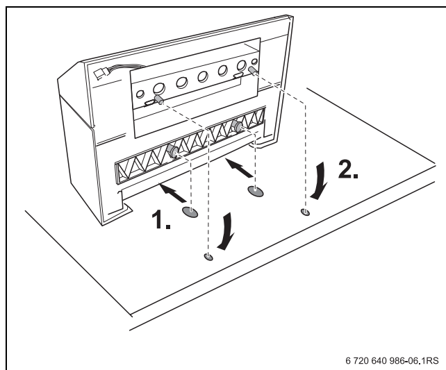
Fig. 3 Montaggio dell'apparecchio di regolazione sulla caldaia (immagine: lato posteriore caldaia)
