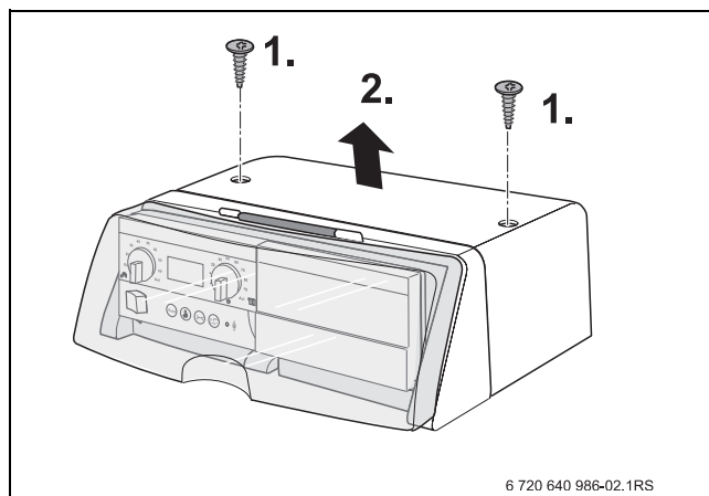
Fig. 2 Rimozione del pannello di copertura
