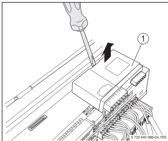
Fig. 10 Rimozione di un modulo funzione
