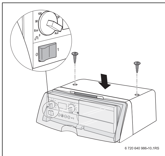
Fig. 6 Montaggio del pannello di copertura
