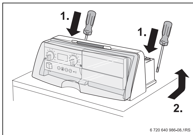
Fig. 11 Smontaggio dell'apparecchio di regolazione dalla caldaia
