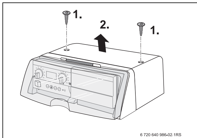
Fig. 8 Rimozione del pannello di copertura
