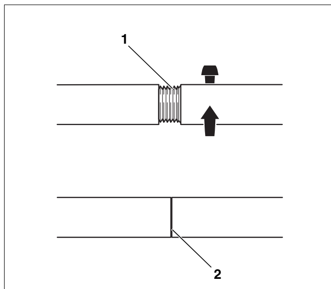
Fig. 16 Strettoi di montaggio 2.3
