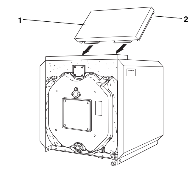
Fig. 37 Montaggio – Copertura posteriore
