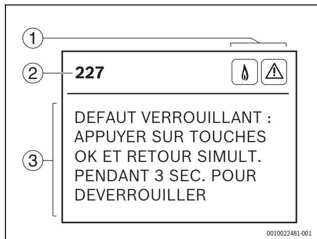
Fig. 13 Menu de défauts (exemple)
