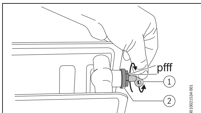
Fig. 12 Purger les radiateurs
