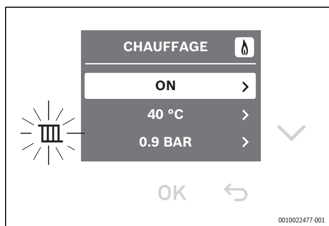
Fig. 10 Menu température chaudière
