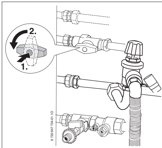
Fig. 4 Ouvrir le robinet de gaz
