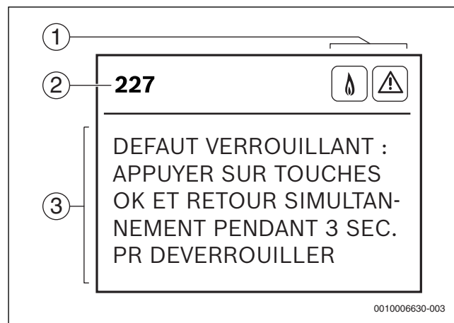
Fig. 5 Menu de défauts
