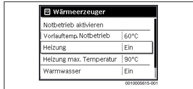
Bild 7 Heizung einschalten
