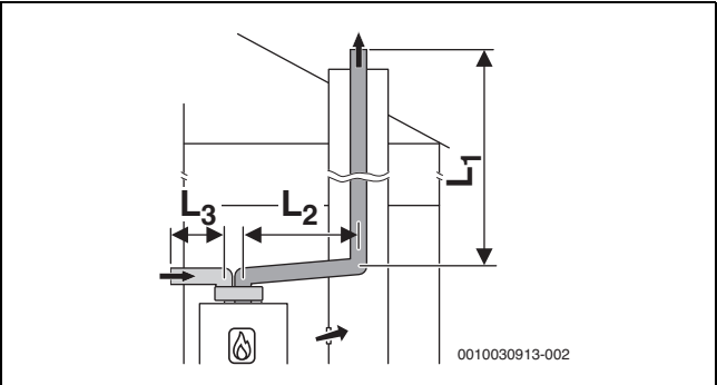
Bild 33 Starre Abgasführung nach C 53(x) im Schacht und Luft-Abgas-Führung mit getrennten Rohren für Luftzufuhr und Abgasableitung im Aufstellraum
