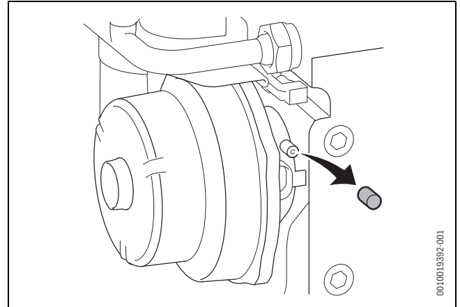
Bild 71 Messstutzen an der Mischeinrichtung
