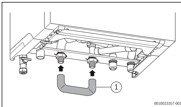
Bild 19 Betrieb ohne Warmwasserspeicher (230 V)
