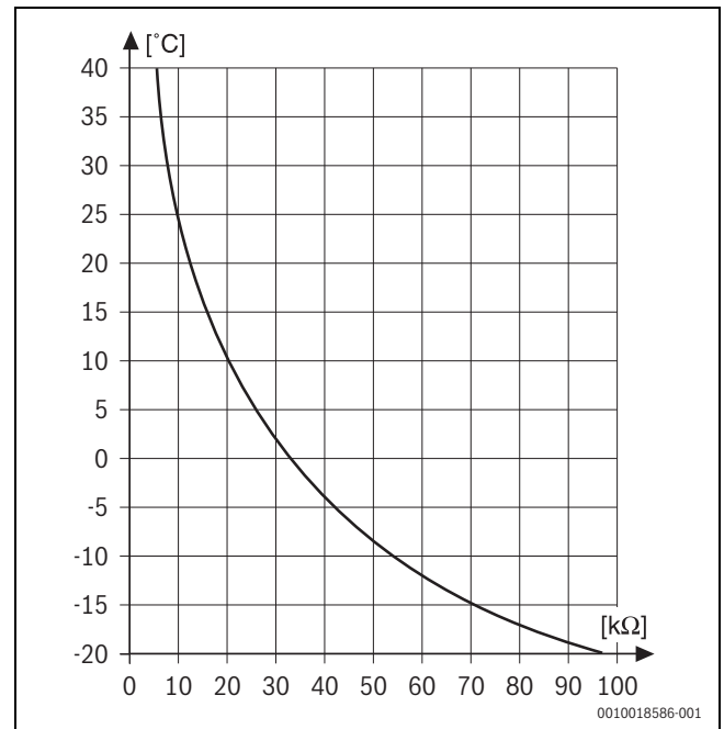
Bild 9 Widerstandskennlinie für Außentemperaturfühler
