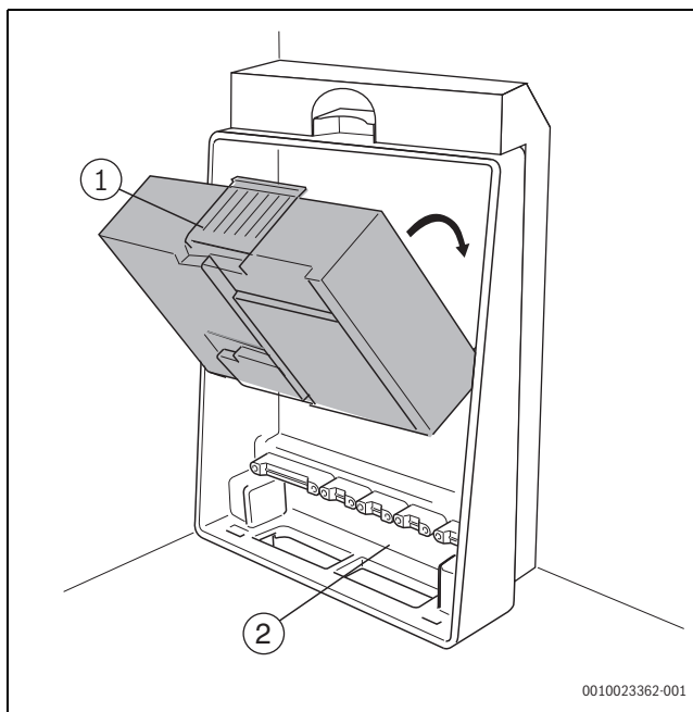
Bild 47 Modul montieren
