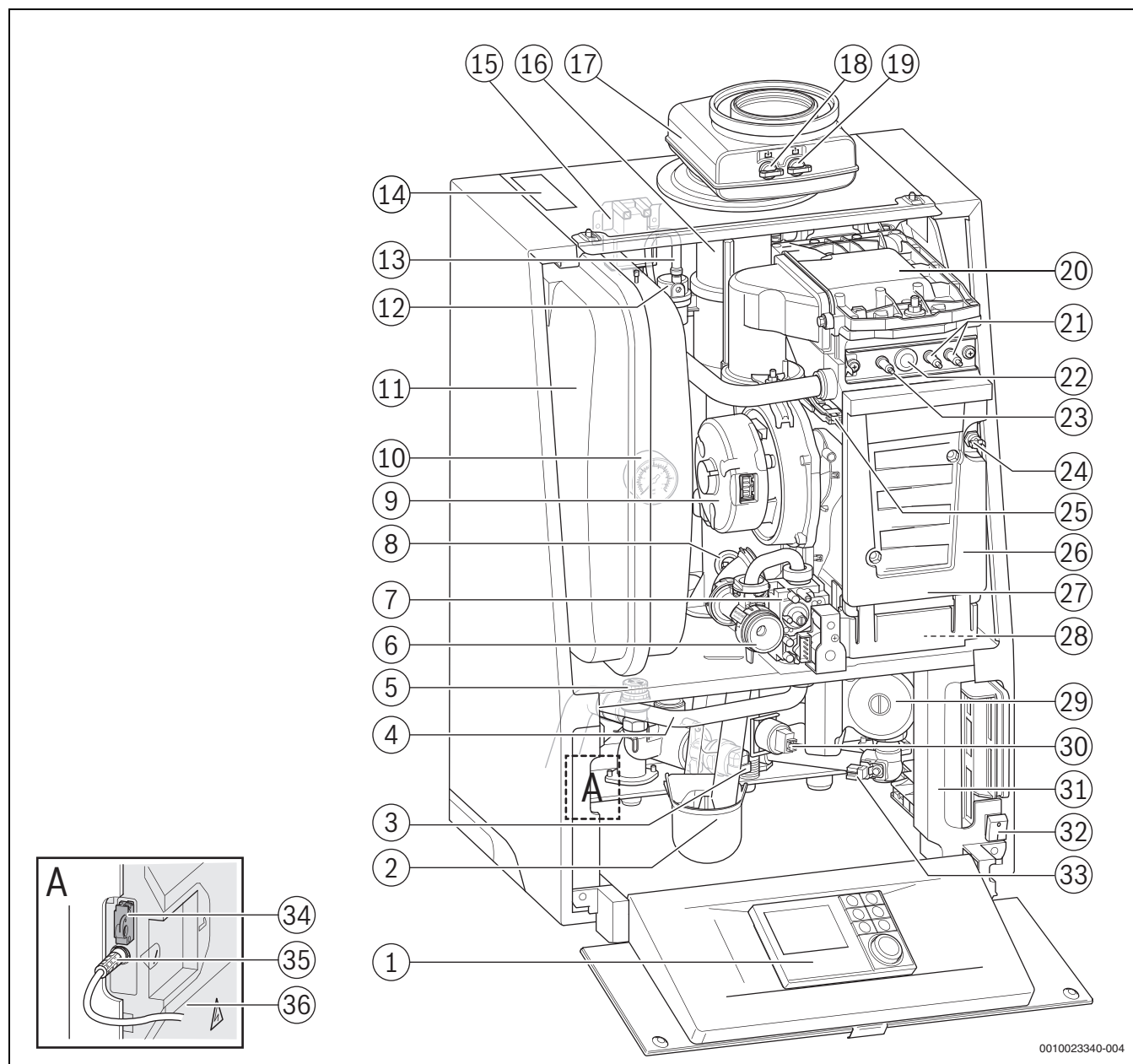
Bild 2 GB192 i
