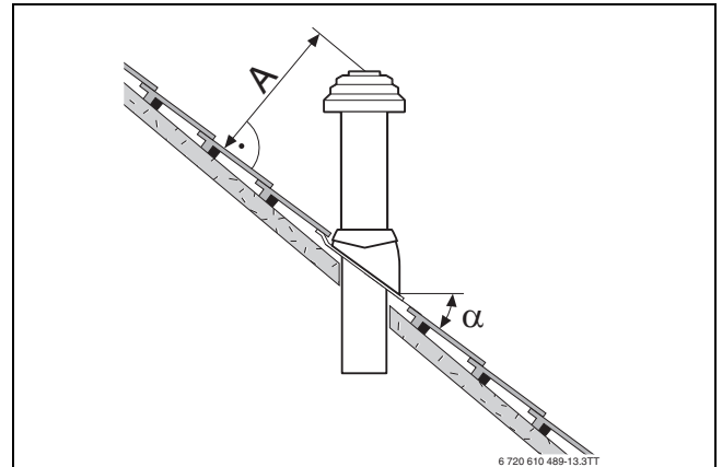
Bild 27 Abstandsmaße und Dachneigungen bei Schrägdach
