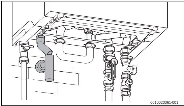
Bild 21 G-TA Kondensatsiphon (Zubehör)
