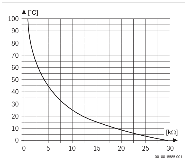
Bild 8 Widerstandskennlinie Temperaturfühler (ausgenommen die Außentemperaturfühler)
