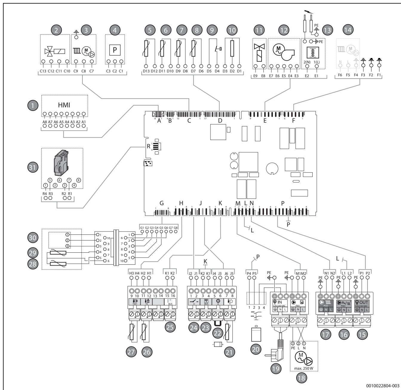
Bild 4 Anschlussplan
