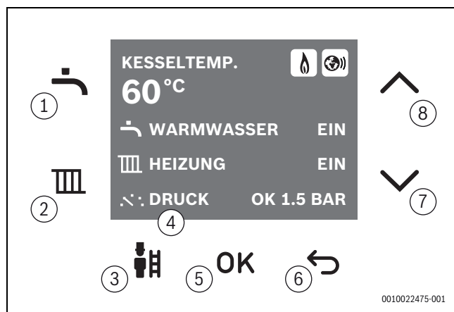
Bild 56 Bedienfeld
