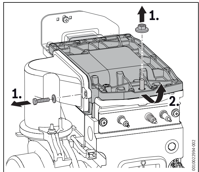
Bild 66 Brennerdeckel ausbauen
