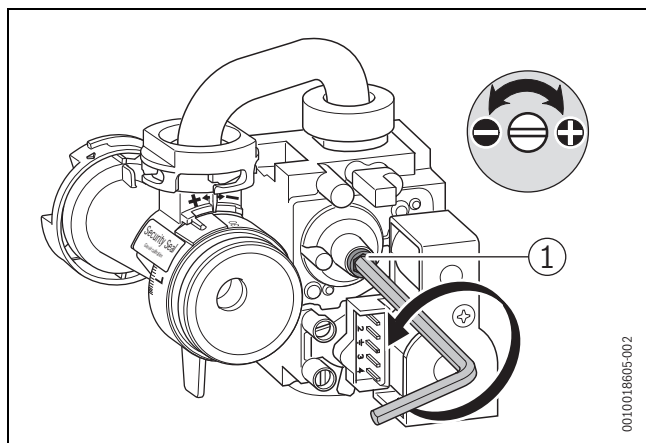
Bild 55 Plombe entfernen
