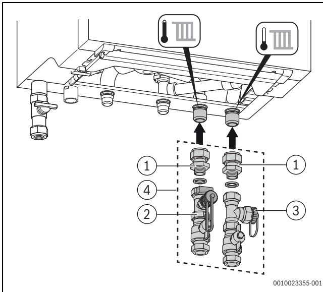
Bild 15 Anschluss der Heizwasserrohre am Gerät
