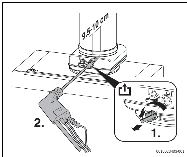
Bild 54 CO/CO 2 -Gehalt messen
