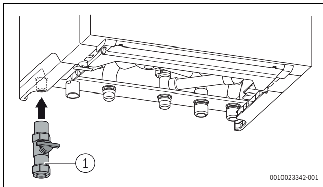
Bild 13 Gasanschluss herstellen
