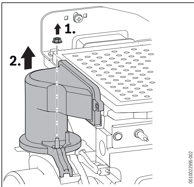
Bild 68 Mischeinrichtung ausbauen
