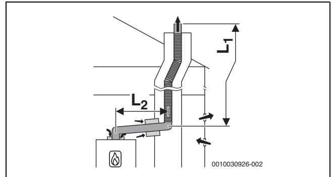
Bild 40 Flexible Abgasführung im Schacht nach B_{23p}/B_{53p} mit raumluftabhängiger Luftzufuhr am Gerät und konzentrischem Verbindungsstück zwischen Aufstellraum und Schacht
