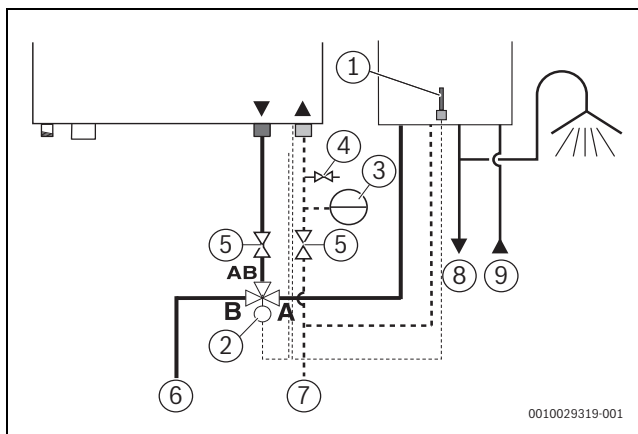
Bild 20 Externes 3-Wege-Ventil montieren
