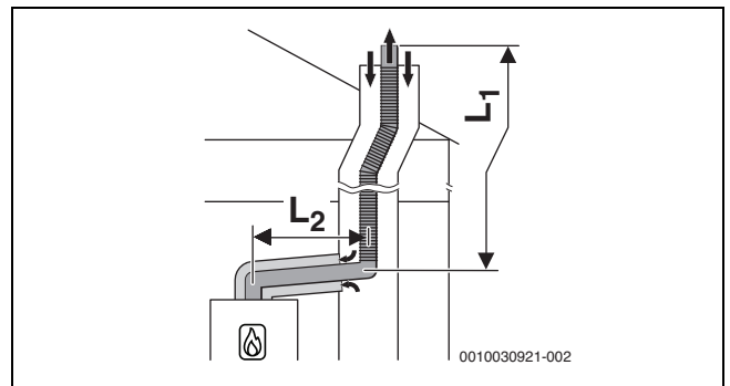
Bild 38 Flexible Abgasführung nach C_{93x} im Schacht und konzentrische Luft-Abgas-Führung im Aufstellraum
