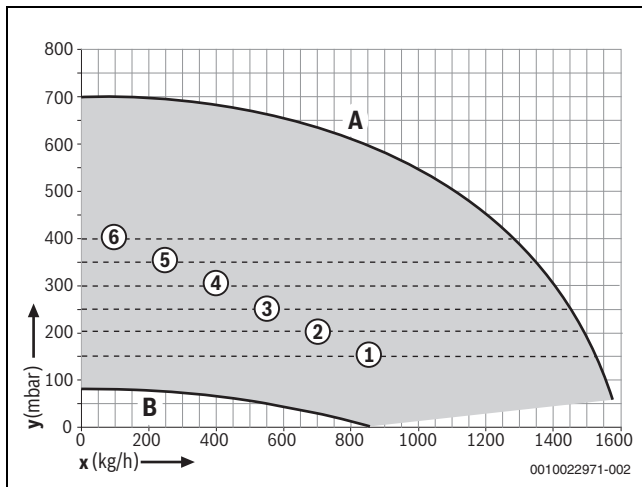
Bild 7 45 kW: Restförderhöhe bei Einstellung 1 - 6
