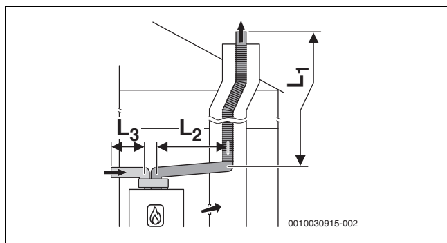
Bild 35 Flexible Abgasführung nach C 53 im Schacht und Luft-Abgas-Führung mit getrennten Rohren für Luftzufuhr und Abgasableitung im Aufstellraum
