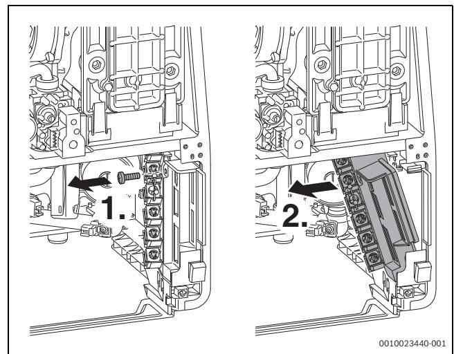
Bild 45 Abdeckung lösen
