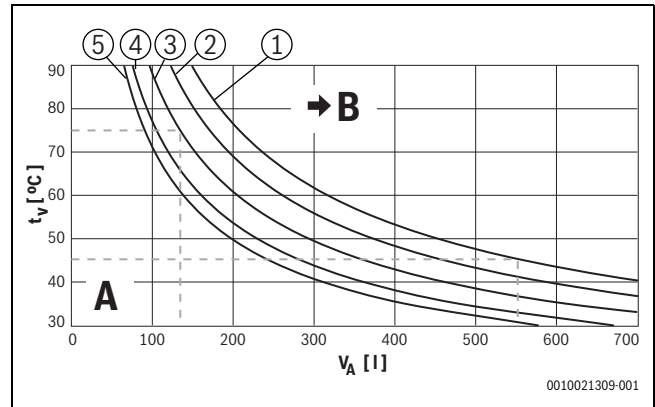
Bild 16 Kennlinien des Ausdehnungsgefäßes, Heizungsausdehnungsgefäß 14 l
