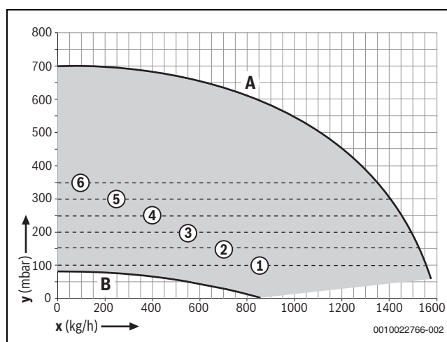
Bild 6 15-35 kW: Restförderhöhe bei Einstellung 1 - 6
