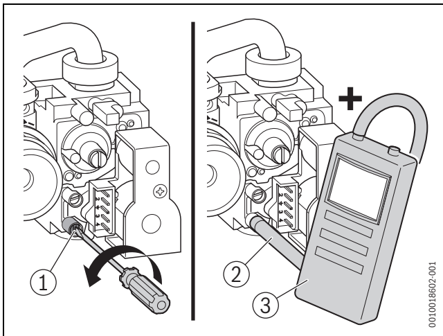
Bild 52 Gas-Anschlussdruck messen
