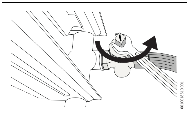
Bild 63 Heizungsanlage bei Frostgefahr entleeren
