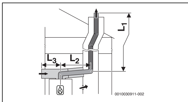
Bild 34 Flexible Abgasführung nach C 53x im Schacht und Luft-Abgas-Führung mit separater Luftzufuhr und konzentrischer Abgasableitung im Aufstellraum
