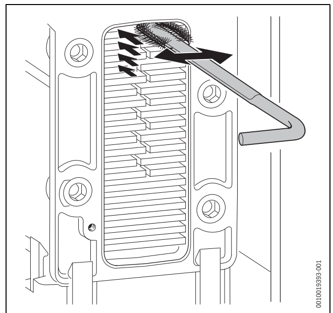
Bild 72 Wärmeblock mit Bürste reinigen
