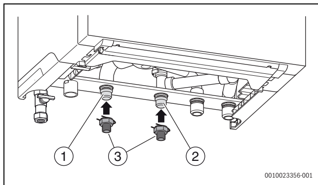
Bild 17 Rohrleitungen für externen Warmwasserspeicher montieren
