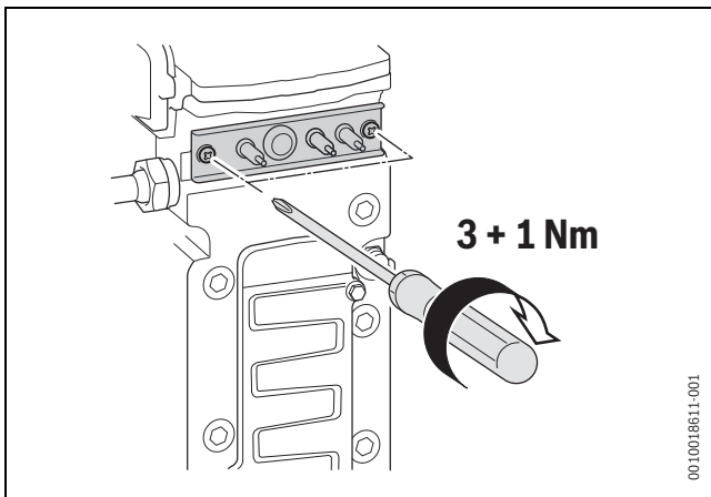
Bild 64 Elektroden-Set montieren
