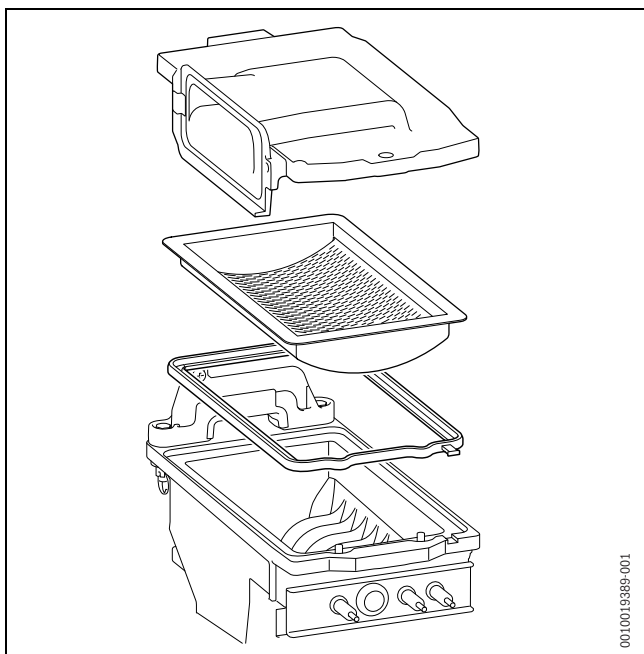
Bild 67 Brenner herausnehmen
