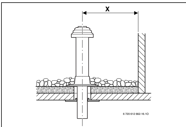
Bild 26 Abstandsmaße bei Flachdach
