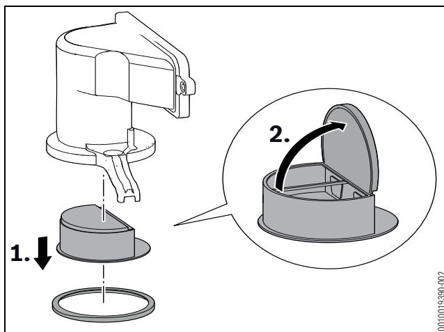
Bild 69 Rückschlagklappe in der Mischeinrichtung
