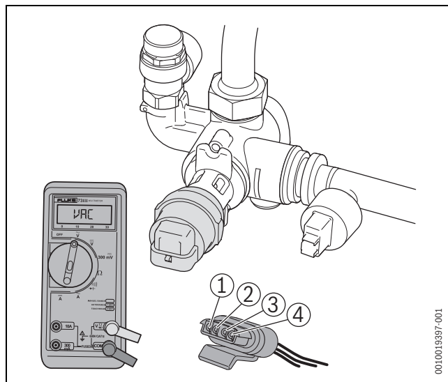
Fig. 75 Vanne à 3 voies
