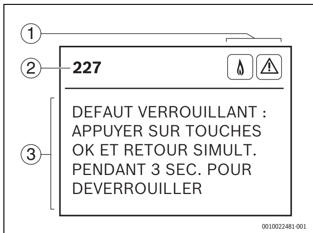
Fig. 76 Menu de défauts
