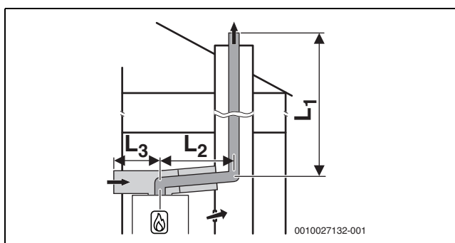
Fig. 32 Conduite d'évacuation des fumées rigide selon C_{53(x)} dans le conduit et circuit d'air et de fumées avec alimentation d'air séparée et conduite d'évacuation des fumées concentrique dans le local d'installation
