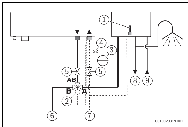
Fig. 20 Monter la vanne à 3 voies externe (230 V)
