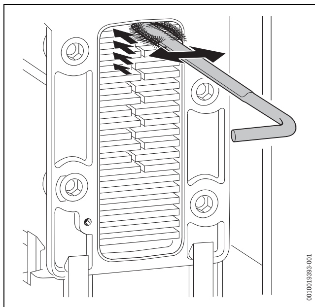
Fig. 72 Nettoyer l'échangeur de chaleur à l'aide de la brosse
