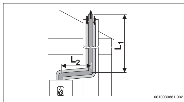
Fig. 30 Circuit d'air et de fumées concentrique selon C_{33x} dans le conduit
