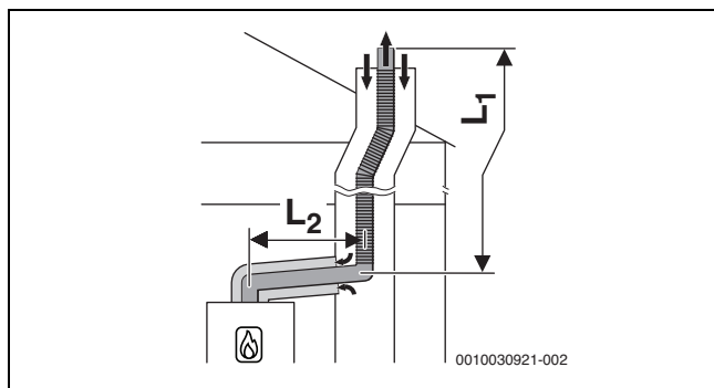
Fig. 38 Evacuation des fumées flexible selon C 93x dans le conduit et circuit d'air et de fumées concentrique dans le local d'installation
