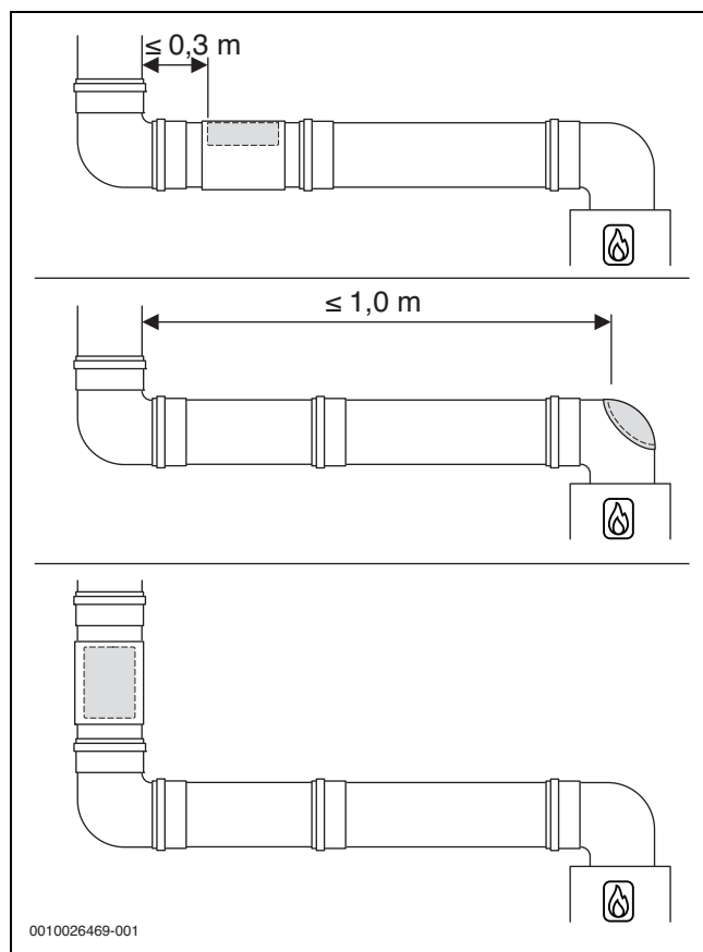
Fig. 23 Disposition de la trappe de visite inférieure
