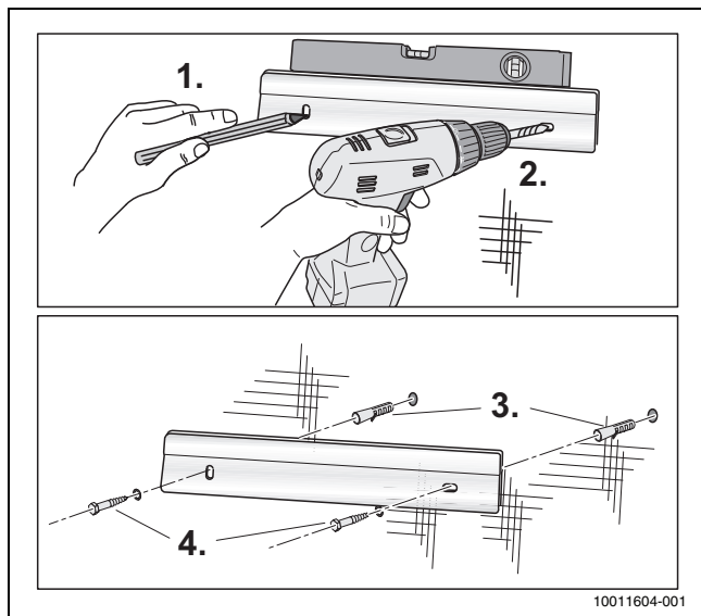
Fig. 11 Montage du support mural
