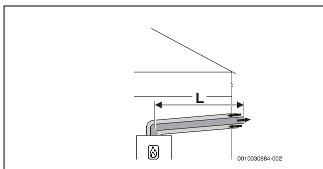
Fig. 29 Circuit d'air et de fumées concentrique horizontal selon C_{13x} par le mur extérieur
