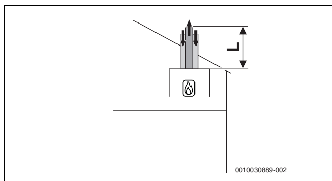
Fig. 31 Circuit d'air et de fumées vertical concentrique selon C_{33(x)}
