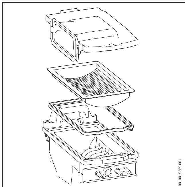
Fig. 67 Retirer le brûleur
