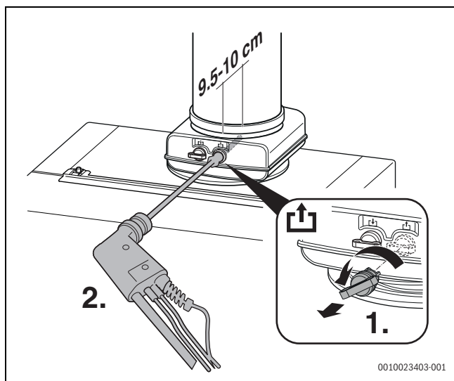
Fig. 54 Mesure de la teneur en CO/CO 2
