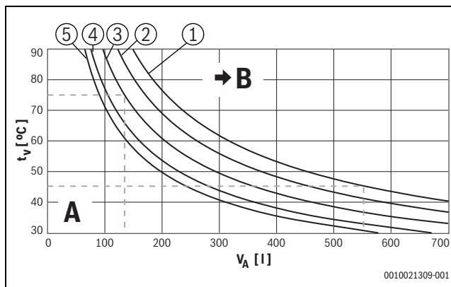
Fig. 16 Courbes caractéristiques du vase d'expansion du chauffage (accessoire vase d'expansion chauffage 14 l)
