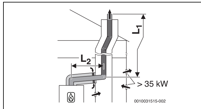
Fig. 42 Evacuation des fumées flexible dans le conduit selon B 33 avec arrivée d'air dépendant de l'air ambiant par le circuit d'air et de fumées concentrique dans le local d'installation
