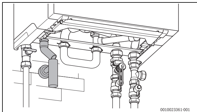
Fig. 21 Siphon de condensats G-TA (accessoire)
