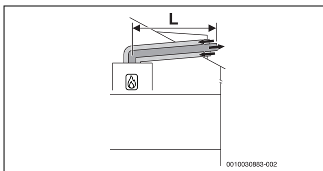
Fig. 28 Circuit d'air et de fumées concentrique horizontal selon C_{13x} par le toit
