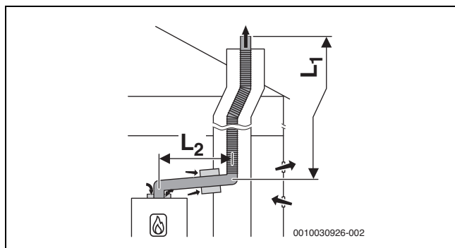
Fig. 40 Evacuation des fumées flexible dans le conduit selon B 23p /B 53p avec alimentation d'air dépendant de l'air ambiant sur l'appareil et pièce de raccordement concentrique entre le local d'installation et le conduit
