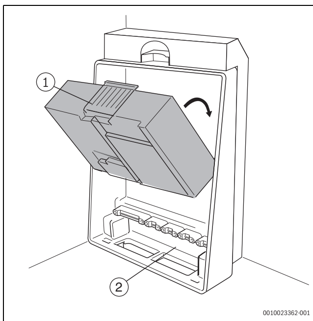
Fig. 47 Monter le module
