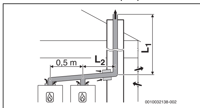
Fig. 43 Cascade avec 2 appareils : évacuation des fumées dans le conduit rigide selon B 23p /B 53p avec arrivée d'air dépendant de l'air ambiant sur l'appareil
