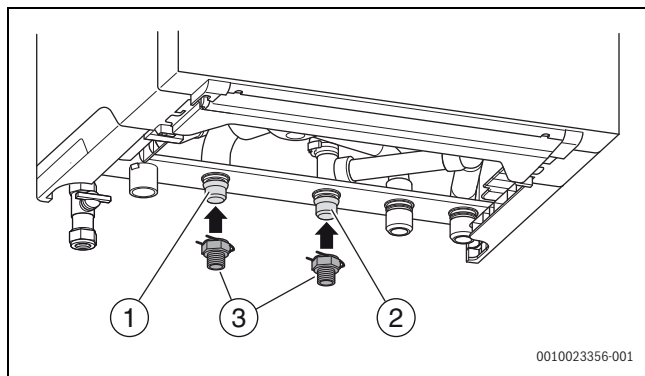
Fig. 17 Monter les conduites pour le ballon ECS externe
