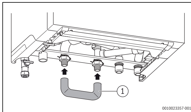
Fig. 19 Fonctionnement sans ballon ECS (230 V)
