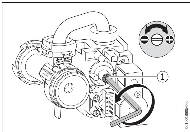
Fig. 55 Retirer le plomb
