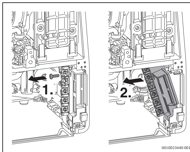
Fig. 45 Couvercle du bornier
