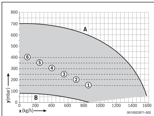
Fig. 7 45 kW: Hauteur de refoulement résiduel au réglage 1 - 6
