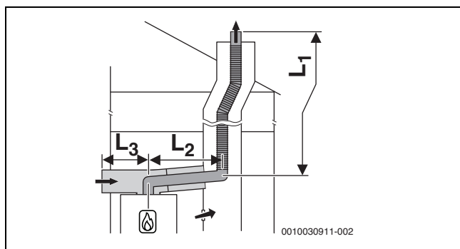
Fig. 34 Conduite d'évacuation des fumées flexible selon C 53x dans le conduit et circuit d'air et de fumées avec alimentation d'air séparée et conduite d'évacuation des fumées concentrique dans le local d'installation
