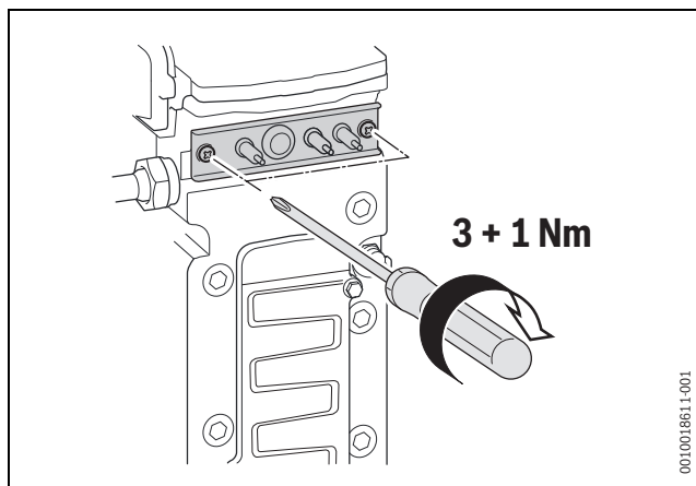
Fig. 64 Monter le jeu d'électrodes
