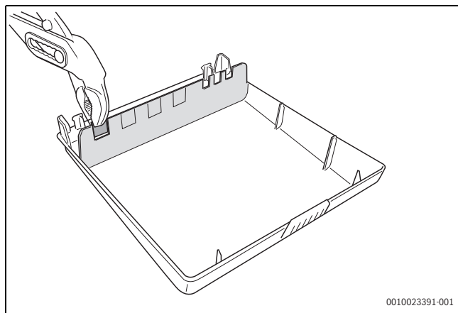
Fig. 49 Enlever le chemin de câbles
