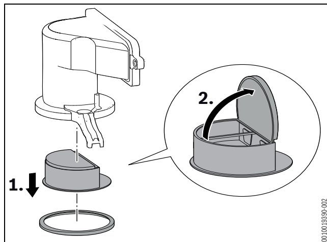
Fig. 69 Clapet anti-retour du dispositif de mélange
