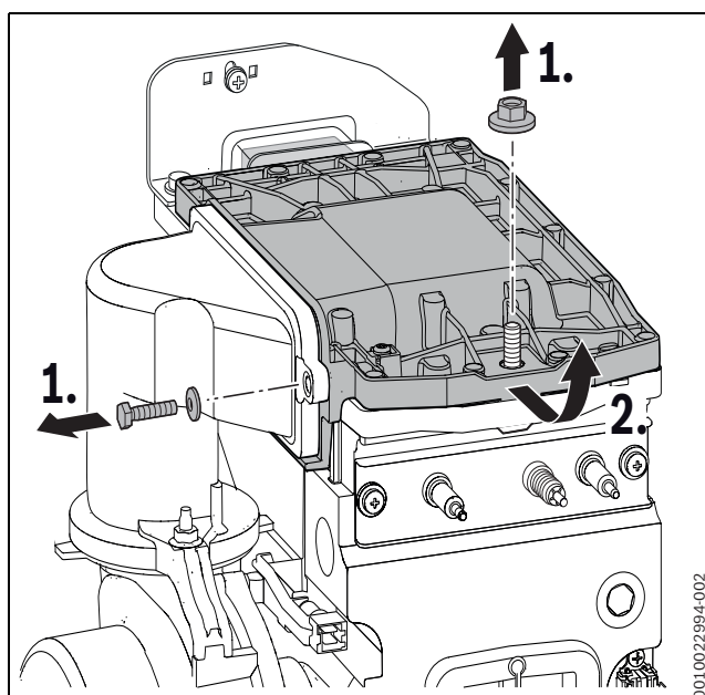
Fig. 66 Démontez le couvercle du brûleur
