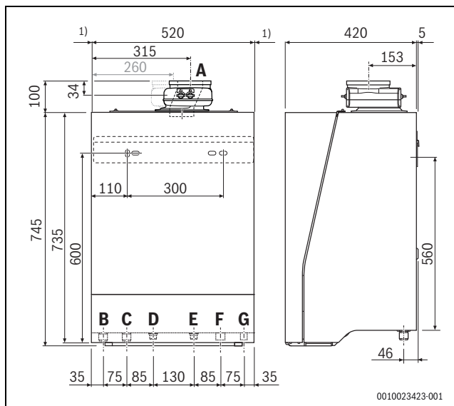
Fig. 3 Dimensions et raccords [mm]
