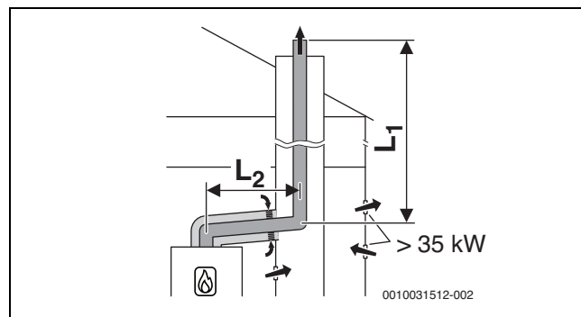
Fig. 41 Evacuation des fumées rigide dans le conduit selon B 33 avec arrivée d'air dépendant de l'air ambiant par le circuit d'air et de fumées concentrique dans le local d'installation
