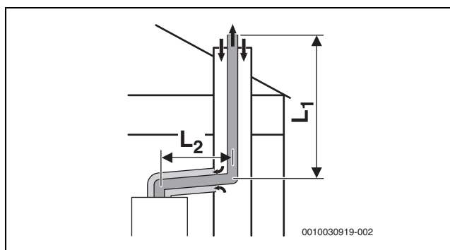
Fig. 37 Evacuation des fumées rigide selon C93x dans le conduit et circuit d'air et de fumées concentrique dans le local d'installation
