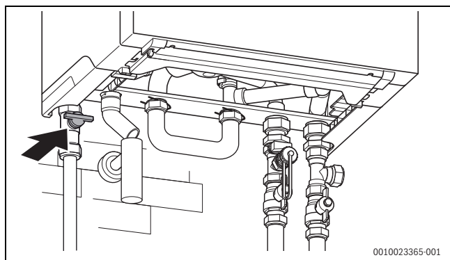
Fig. 62 Robinet de gaz fermé
