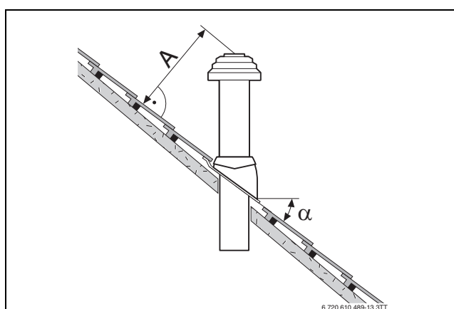
Fig. 27 Distances et inclinaisons de toits inclinés
