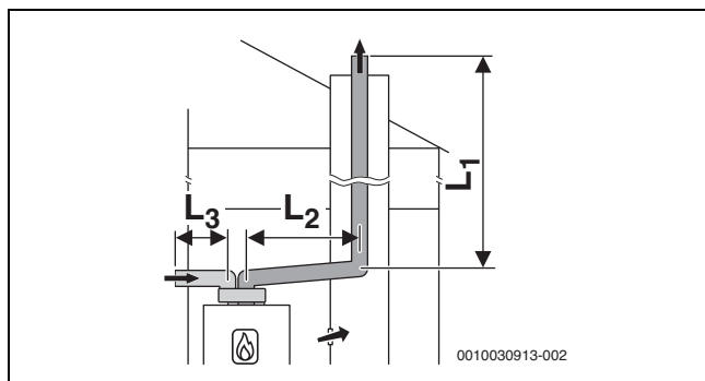
Fig. 33 Starre Abgasführung nach C 53 im Schacht und Luft-Abgas-Führung mit getrennten Rohren für Luftzufuhr und Abgasableitung im Aufstellraum
