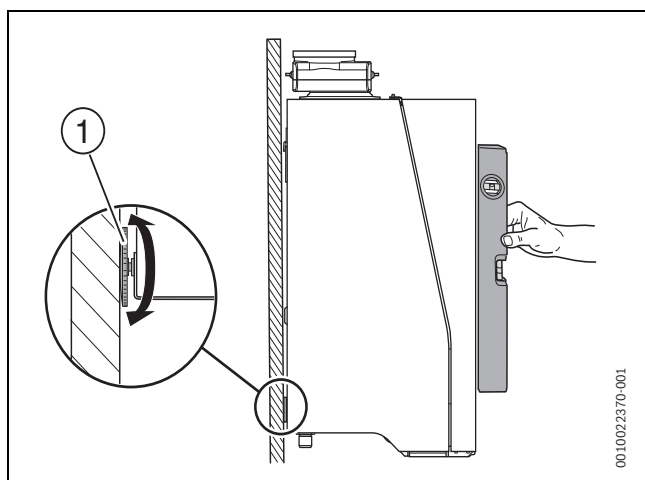
Fig. 12 Positionnement de l'appareil
