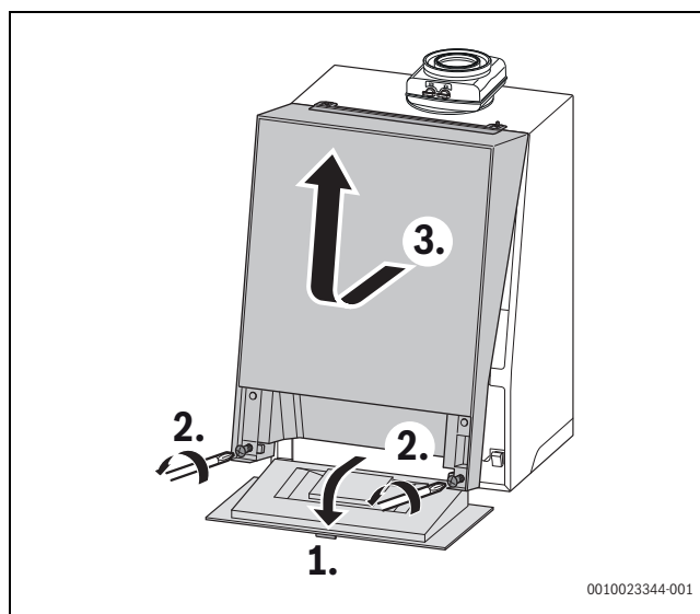
Fig. 14 Démontez le carénage de l'appareil
