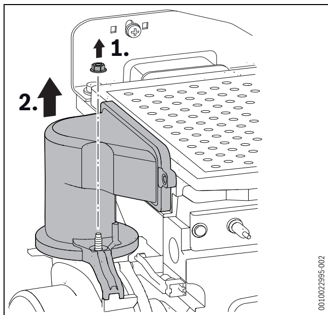
Fig. 68 Démontez le dispositif de mélange
