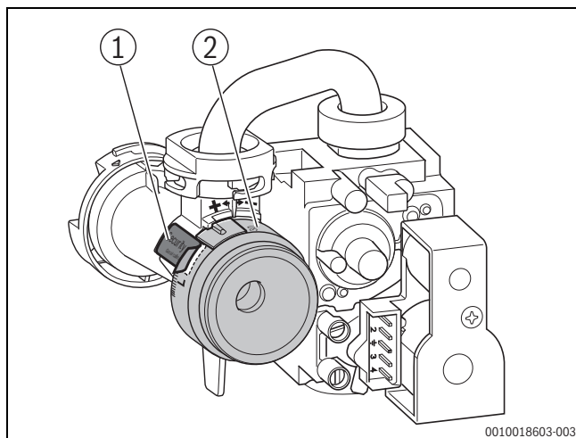
Fig. 53 Libérer l'autocollant
