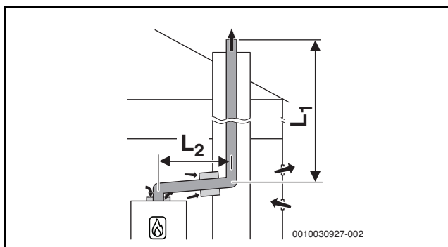
Fig. 39 Evacuation des fumées rigide dans le conduit selon B 23p /B 53p avec alimentation d'air dépendant de l'air ambiant sur l'appareil et pièce de raccordement concentrique entre le local d'installation et le conduit
