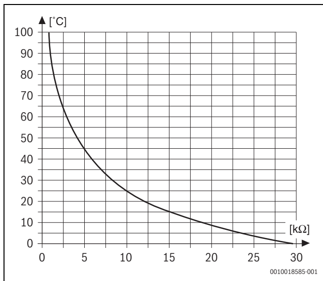
Fig. 8 Courbe caractéristique perte de charge sonde de température (sauf sonde de température extérieure)
