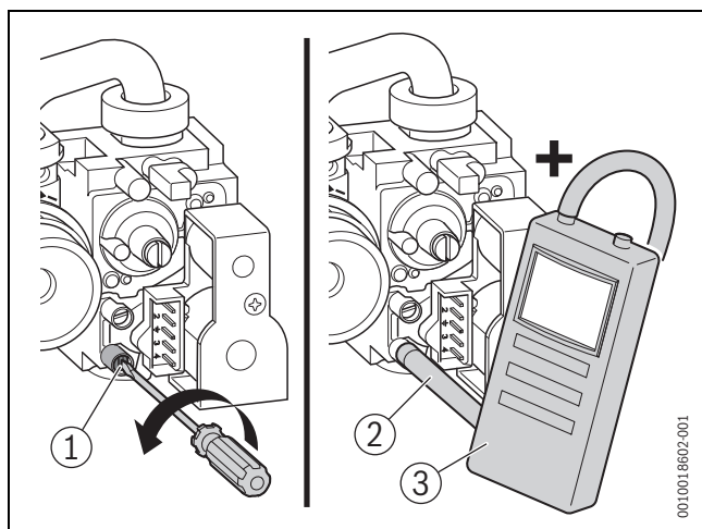
Fig. 52 Mesure de la pression de raccordement du gaz
