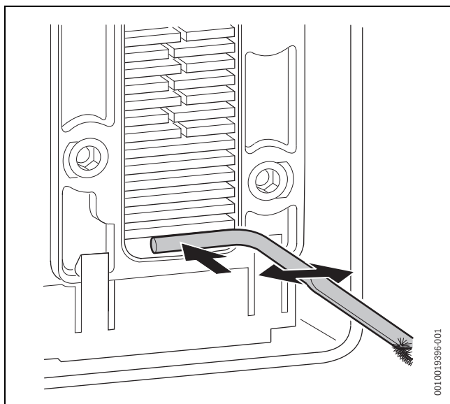
Fig. 74 Nettoyer le bac des condensats
