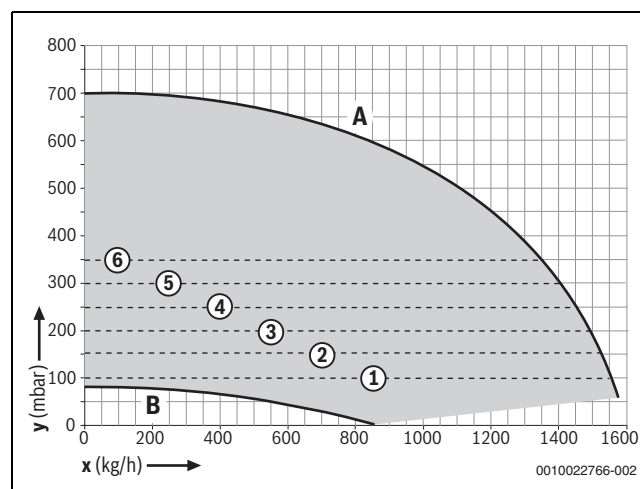
Fig. 6 15-35 kW: Hauteur de refoulement résiduel au réglage 1 - 6
