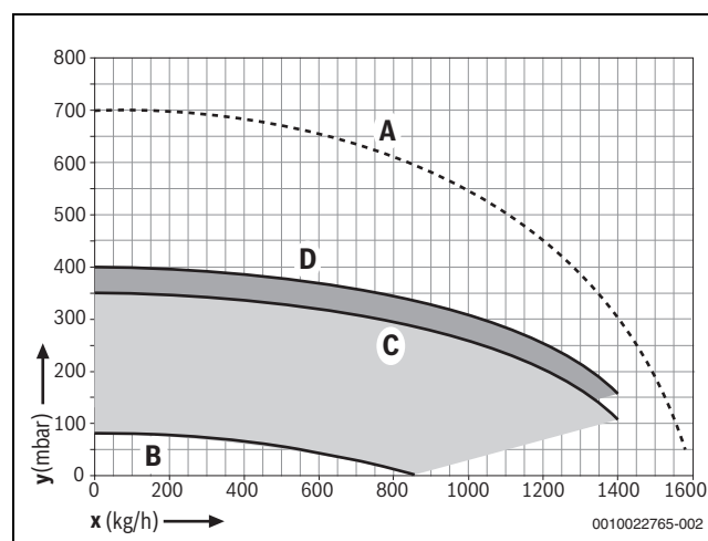
Fig. 5 Hauteur de refoulement résiduel au réglage 0
