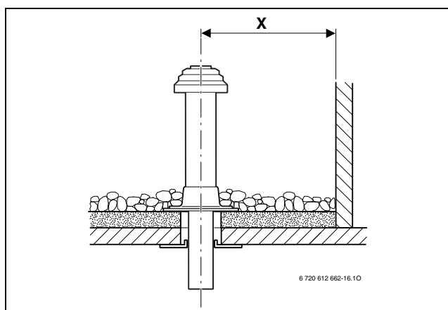
Fig. 26 Distances pour les toits terrasses
