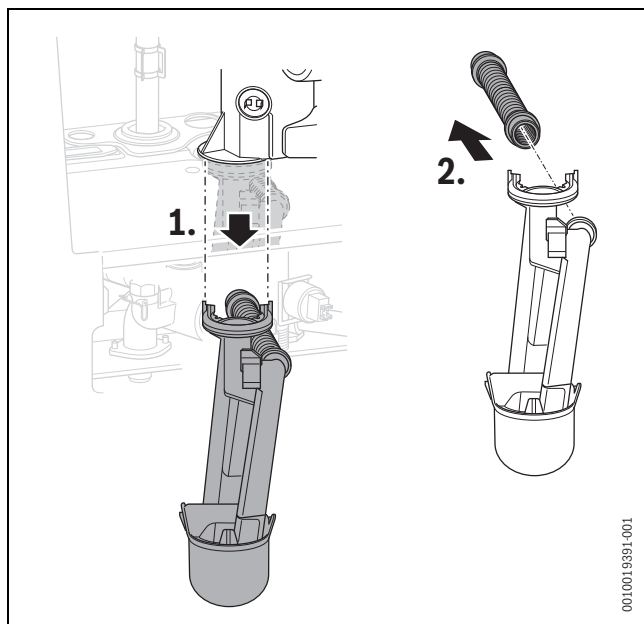
Fig. 70 Siphon de condensats
