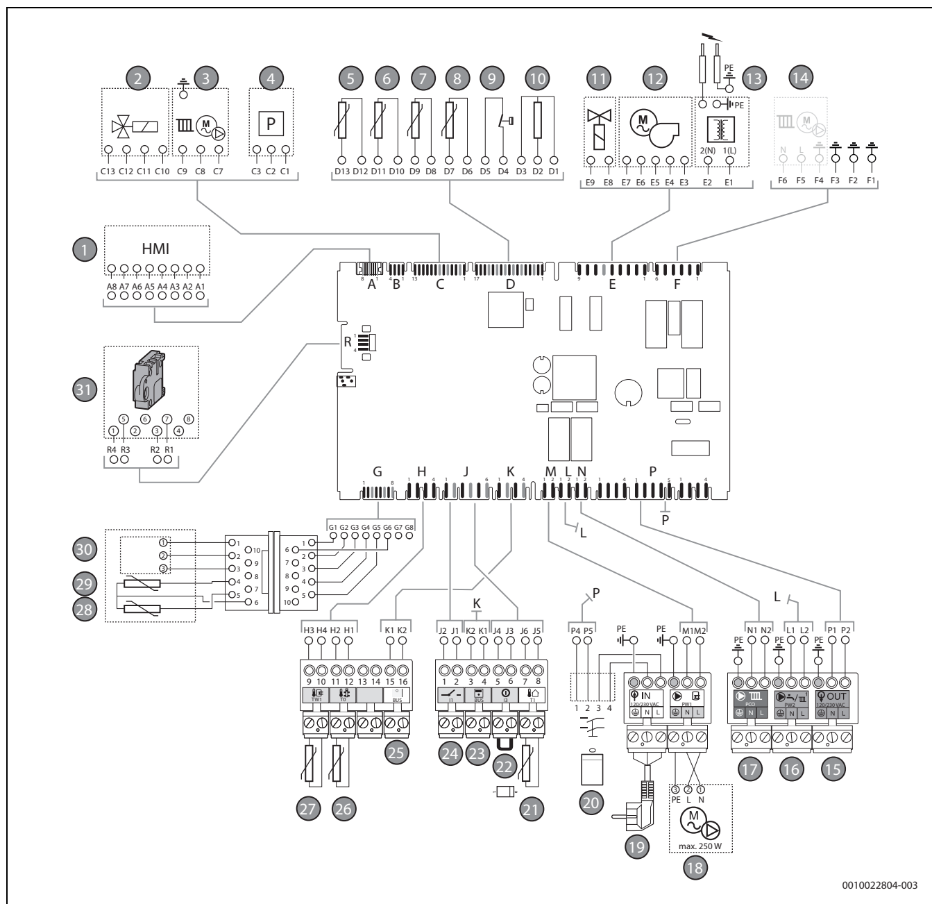
Fig. 4 Schéma de connexion
