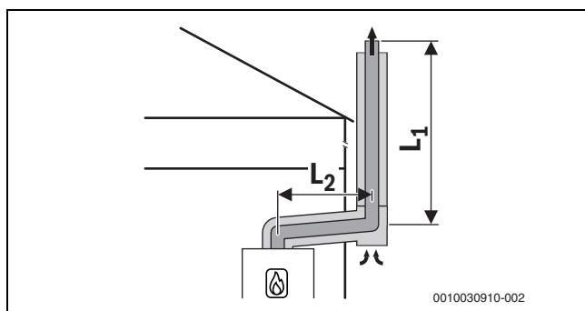
Fig. 36 Circuit d'air et de fumées concentrique selon C53x sur le mur extérieur
