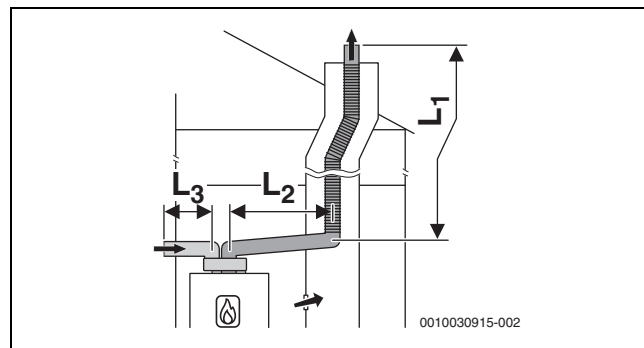
Fig. 35 Flexible Abgasführung nach C 53 im Schacht und Luft-Abgas-Führung mit getrennten Rohren für Luftzufuhr und Abgasableitung im Aufstellraum
