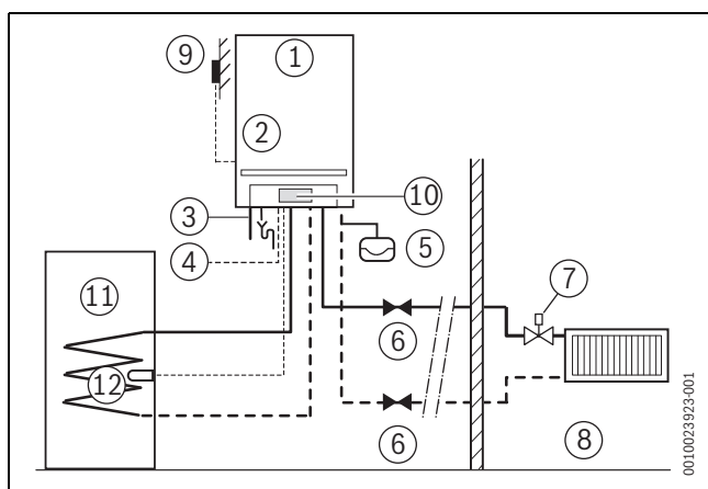
Fig. 18 Exemple d'application avec régulation en fonction de la température extérieure et ballon ECS
