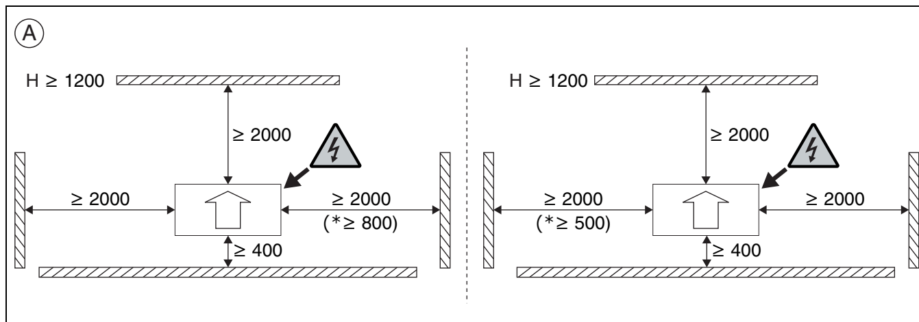
Fig. 5 Distanze in fase di installazione
