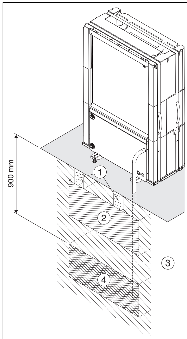
Fig. 8 Scarico condensa nel letto di drenaggio di ghiaia
