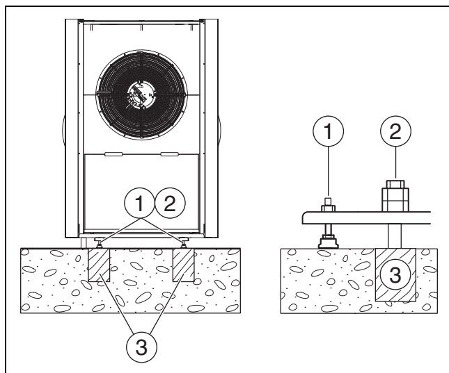
Fig. 10 Fissaggio della pompa di calore
