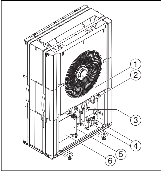
Fig. 2 Panoramica del prodotto
