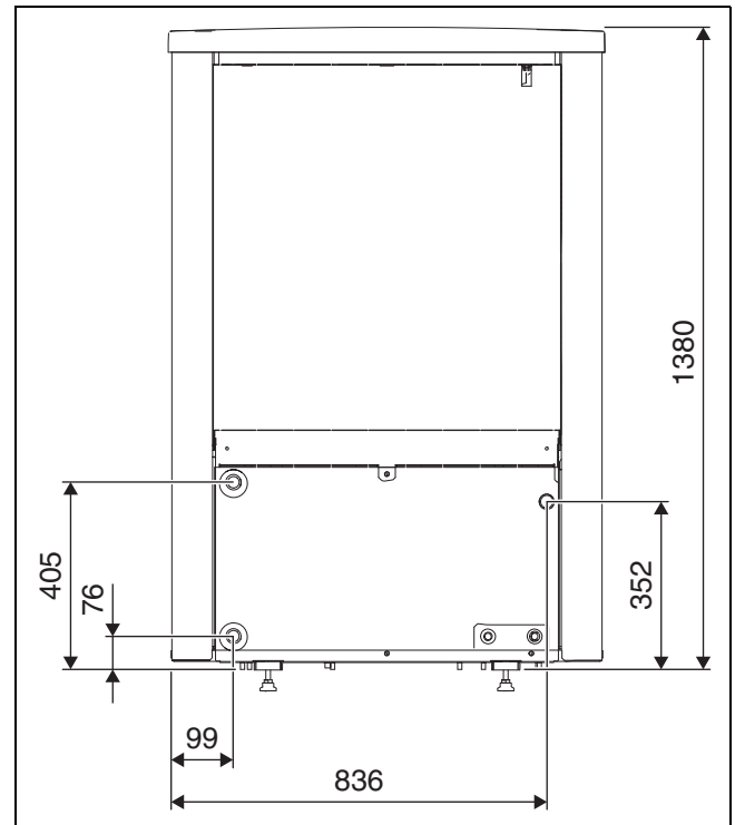
Fig. 3 Dimensioni e attacchi del modello di pompa di calore ODU4.2i S+ / ODU6.2i S+, lato posteriore
