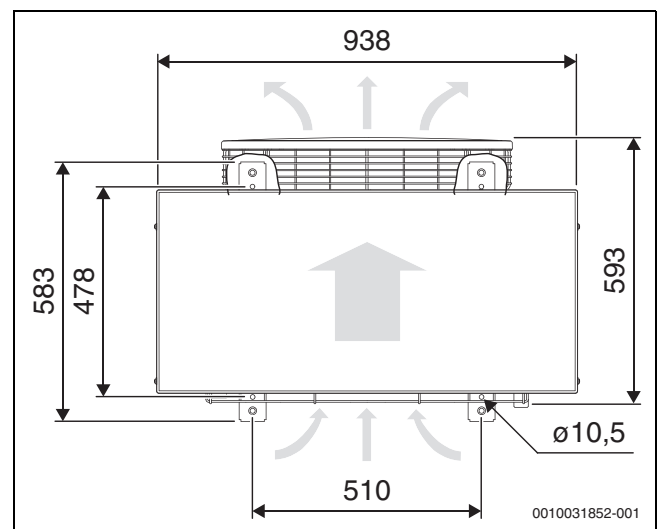
Fig. 4 Dimensioni del modello di pompa di calore ODU4.2i S+ / ODU6.2i S+, vista dall'alto
