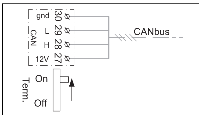
Fig. 13 Terminazione CAN-BUS
