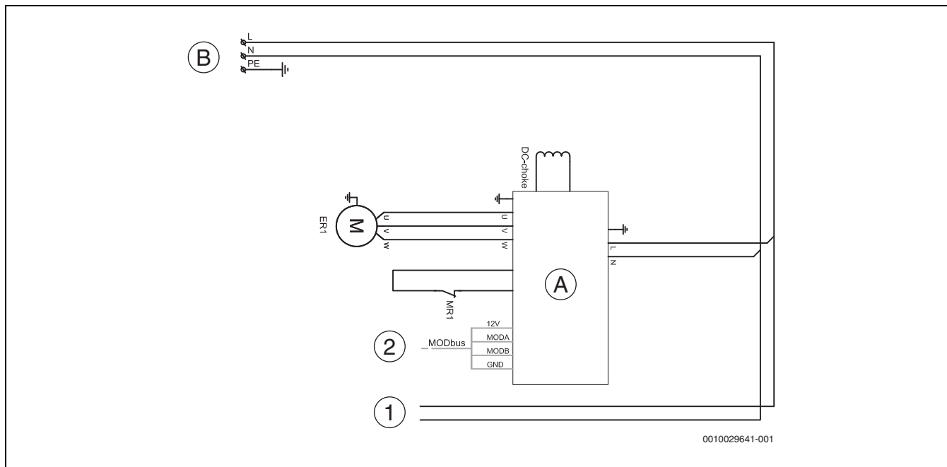
Fig. 19 Schema elettrico per inverter, corrente alternata / alimentazione elettrica trifase
