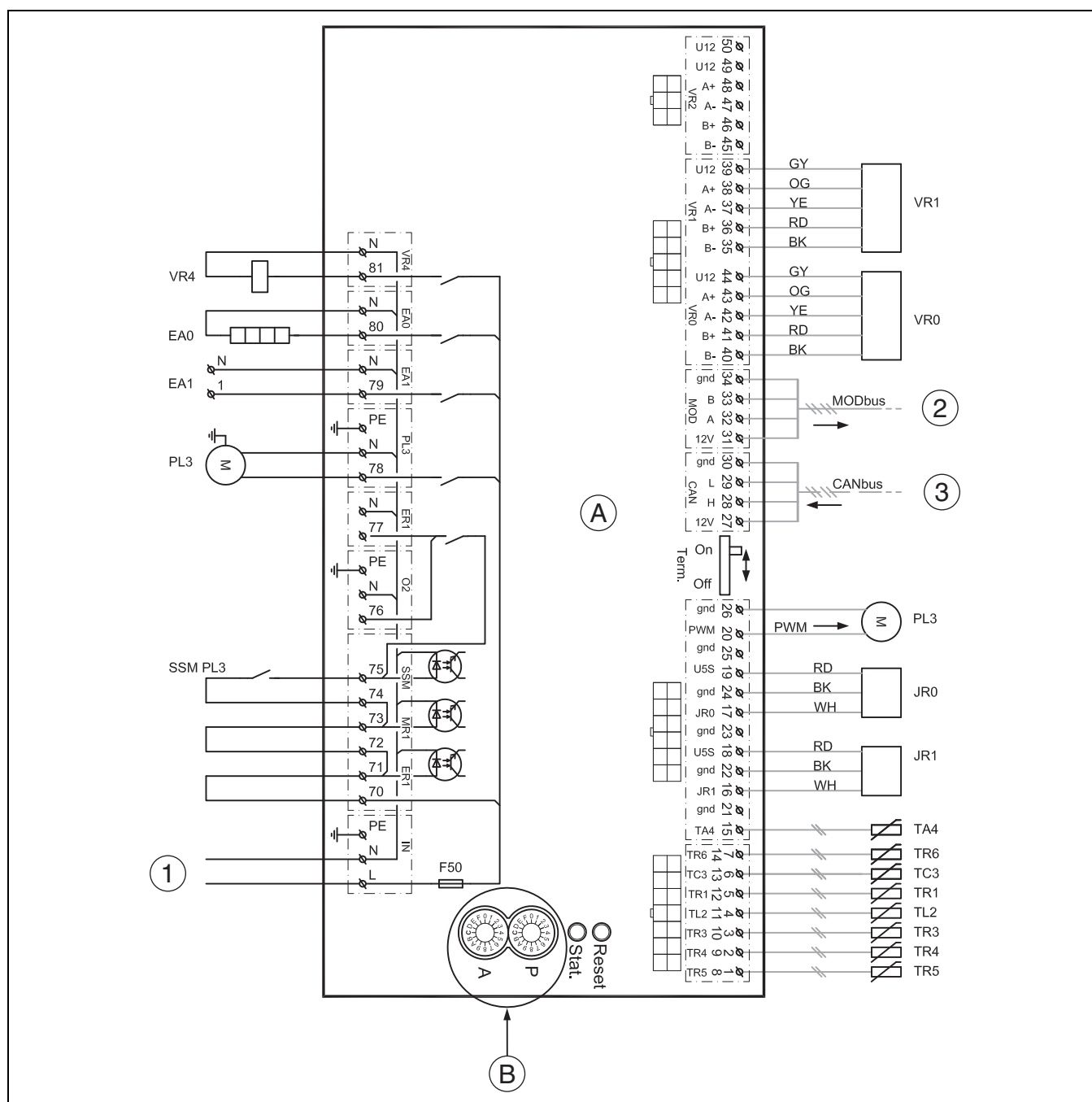
Fig. 20 Schema elettrico per modulo I/O
