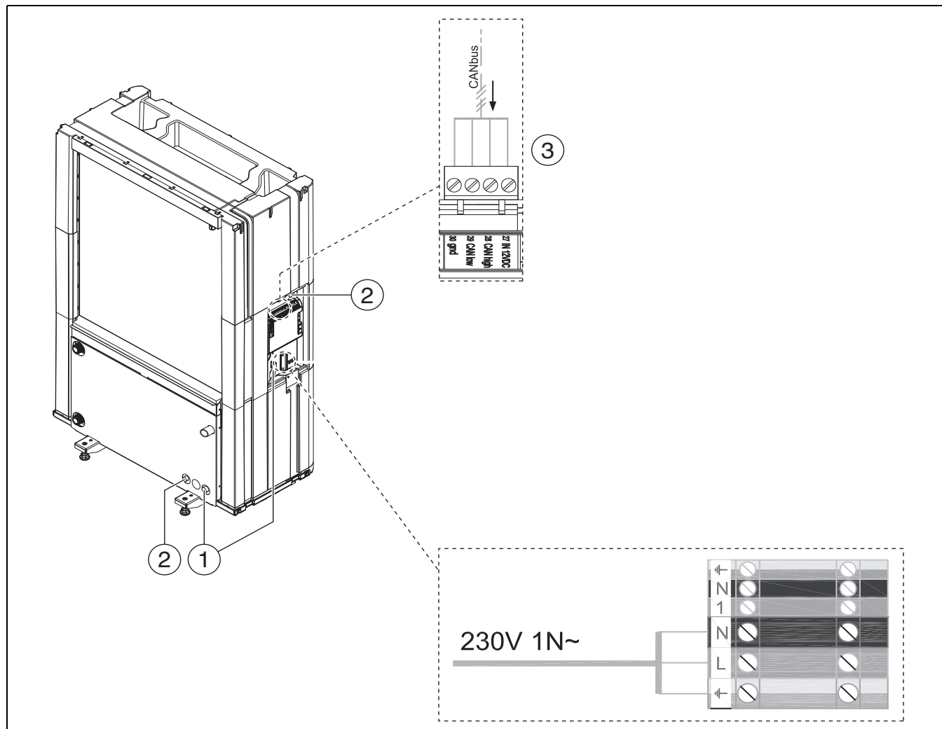
Fig. 14 Canali passacavi e unità di comando
