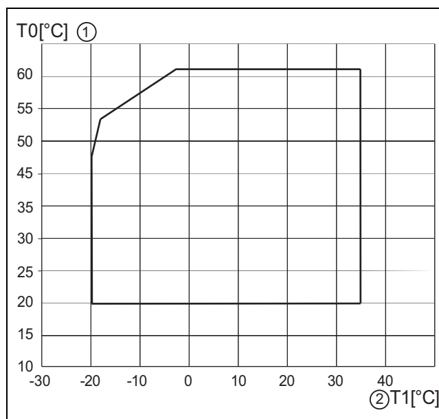
Fig. 17 Pompa di calore senza generatore di calore supplementare
