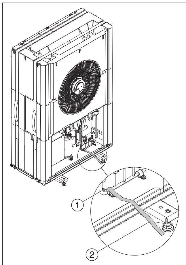
Fig. 9 Dispositivo di sicurezza per il trasporto
