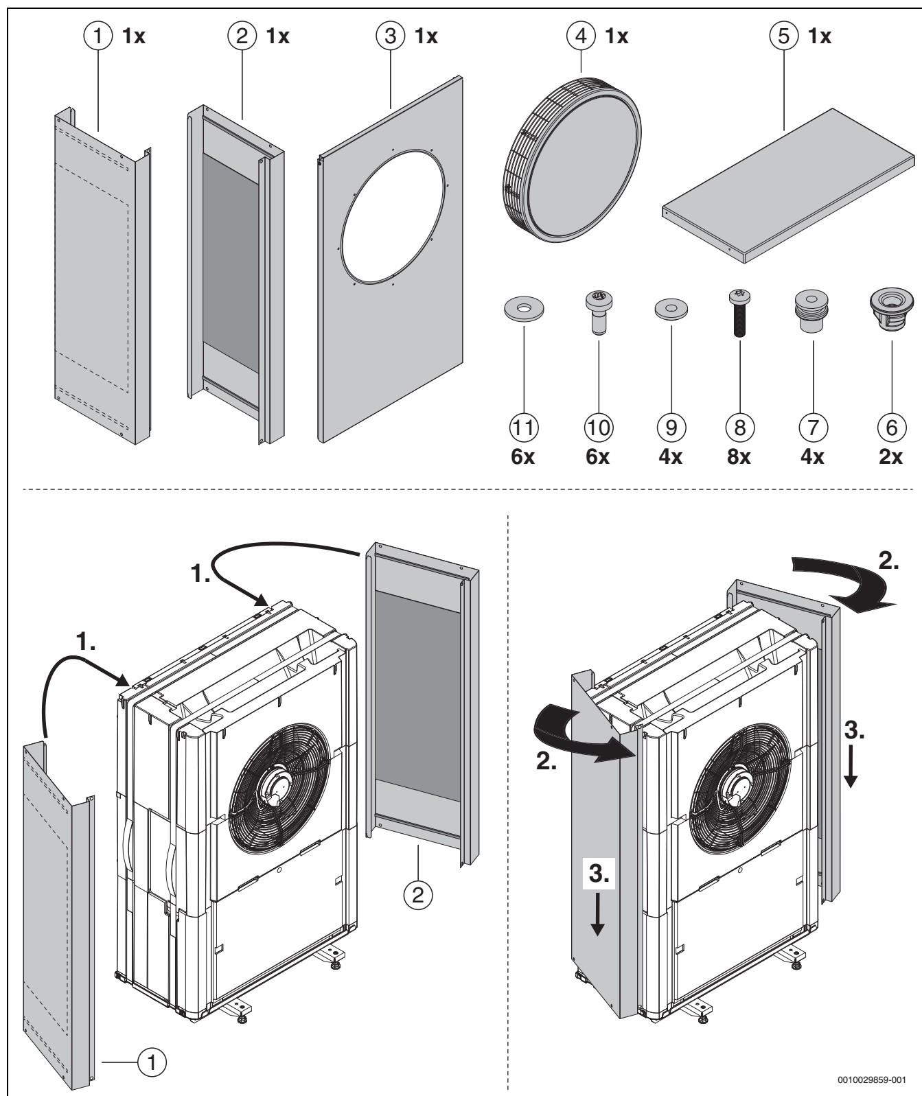
Fig. 15 Montaggio dei pannelli laterali e del coperchio
