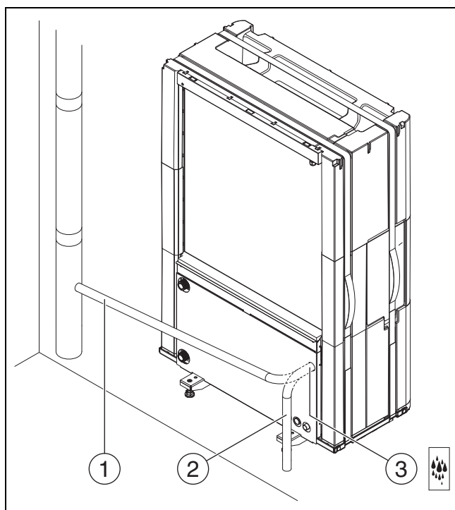
Fig. 11 Raccordi dei tubi per la condensa, validi per tutte le dimensioni
