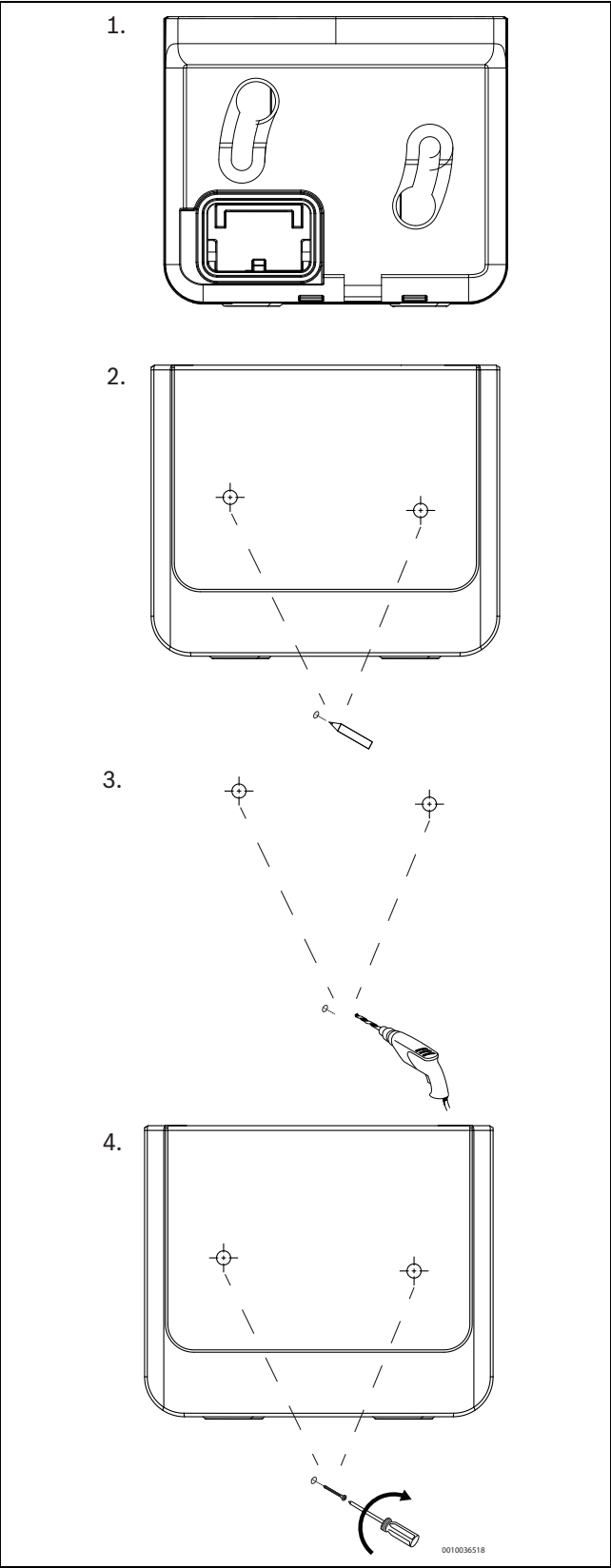
Fig. 18 Monter le support au mur
