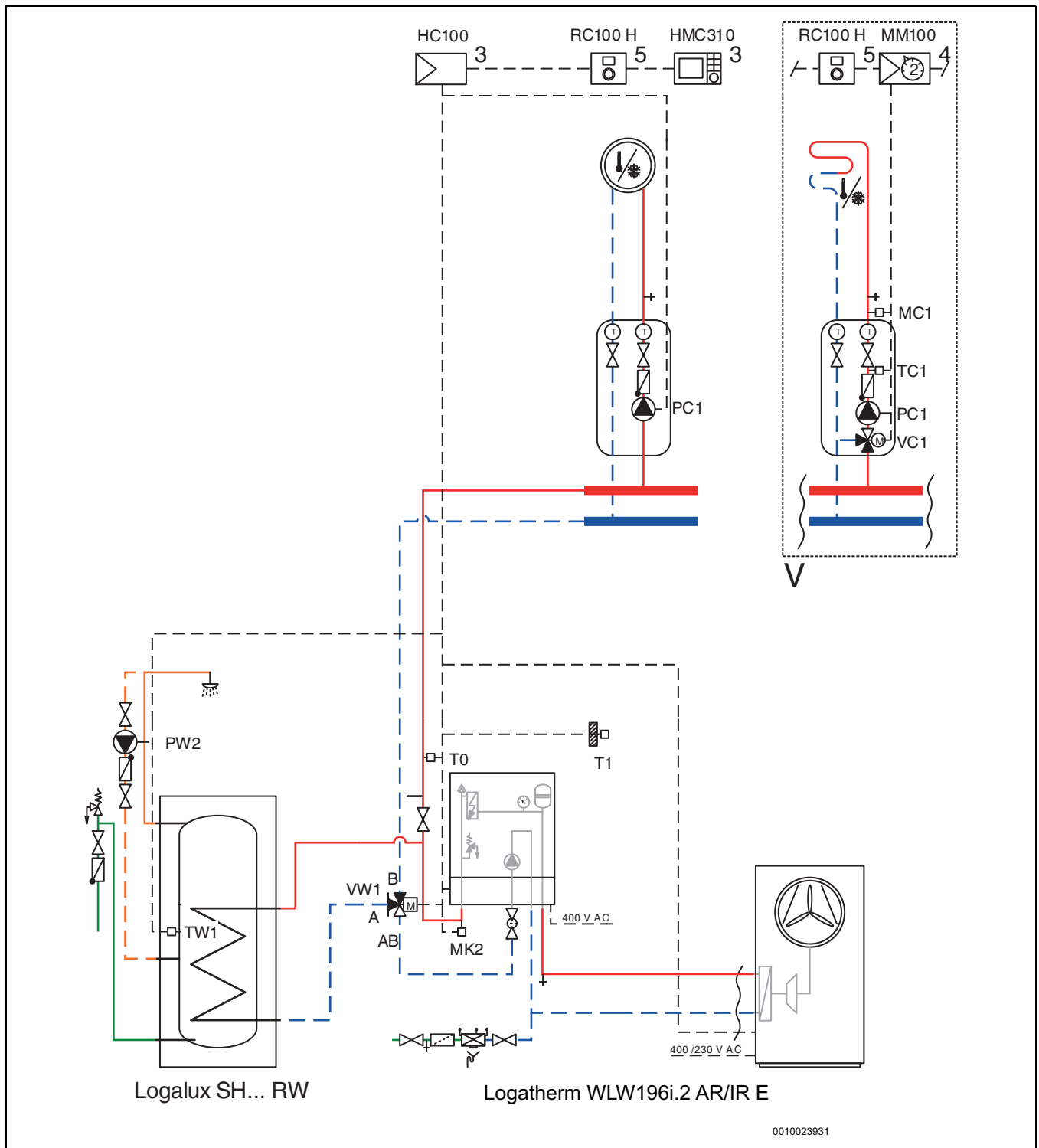
Fig. 32 Chauffage d'appoint électrique avec préparateur d'eau chaude sanitaire
