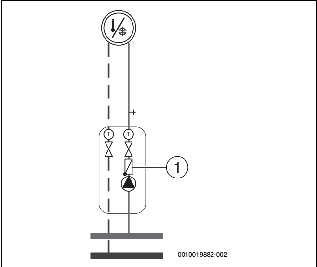
Fig. 31 Circuit de chauffage
