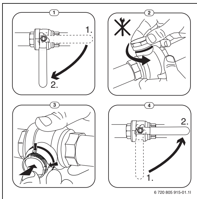
Fig. 21 Nettoyage du filtre
