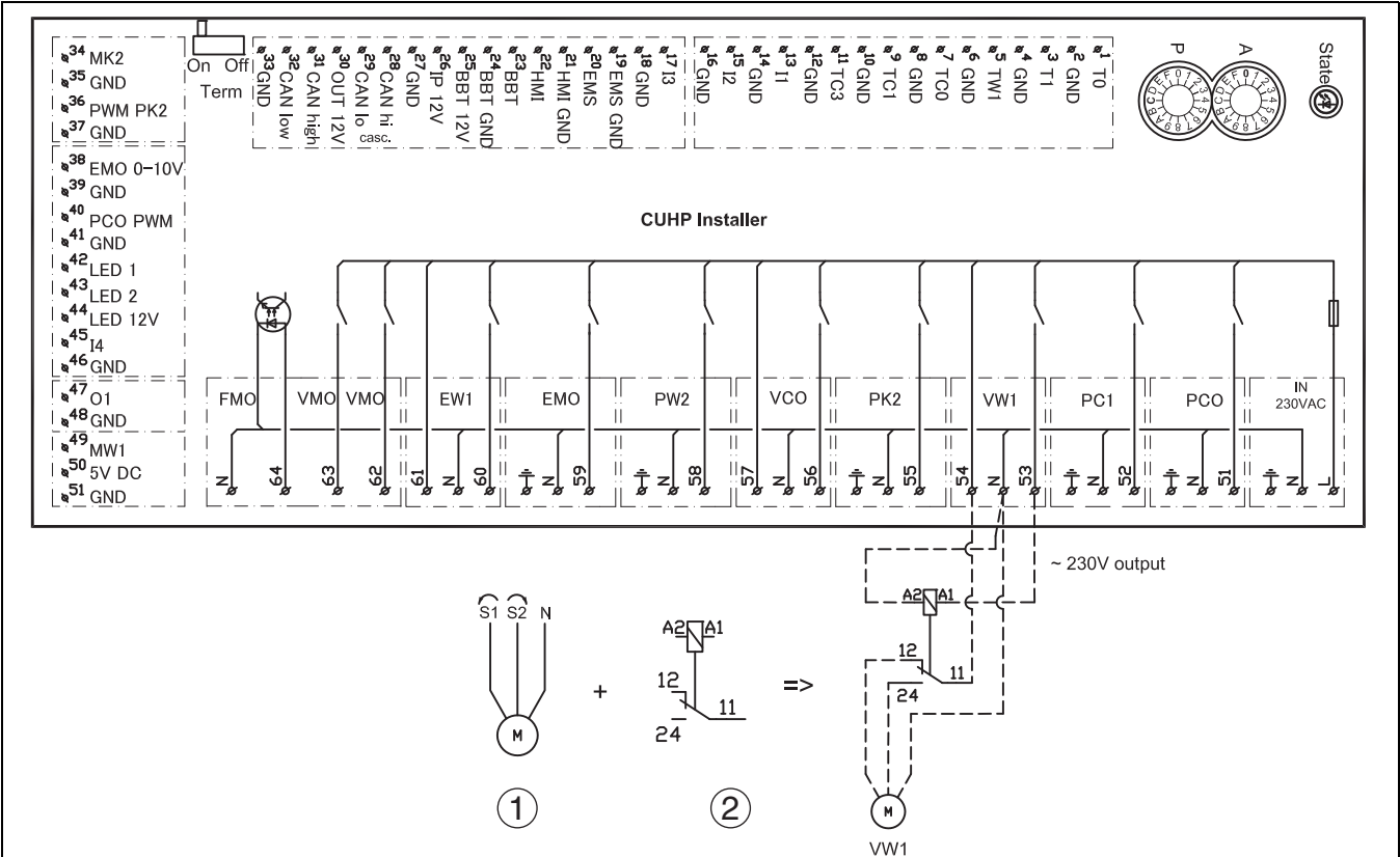
Fig. 37 Alternative d'installation de la vanne sélective
