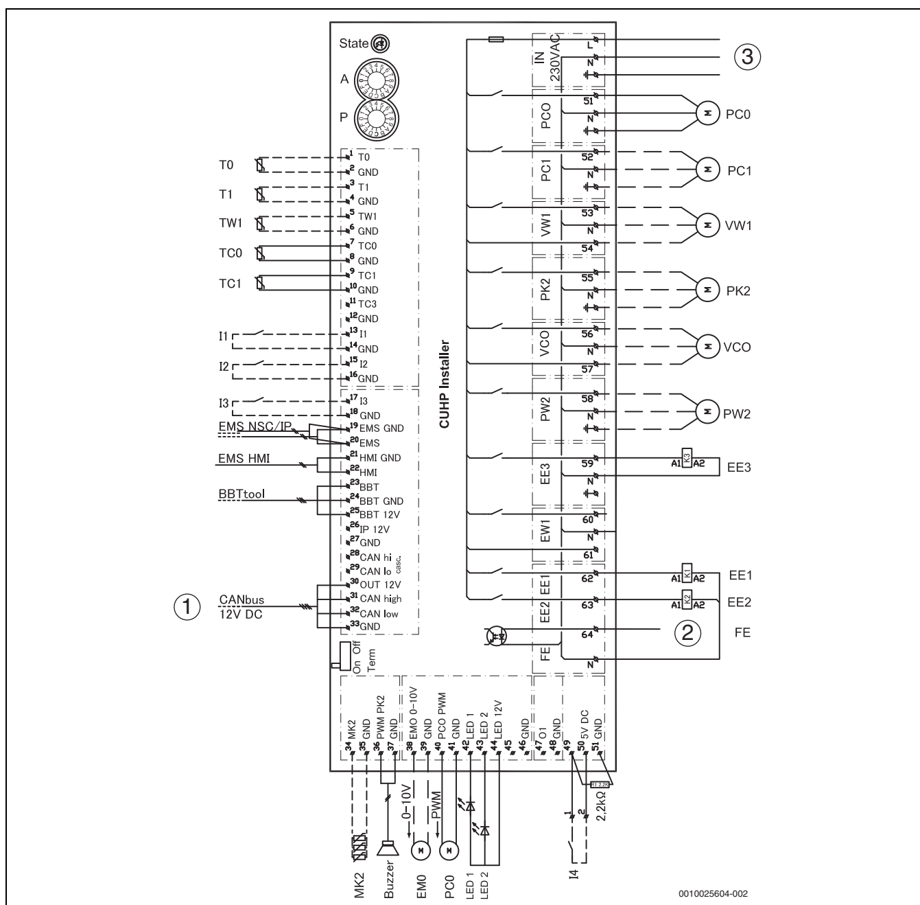
Fig. 36 Schéma de connexion du module d'installation avec chauffage d'appoint électrique intégré
