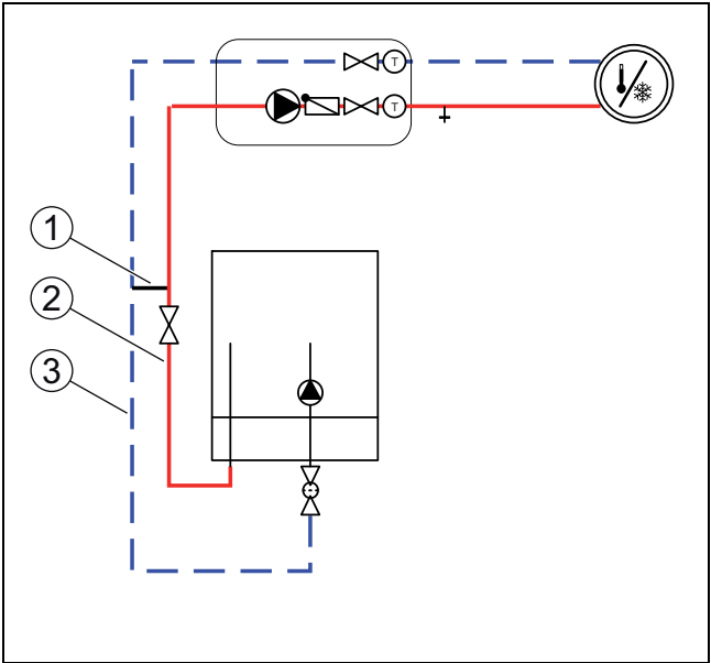
Fig. 30 Unité intérieure avec circuit de chauffage et by-pass
