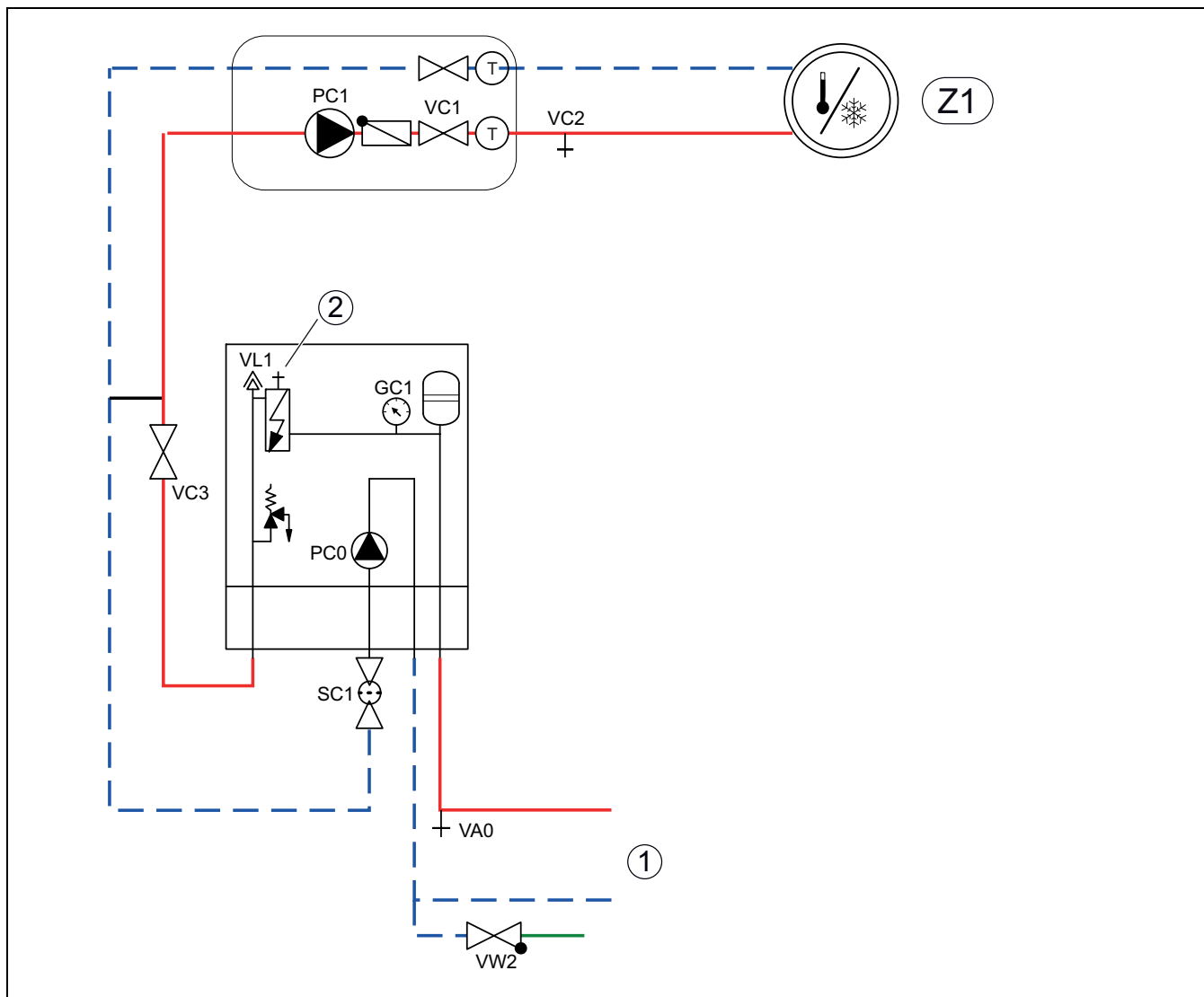
Fig. 20 Unité intérieure avec chauffage d'appoint électrique intégré et système de chauffage
