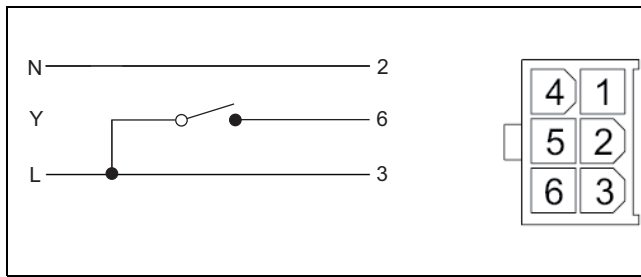
Fig. 27 Connecteur Molex
