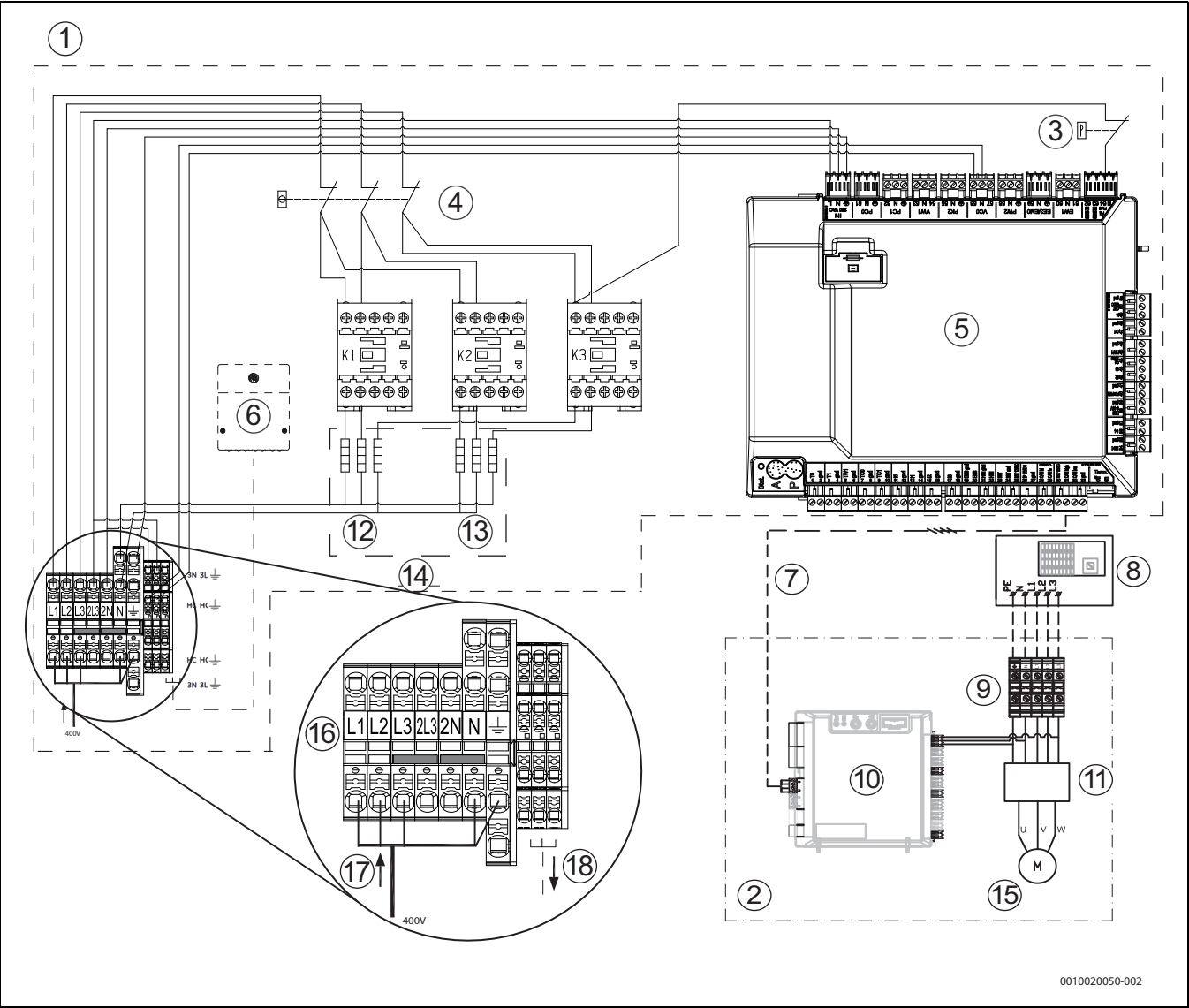
Fig. 35 Pompe à chaleur (courant triphasé) avec chauffage d'appoint électrique intégré (courant triphasé)
