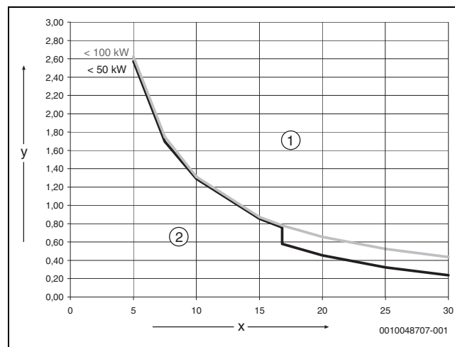
Fig. 1 Générateur de chaleur < 50 kW < 100 kW
