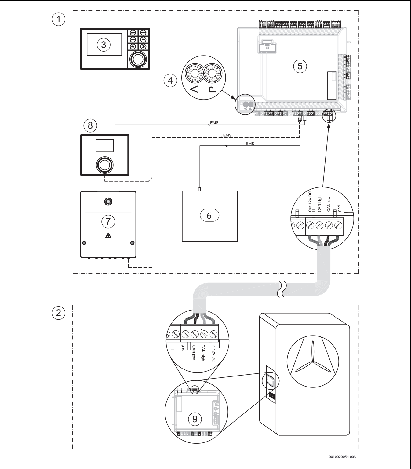
Fig. 33 CAN-BUS/EMS-BUS pour unité intérieure avec chauffage d'appoint électrique – aperçu
