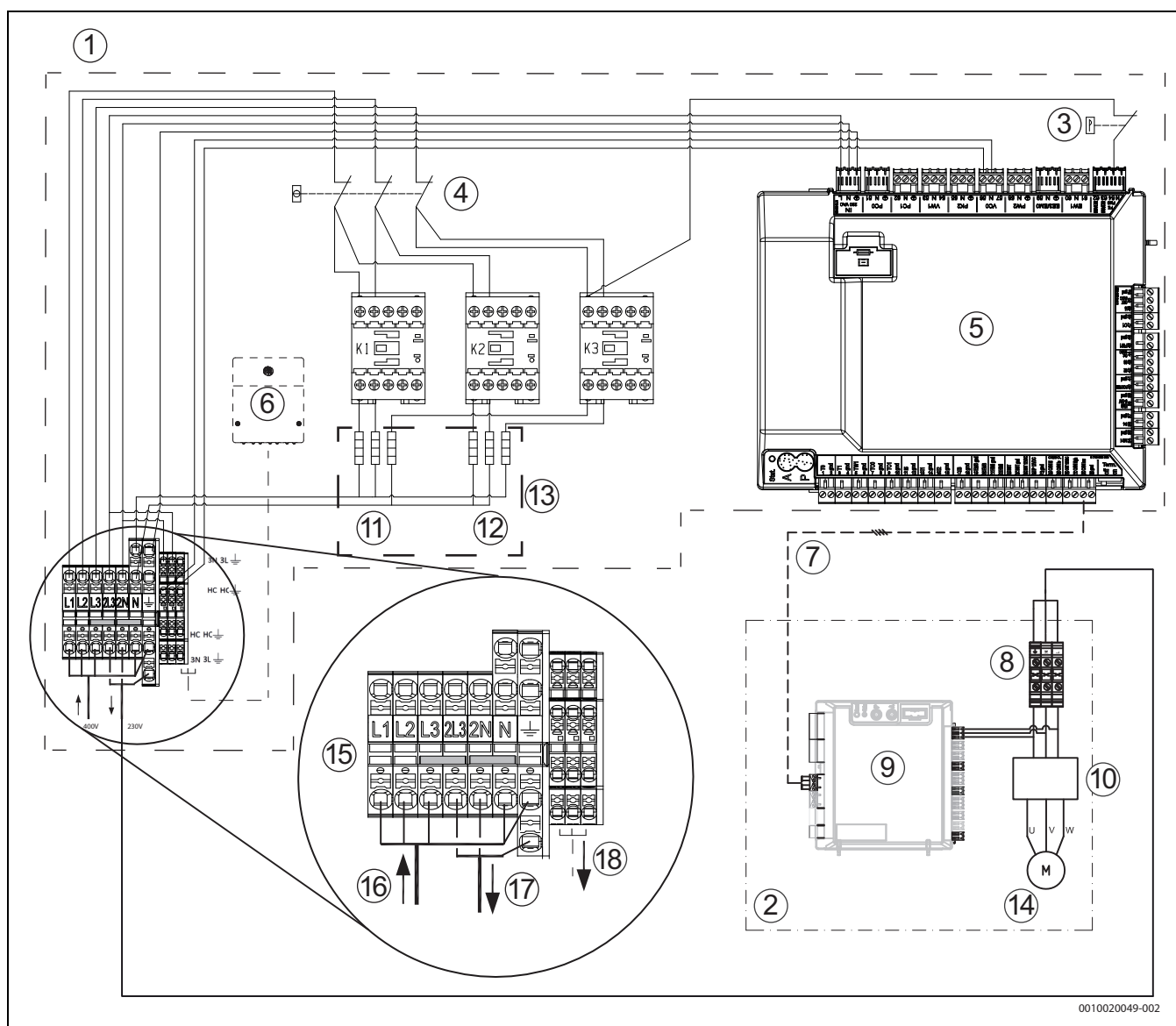
Fig. 34 Pompe à chaleur monophasée avec chauffage d'appoint électrique intégré (courant triphasé)
