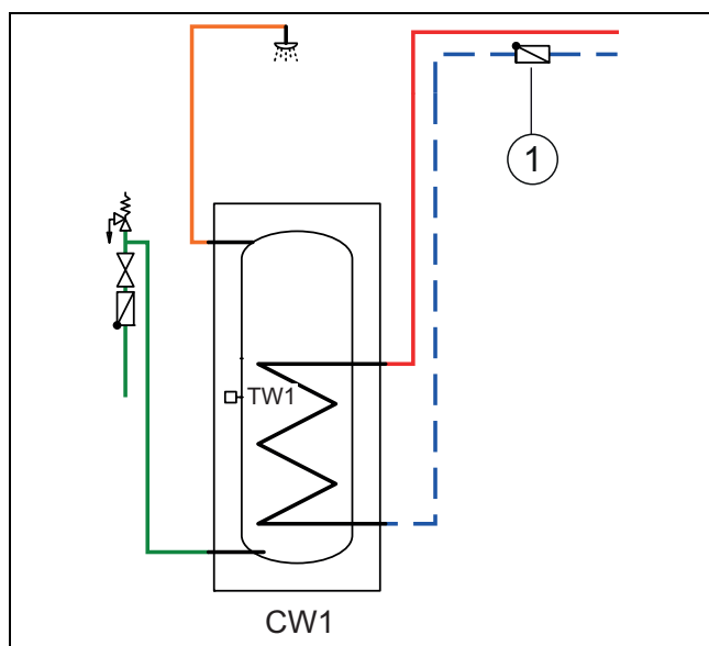
Fig. 23 Ballon d'eau chaude sanitaire
