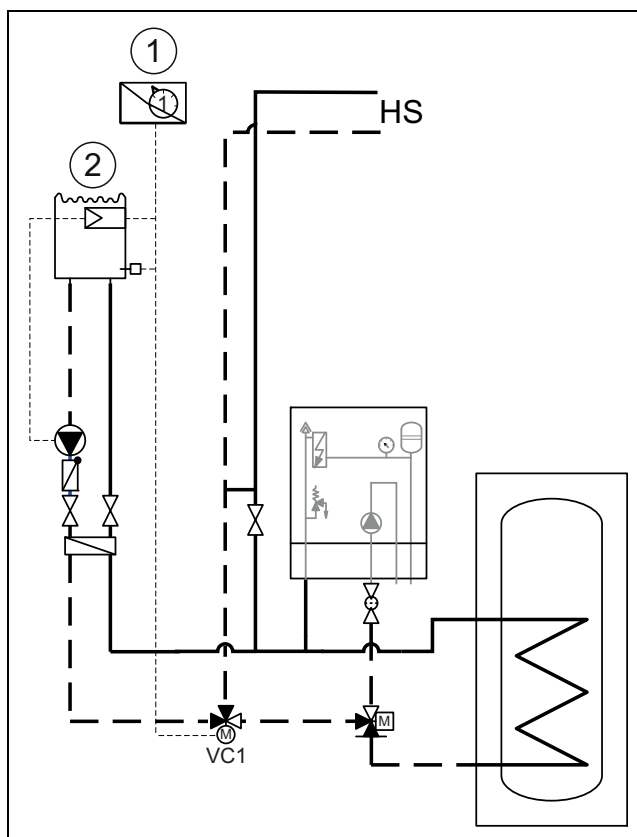
Fig. 28 Exemple d'installation de piscine
