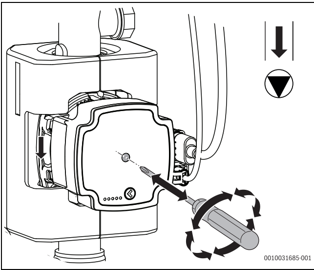
Fig. 33 Débloquer la pompe
