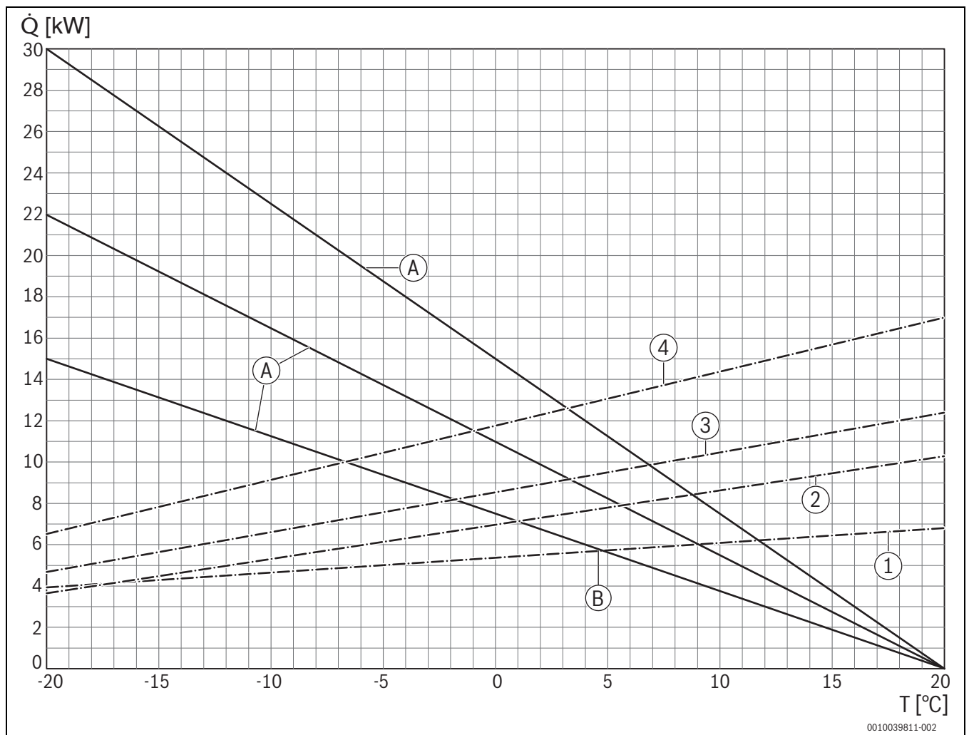
Fig. 29 Diagramme du tableau 7 ; pour déterminer les points de bivalence de la température pour une température de départ de 55 °C
