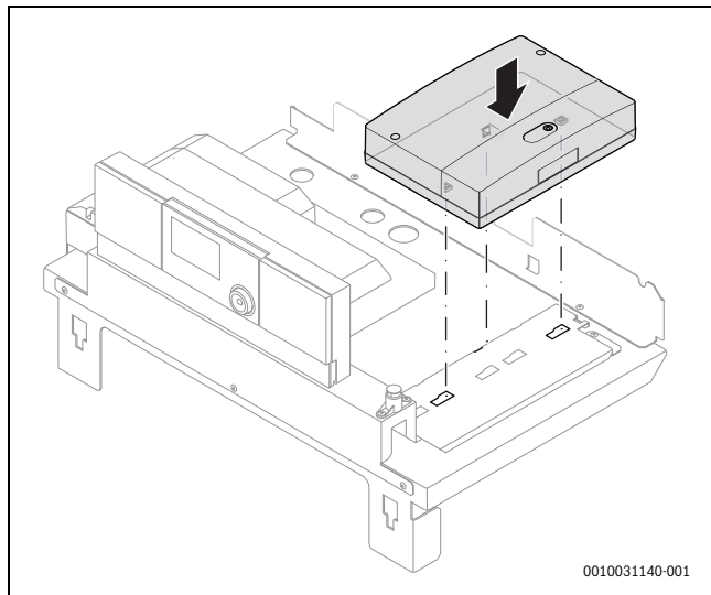
Fig. 17 Montage du module électronique sous le capot de la chaudière (exemple)
