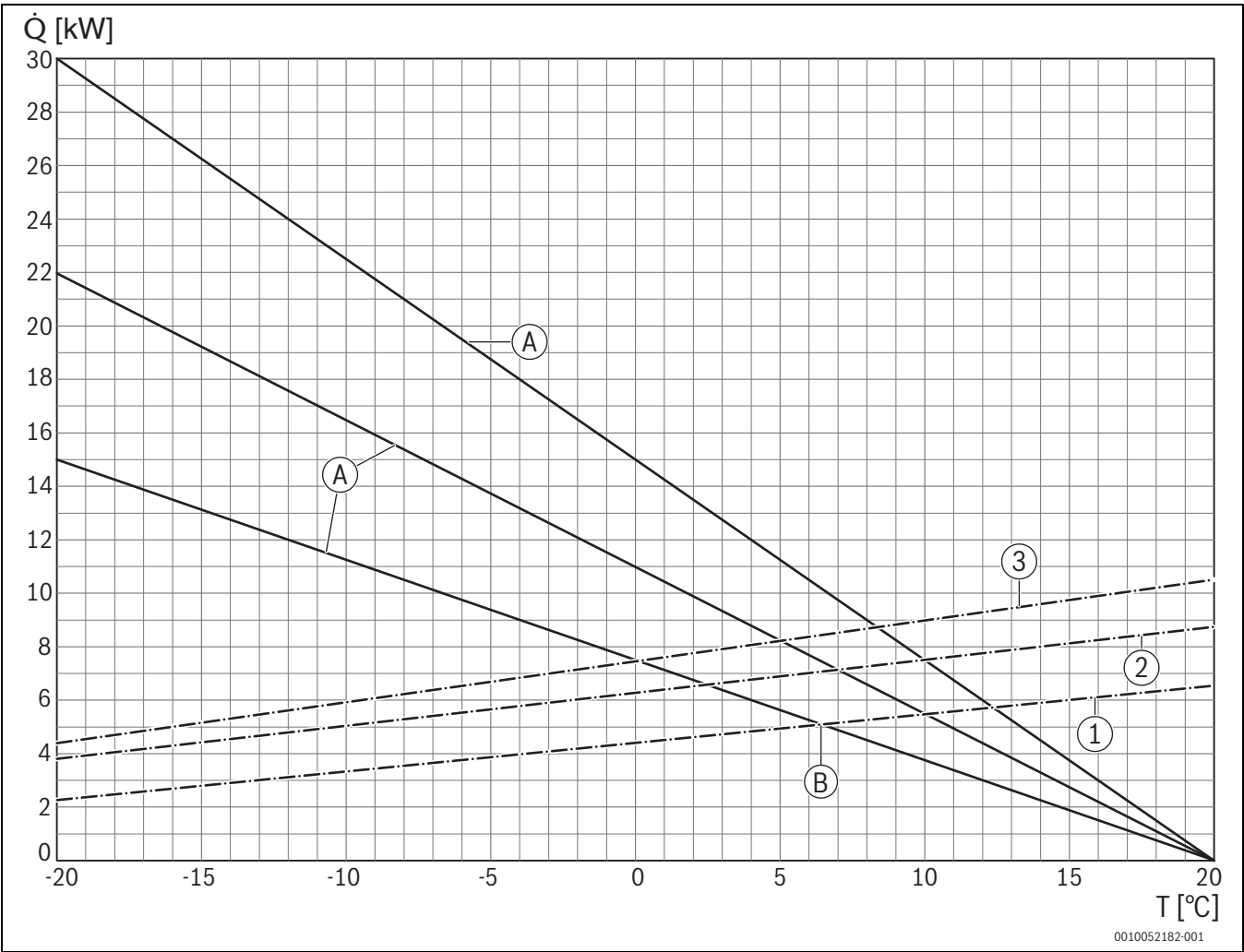
Fig. 28 Diagramme du tableau 6 ; pour déterminer les points de bivalence de la température pour une température de départ de 45 °C
