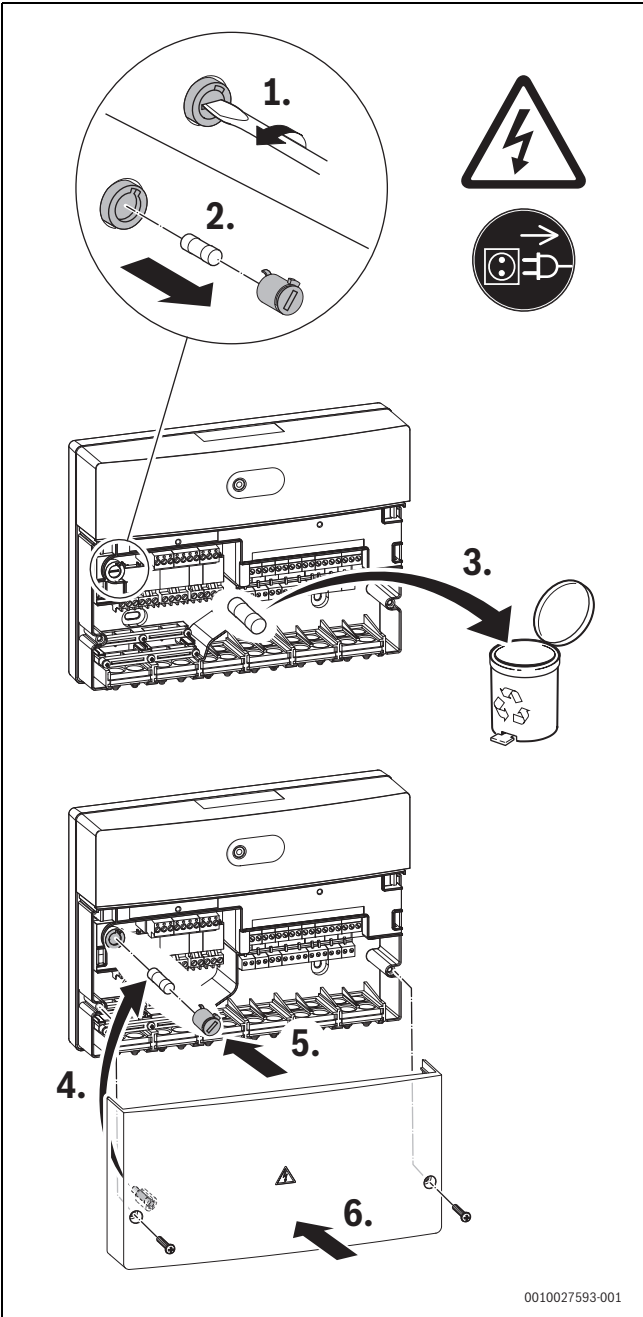
Fig. 35 Remplacer le fusible
