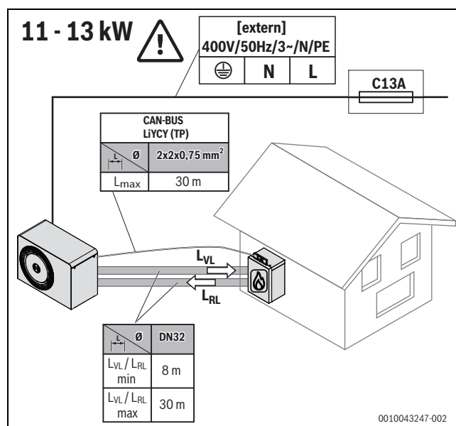
Fig. 9 Exigences relatives à la longueur des conduites 11 – 13 kW
