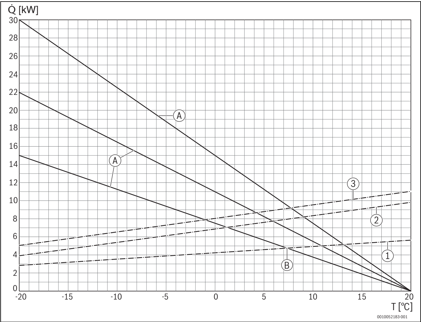
Fig. 26 Diagramme du tableau 4 ; pour déterminer les points de bivalence de la température pour une température de départ de 35 °C
