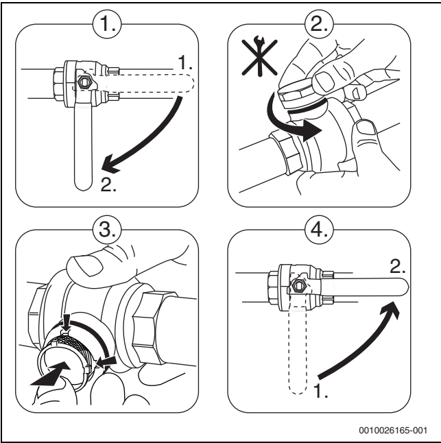
Fig. 32 Montage et démontage du filtre de particules (exemple)
