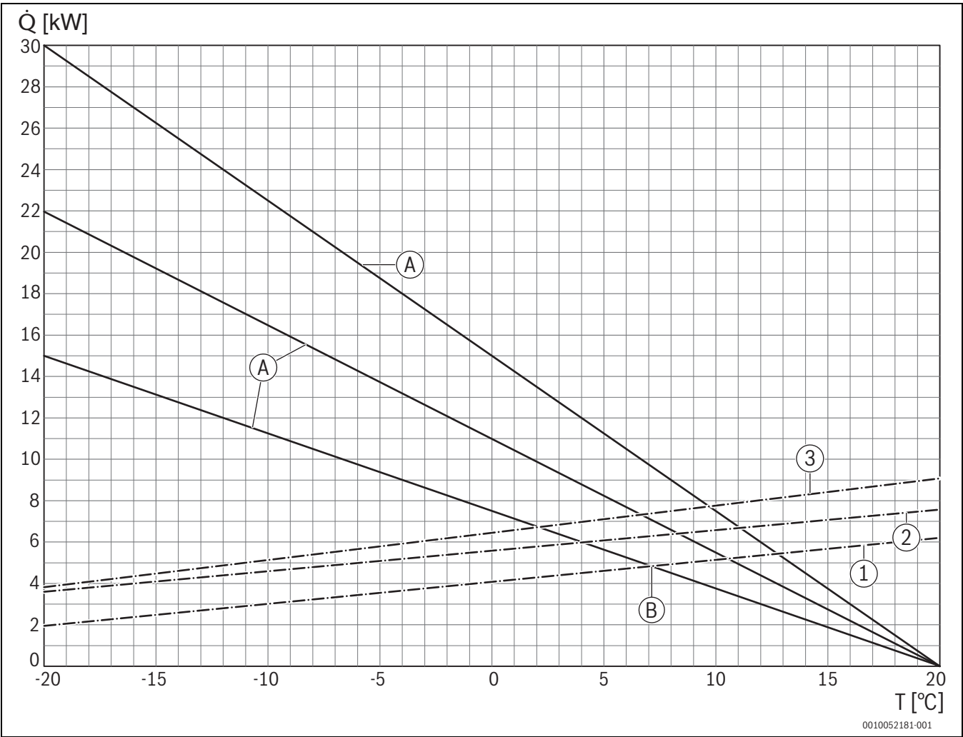
Fig. 30 Diagramme du tableau 8 ; pour déterminer les points de bivalence de la température pour une température de départ de 55 °C
