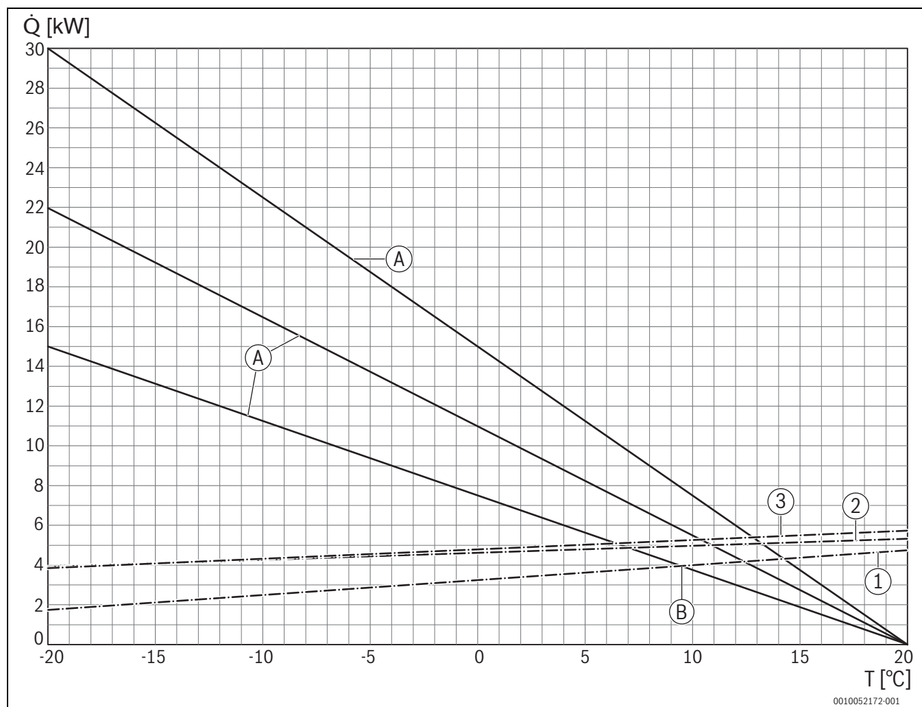
Fig. 31 Diagramme du tableau 9 ; pour déterminer les points de bivalence de la température pour une température de départ de 65 °C
