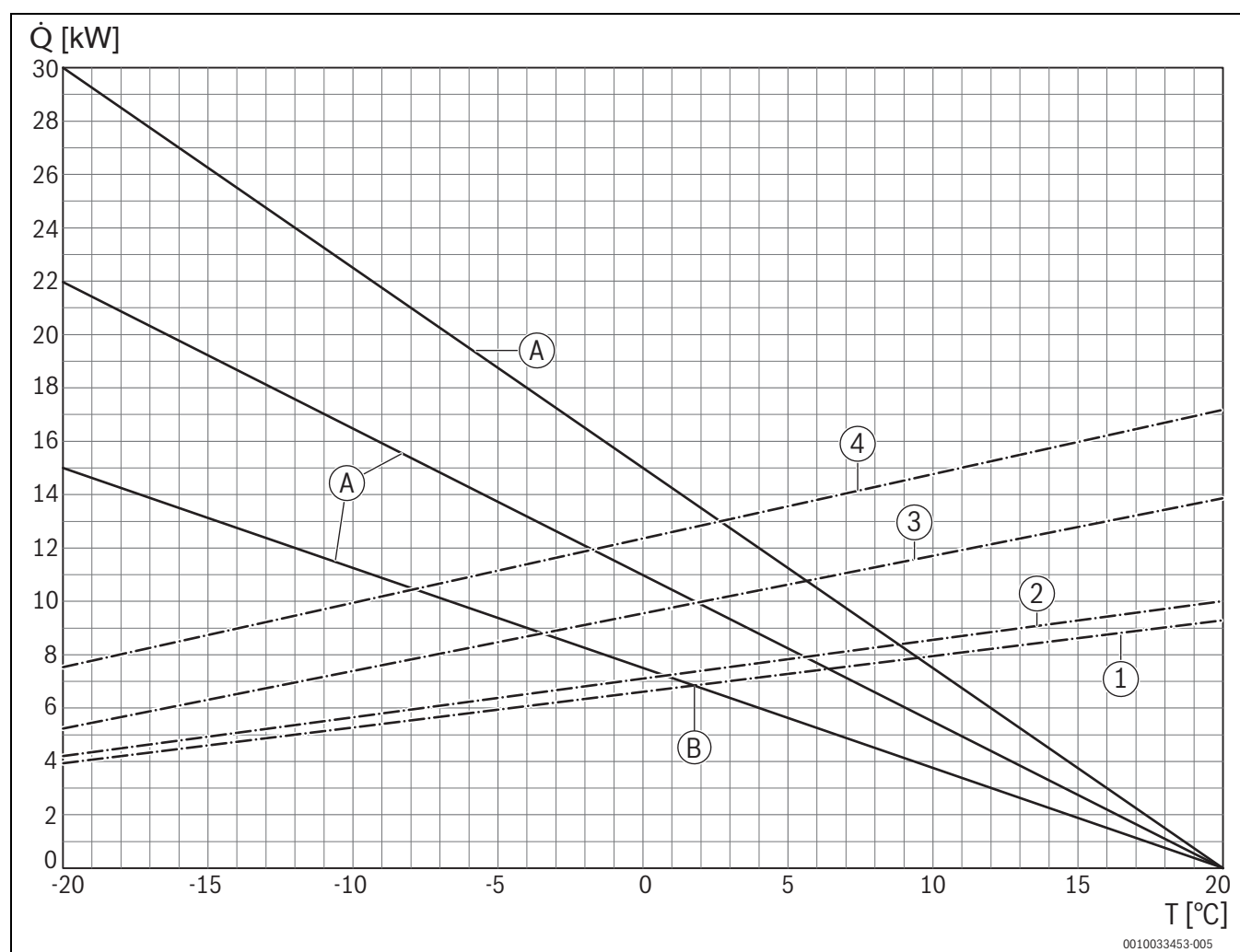
Fig. 25 Diagramme du tableau 3 ; pour déterminer les points de bivalence de la température pour une température de départ de 35 °C
