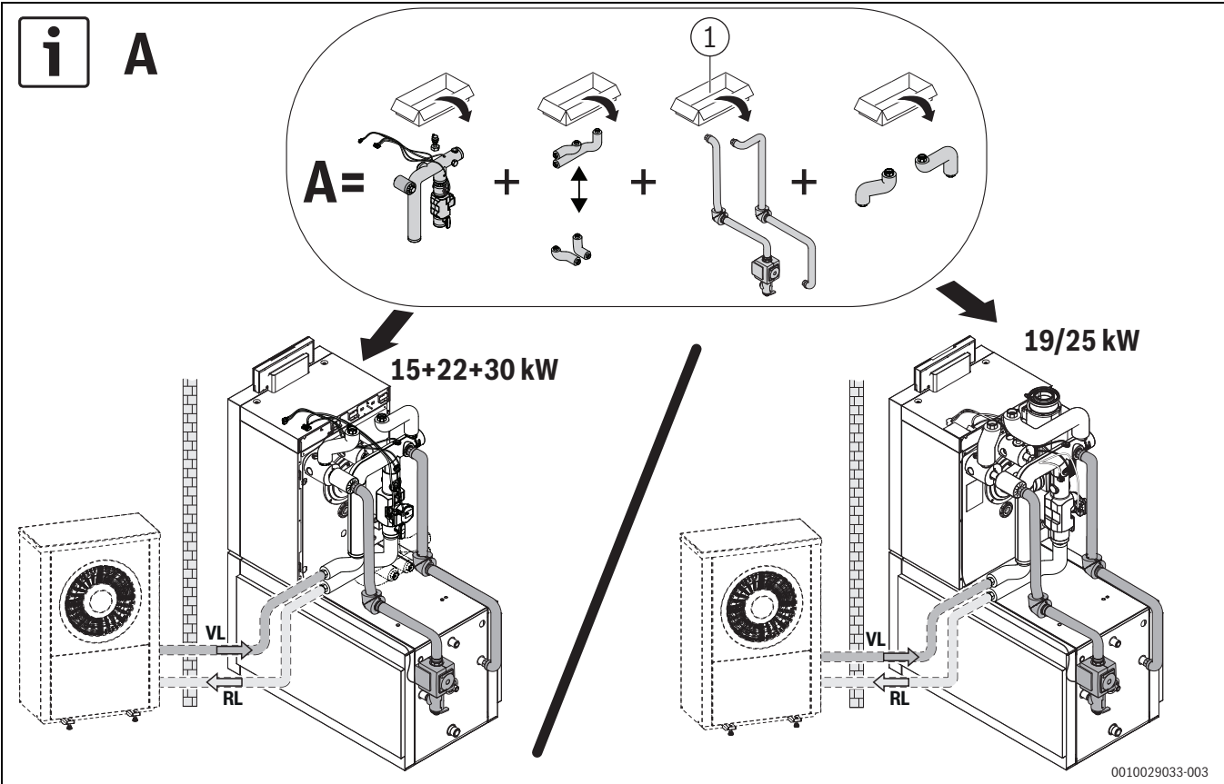
Fig. 10 Connexion ballon du ballon horizontal, variante A
