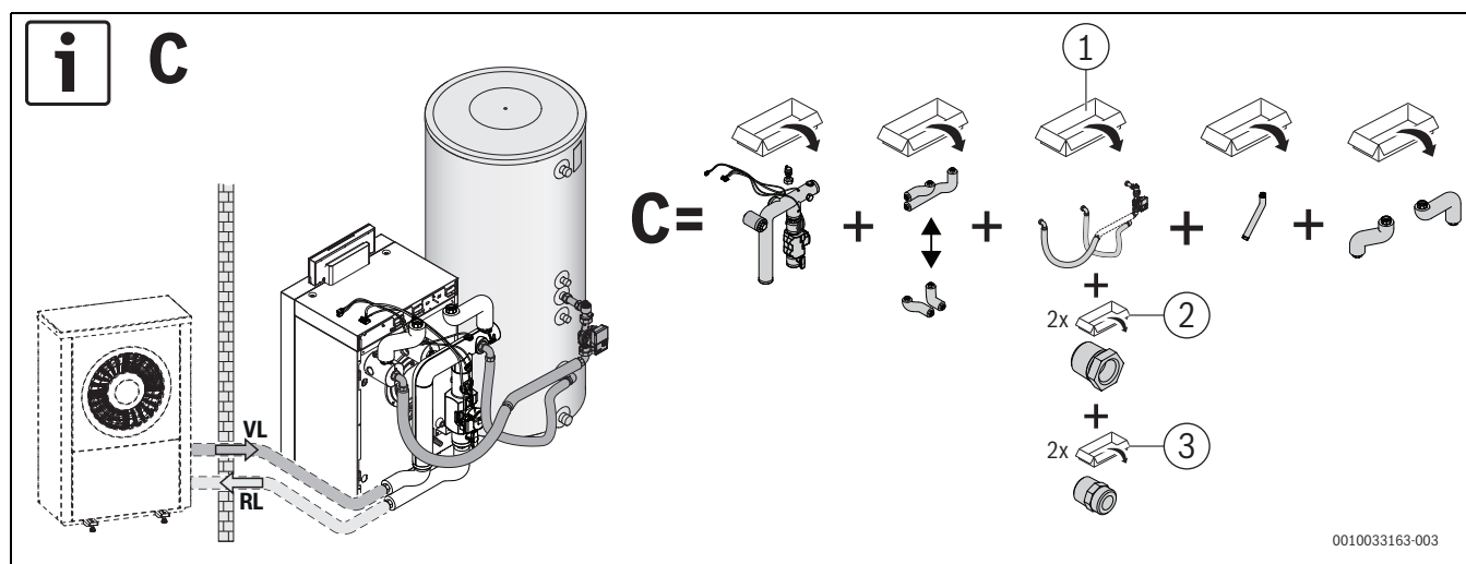
Fig. 14 Connexion ballon ballon vertical à gauche, variante C, exemple d'illustration pour taille de chaudière 15 kW
