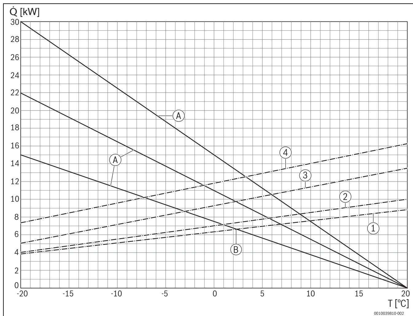
Fig. 27 Diagramme du tableau 5 ; pour déterminer les points de bivalence de la température pour une température de départ de 45 °C
