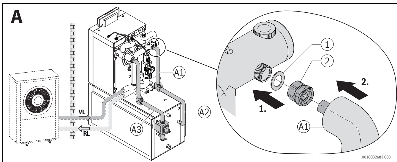
Fig. 12 Montage de la connexion ballon du ballon horizontal, variante A, exemple d'illustration pour taille de chaudière 15 kW
