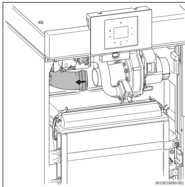
Fig. 39 Retrait du tuyau d'aspiration d'air
