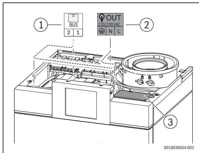
Fig. 30 Monter le module de fonction
