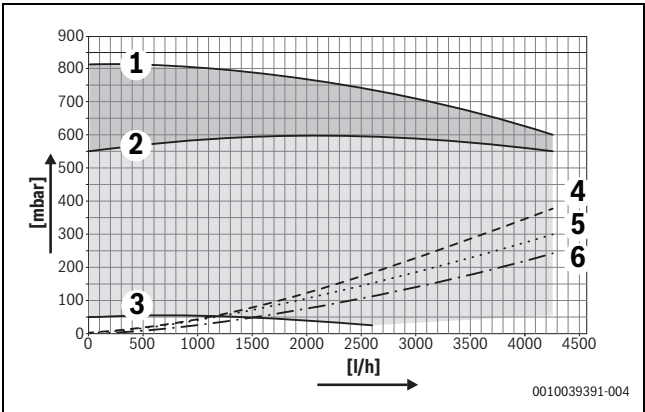
Fig. 53 Hauteur de refoulement résiduelle de la pompe 85kW-100kW
