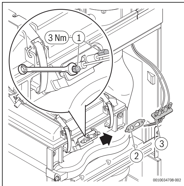
Fig. 48 Remplacement de la cartouche d'allumage
