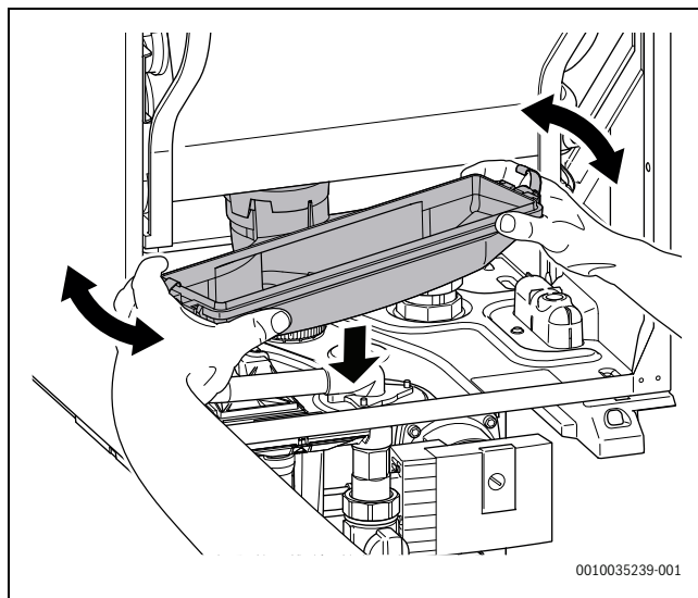
Fig. 47 Retirer le bac à condensats
