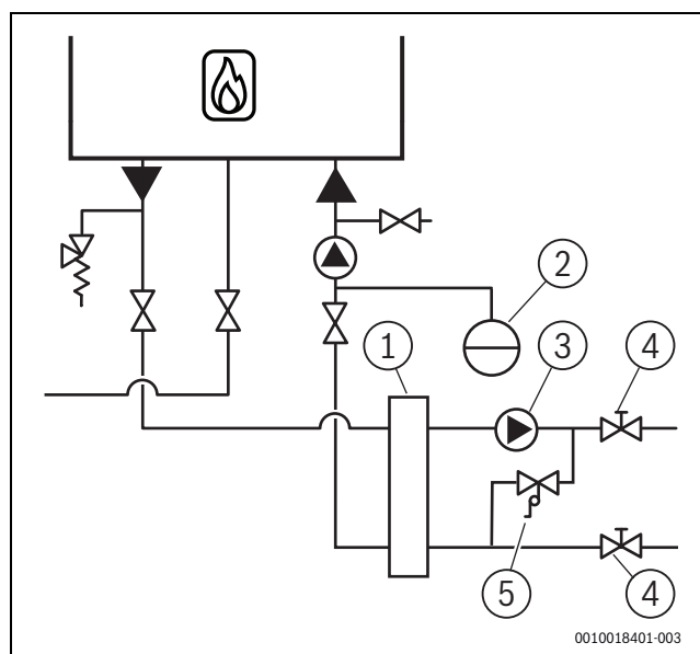
Fig. 19 Mise en place avec bouteille de découplage hydraulique
