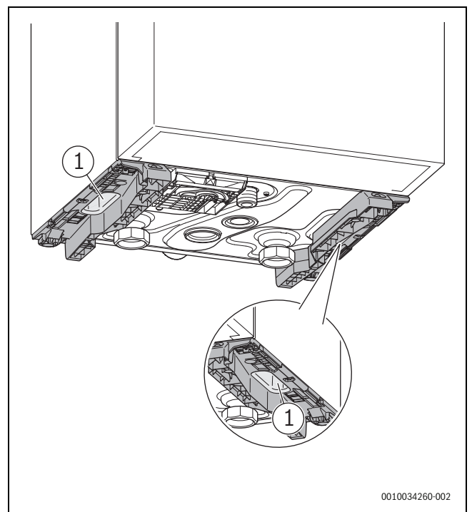
Fig. 7 Position des poignées encastrées
