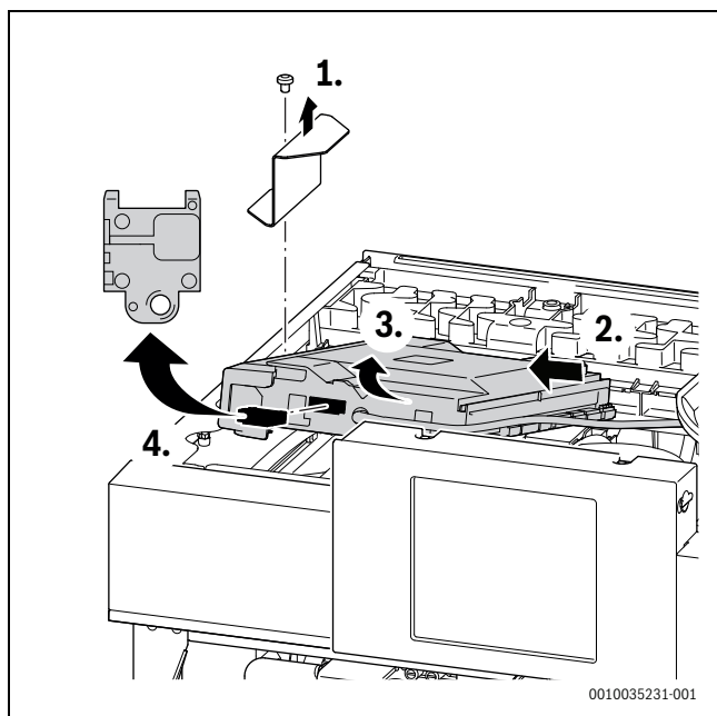
Fig. 50 Remplacer la clé de codage
