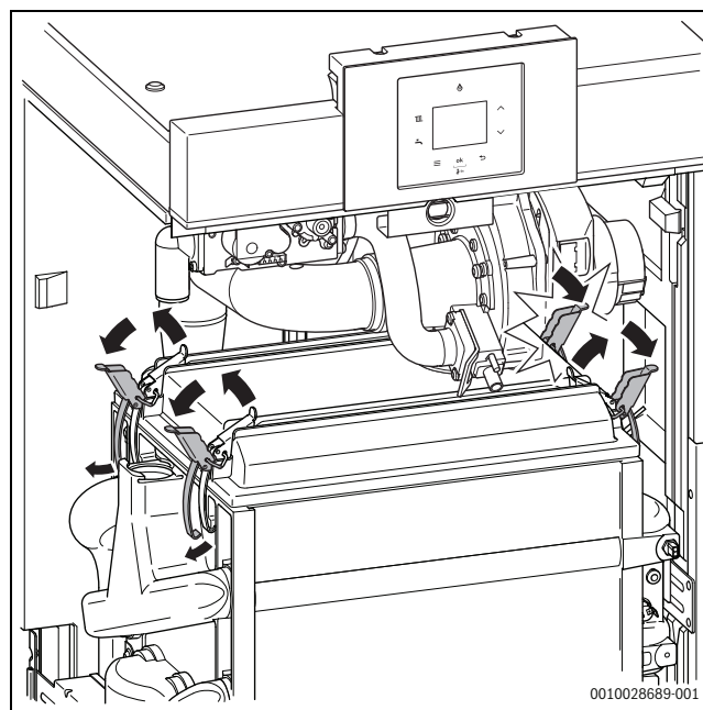
Fig. 40 Ouverture des fermetures à clic
