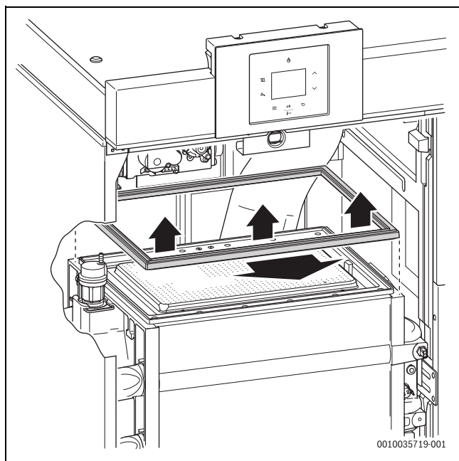
Fig. 42 Retirer le joint du brûleur
