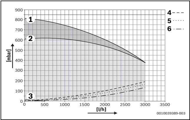
Fig. 52 Hauteur de refoulement résiduelle de la pompe 50kW-85kW
