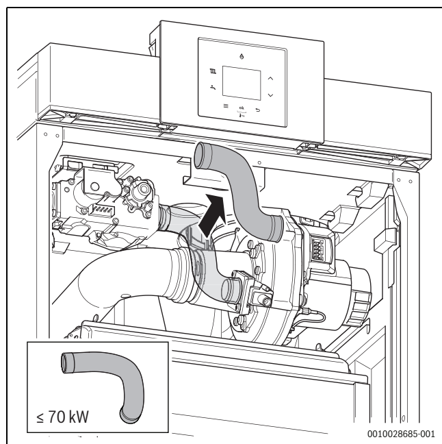
Fig. 38 Retrait du tuyau de gaz \geq 85 kW
