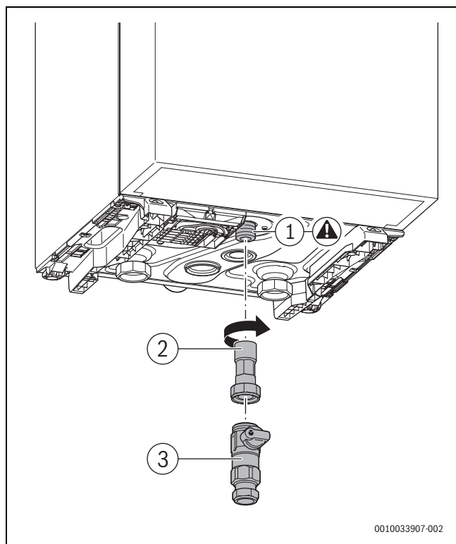
Fig. 13 Installation de la vanne de gaz
