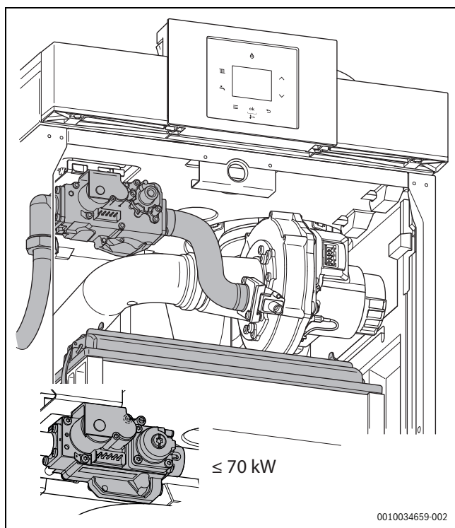
Fig. 36 Contrôle de la trajectoire du gaz
