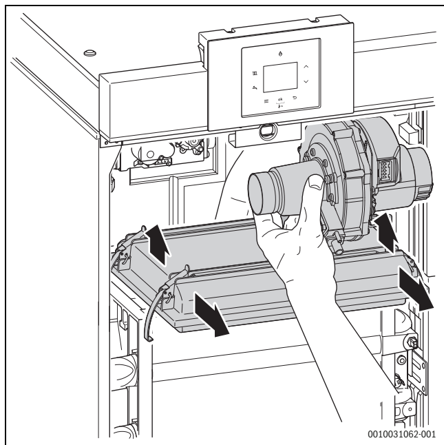
Fig. 41 Retirer l'unité gaz-air avec le capot de brûleur
