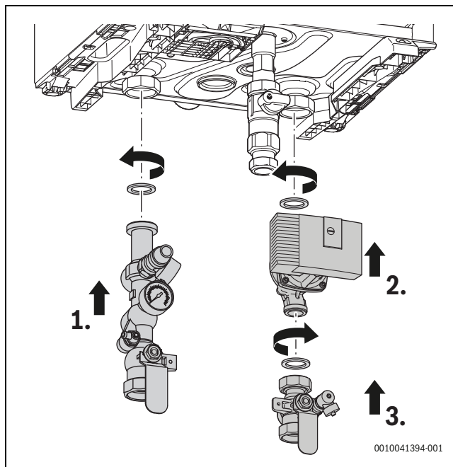
Fig. 14 Installer le raccordement de départ/retour
