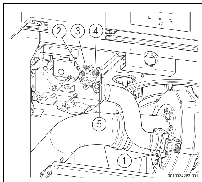
Fig. 33 Vue d'ensemble des tubulures de mesure et des vis de réglage ≥ 85 kW
