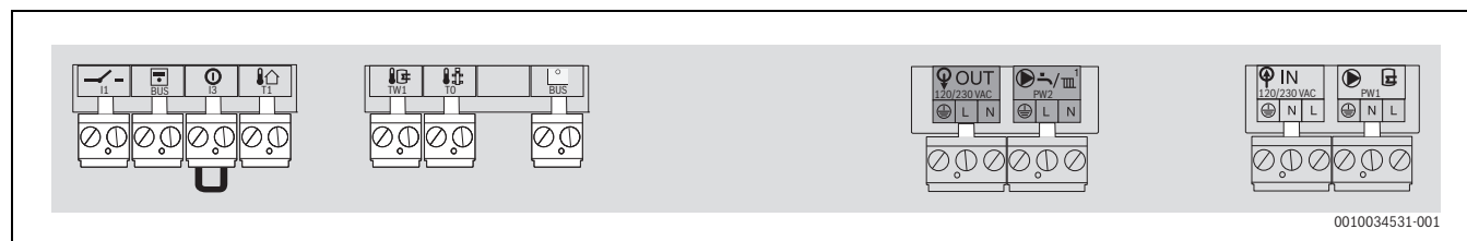
Fig. 23 Aperçu de la barrette de raccordement
