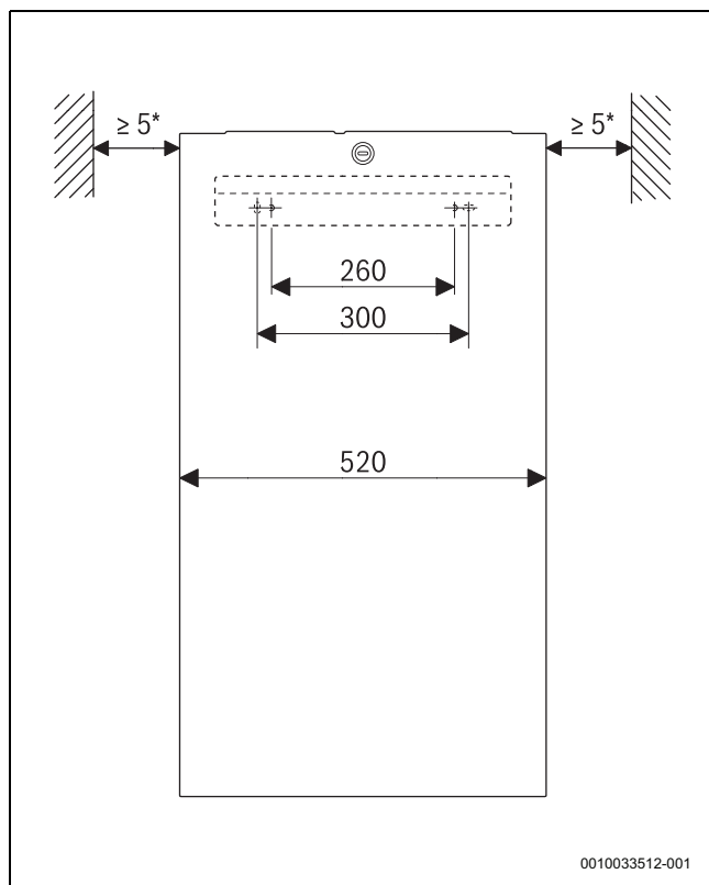
Fig. 5 Vue de face [mm]
