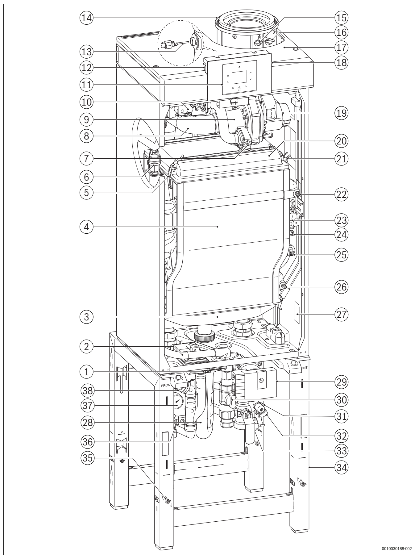
Fig. 1 GB272 avec kit de raccordement sur le cadre-support
