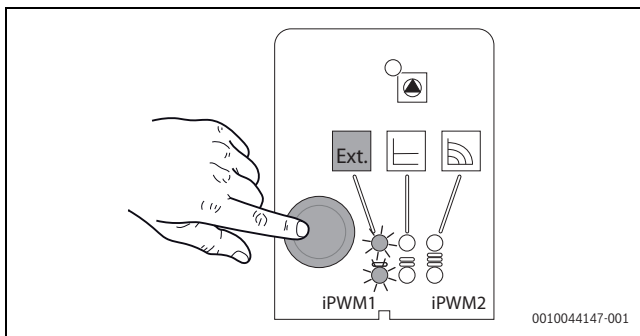
Fig. 27 Régler la pompe de chaudière sur \leq 70 kW
