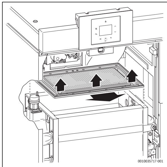
Fig. 43 Retirer le brûleur
