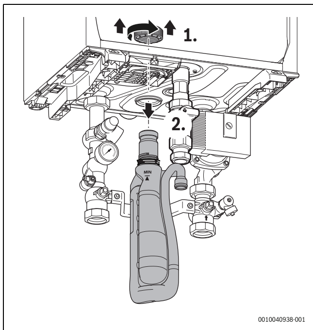
Fig. 45 Retirer le siphon de la chaudière
