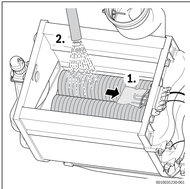
Fig. 44 Nettoyage de l'échangeur thermique
