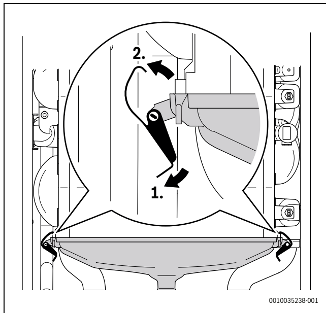
Fig. 46 Ouverture des fermetures à clic du bac à condensats
