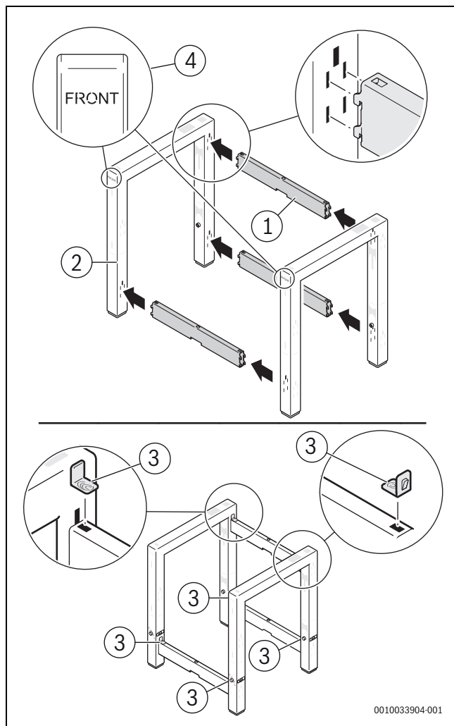
Fig. 8 Installation du cadre-support
