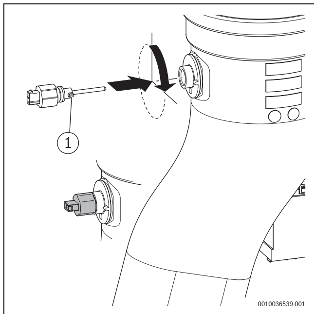
Fig. 49 Remplacer la sonde de température des gaz brûlés
