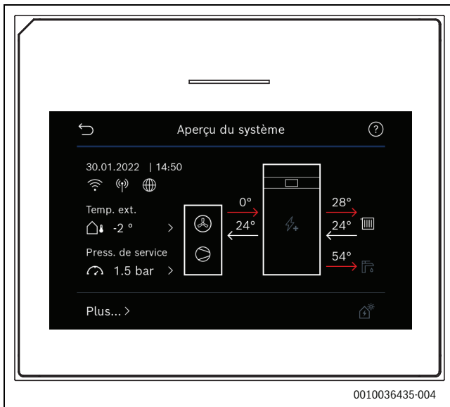
Fig. 11 Aperçu système de la pompe à chaleur
