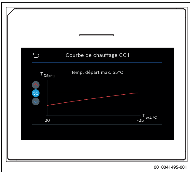
Fig. 5 Régler la température maximale de départ
