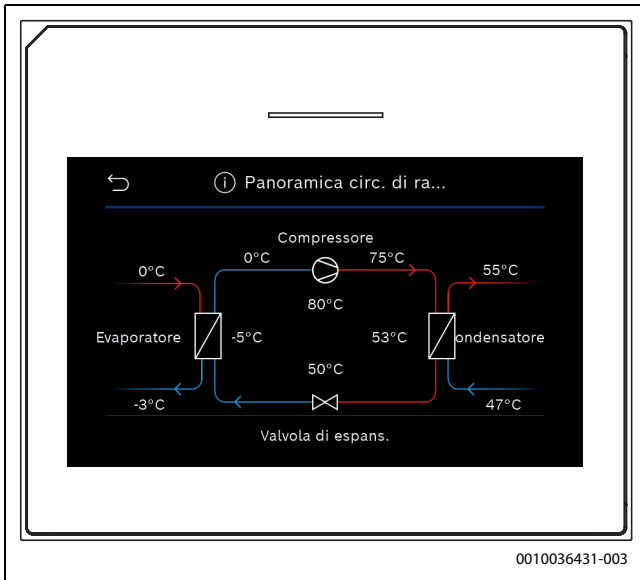
Fig. 10 Panoramica del circuito di raffreddamento
