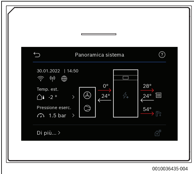
Fig. 11 Panoramica del sistema della pompa di calore
