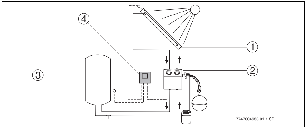
Bild 2 Anlagenschema
